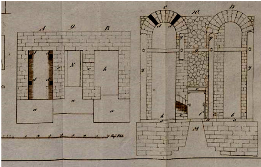
Abbildung Eiserfeyer Kalkofen unter „Benutzung der Hochofen-Gichtflamme zum Betrieb eines Kalkofens“ aus Archiv für Bergbau und Hüttenwesen
