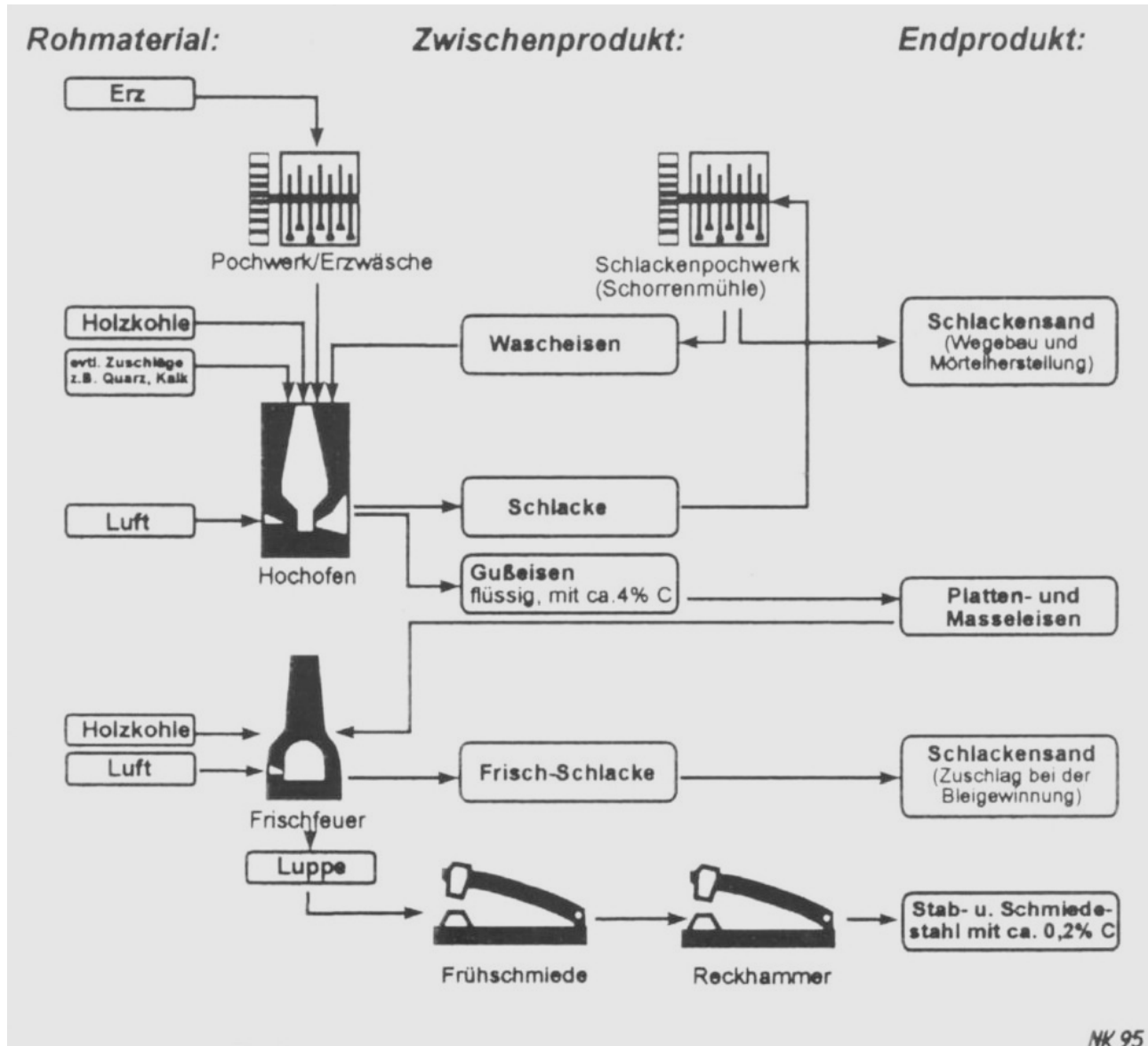
Verhüttungsschema Eifeler Reidtwerke: Vom Eisenerz zum Stahl Grafik aus der Festschrift „100 Jahre Eifelverein Ortsgruppe Kall“
