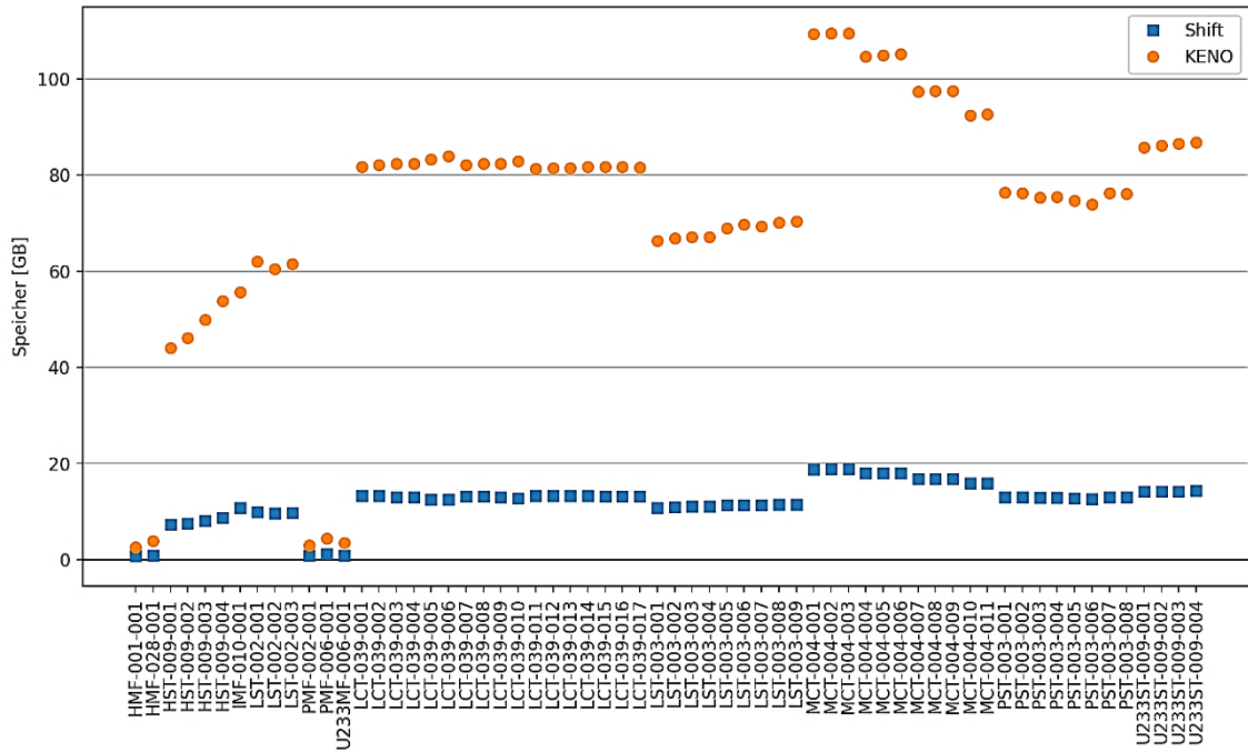
Abb. 3.10 Arbeitsspeicherbedarf der TSUNAMI-Shift - und TSUNAMI-KENO-V.a -Rechnungen
