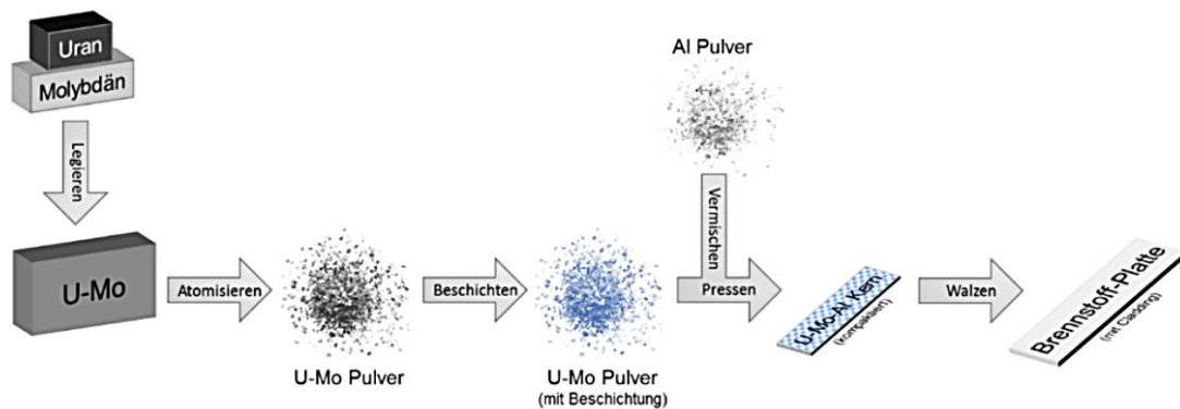
Abb. 4.23 Schematische Übersicht zum Fertigungsprozess eines dispersen U-Mo-Brennstoffes
