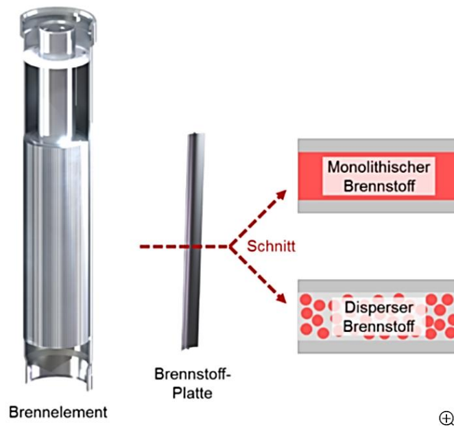
Abb. 4.22 Typisches Brennelement des FRM-II, mit einzelnen, zu Evolventen gebogenen Brennstoffplatten die mittels dazwischen ausgeprägten Kühlschlitzen, zirkular zu einem Brennelement angeordnet werden.
