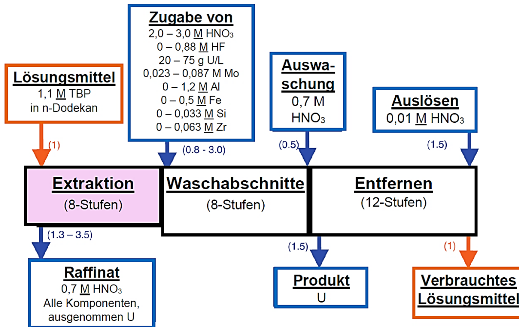
Abb. 4.25 Fließschema mit Konzentrationsangaben der einzusetzenden Chemikalien für die Uranrückgewinnung aus aufgelösten U-Mo-Herstellungsfragmenten
