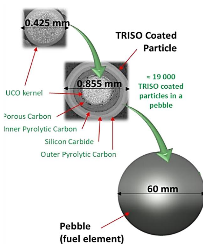
Abb. 4.6 Prinzipieller Aufbau einer Brennstoffkugel der Xe-100 Design Solution der Firma X-Energy
