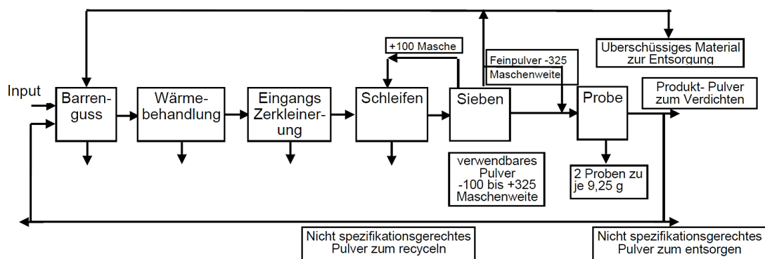
Abb. 4.18 Schematische Darstellung des Ablaufs des Pulverproduktionsprozesses
