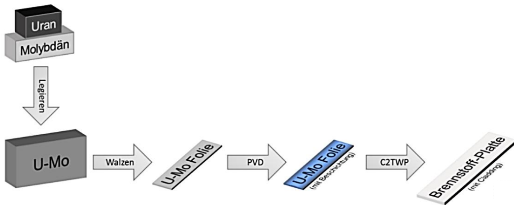
Abb. 4.24 Schematische Übersicht zum Fertigungsprozess eines monolithischen U-Mo-Brennstoffes
