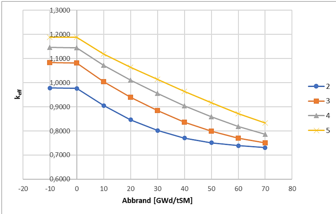
Abb. 3.19 k_{\text{eff}} Werte der Kritikalitätsrechnungen zum Lagerbehälter
