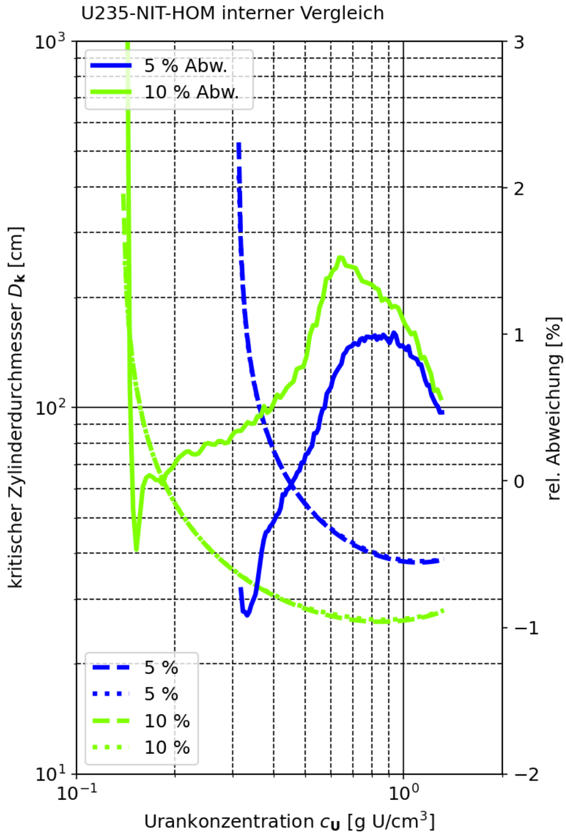
Abb. 2.4 Kritischer Zylinderdurchmesser von Uranylinitrat-Wasser-Systemen. Vergleich der Rechnungen mit klassischer Volumenaddition und unter Verwendung der Dichteformel nach CRISTAL V2
