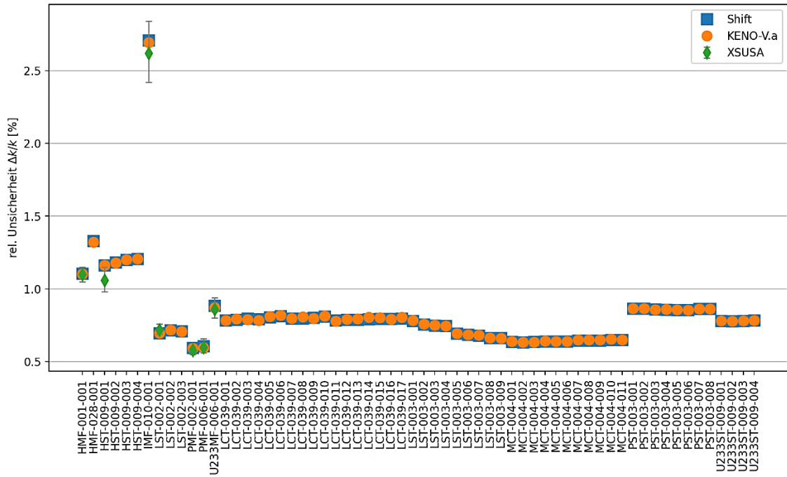
Abb. 3.8 Relative Unsicherheiten des Multiplikationsfaktors aufgrund von Unsicherheiten in den nuklearen Daten
