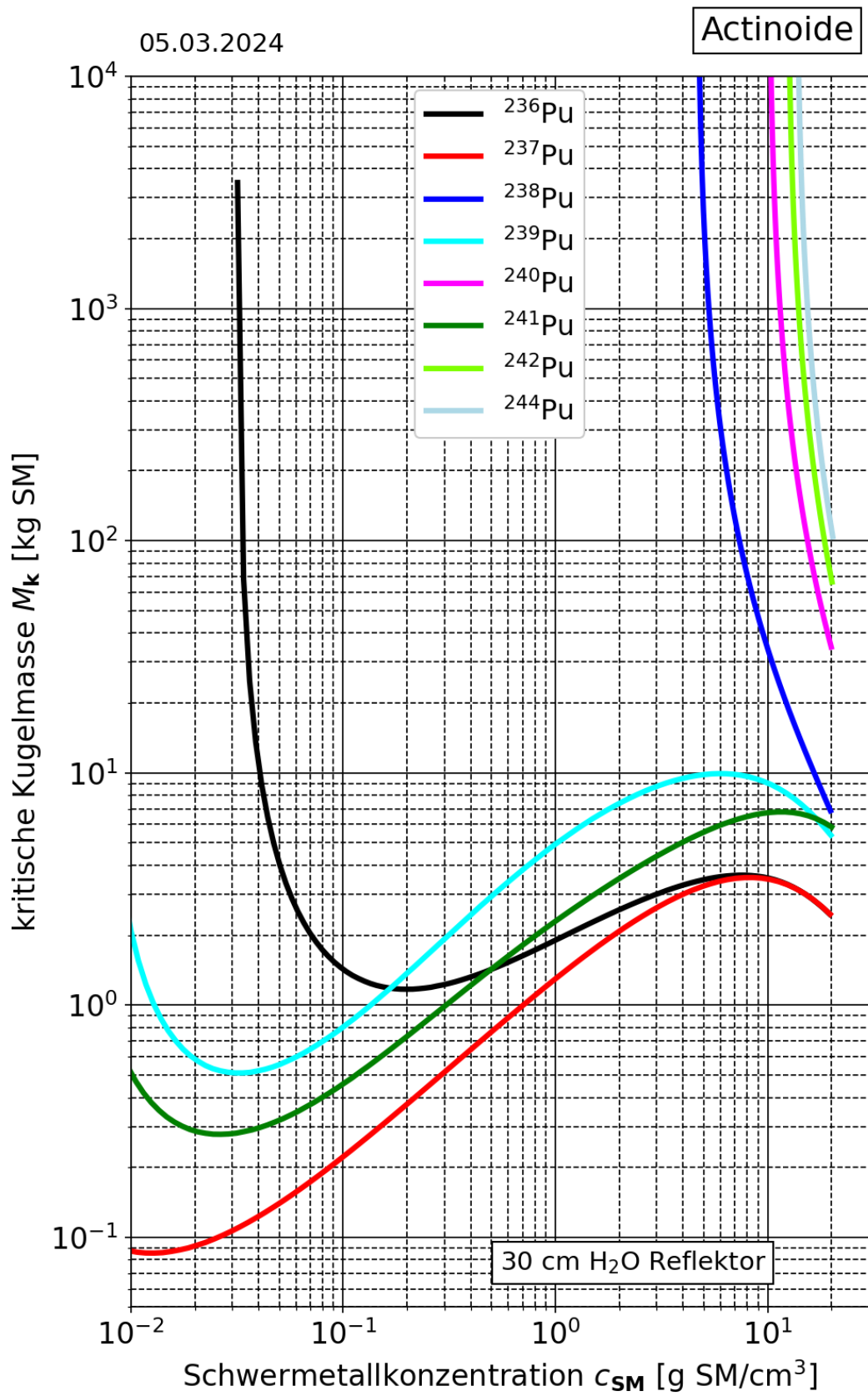
Abb. 2.11 Kritische Kugelmasse M_k für alle gerechneten Plutonium Isotope mit H 2 O Reflektor
