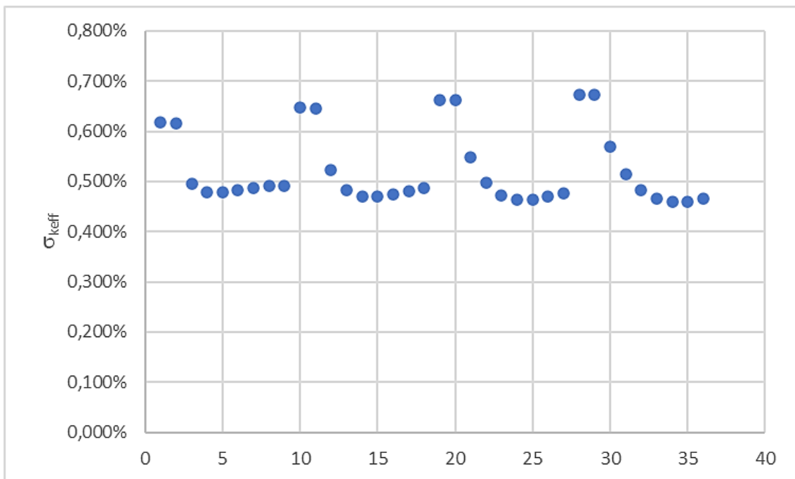
Abb. 3.20 \sigma_{k_{\text{eff}}} der Kritikalitätsrechnungen zum Lagerbehälter
