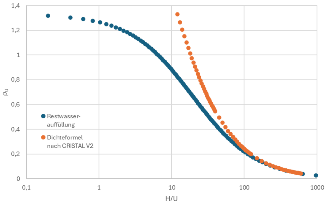
Abb. 2.1 Urandichte \rho_U in Abhängigkeit des Moderationsverhältnisses H/U Uranyl-nitrat
