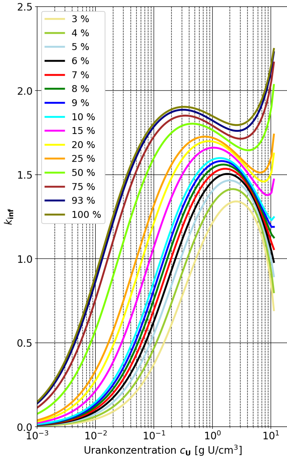
Abb. 2.18 Infiniter Multiplikationsfaktor k_{inf} für homogene Uransilizid-Wasser-Gemische
