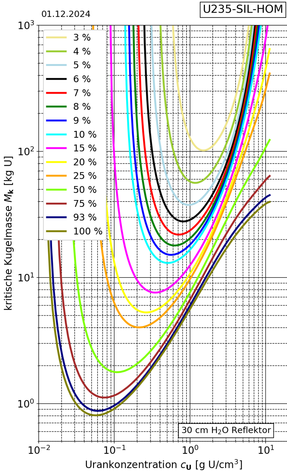
Abb. 2.19 Kritische Kugelmasse für homogene Uransilizid-Wasser-Gemische
