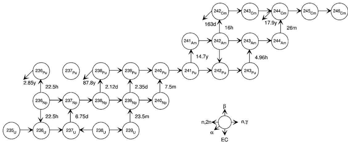
Abb. 4.5 Actinoiden-Transmutationskette, basierend auf der Bateman-Gleichung
