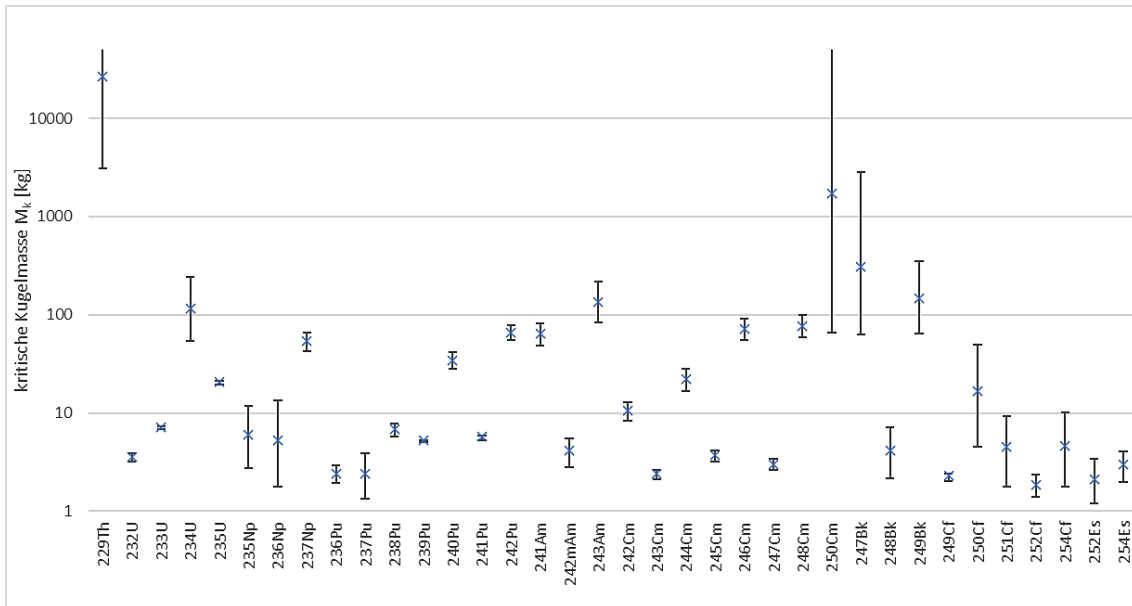
Abb. 2.17 Kritische Kugelmasse M_k [kg] der metallischen Systeme mit abgeschätzten Unsicherheiten aufgrund von Unsicherheiten der nuklearen Daten
