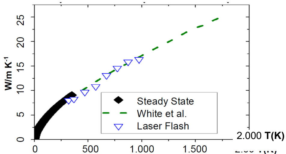
Abb. 4.12 Verlauf der Wärmeleitfähigkeit \text{U}_3\text{Si}_2 über der Temperatur in Kelvin T(K), basierend auf Steady State, Laser Flash sowie rechnerischen Daten /INL 18/
