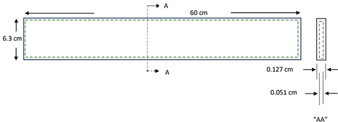
Abb. 4.20 Typische Schnittbilder einer assemblierten Brennstoffplatte
