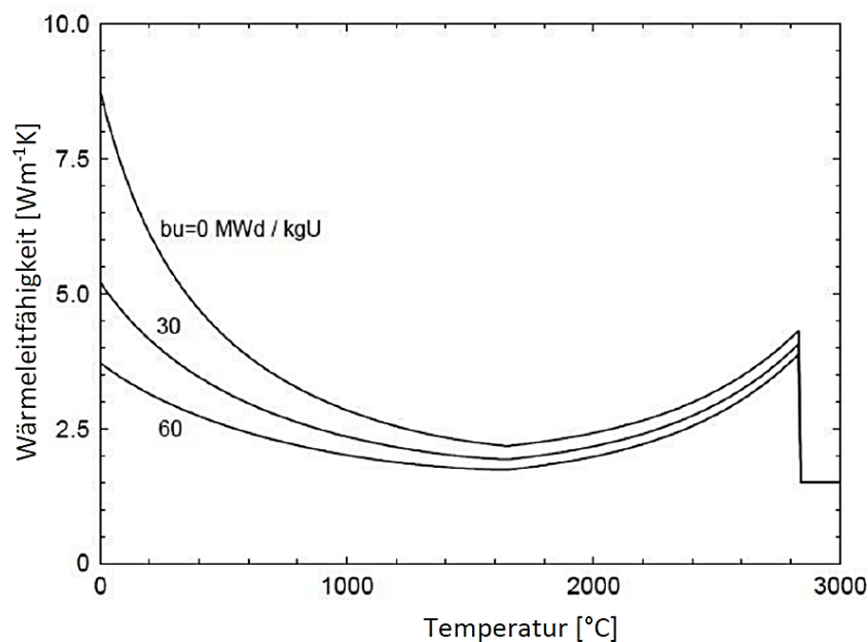
Abb. 4.11 Wärmeleitfähigkeit von UO_2 in ^\circ\text{C}
