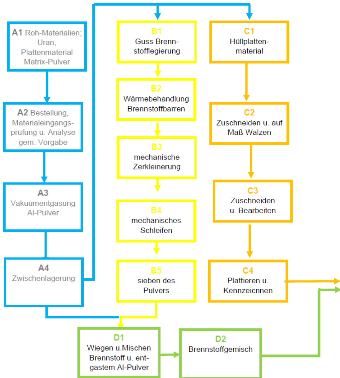
Abb. 4.16 Darstellung von Prozessschritt 1 bis 4 bei der U_3Si_2-Al Produktion
