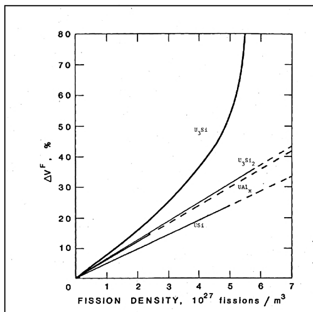
Abb. 4.15 Quellung von USi , U_3Si , U_3Si_2 und UAl_x -Brennstoffpartikeln als Funktion der Spaltungen. Gestrichelte Verläufe zeigen Bereiche, die mit LEU-Brennstoffen nicht erreichbar sind
