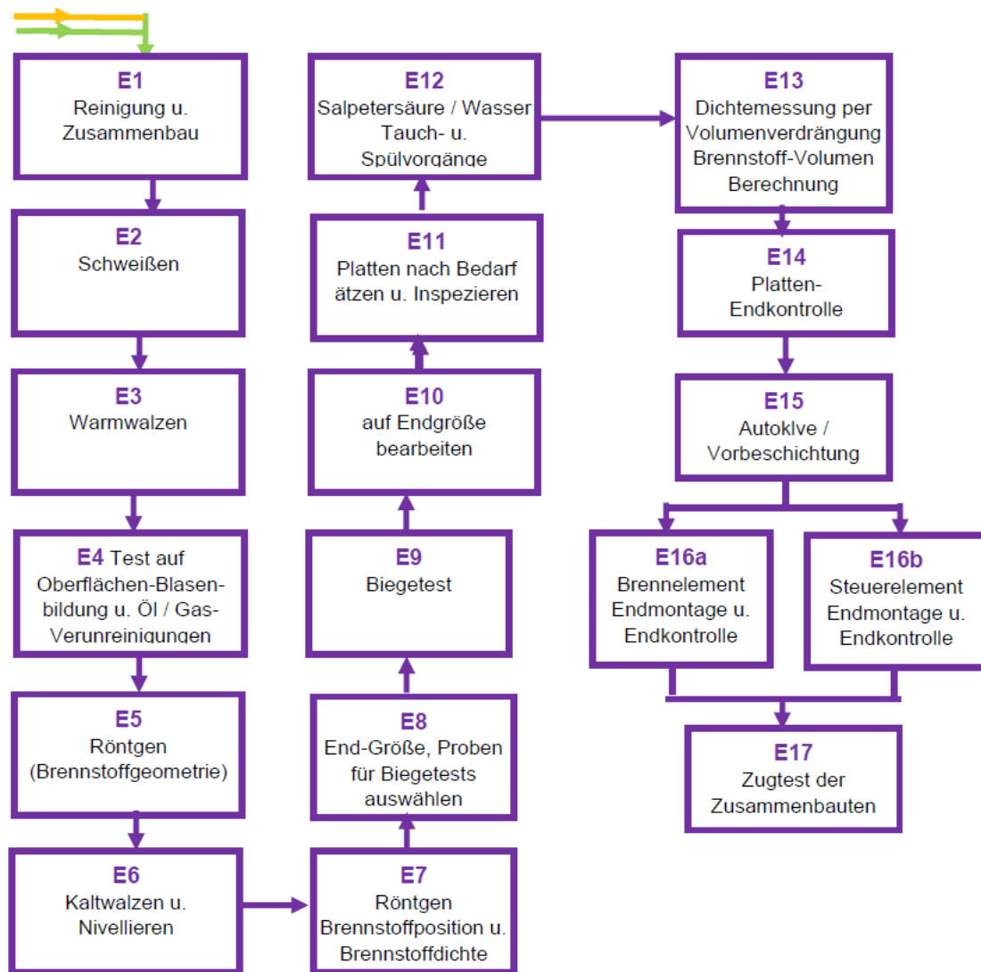
Abb. 4.17 Prozessschritt 5 bei der Herstellung von U_3Si_2 -Al-Dispersionsbrennstoff
