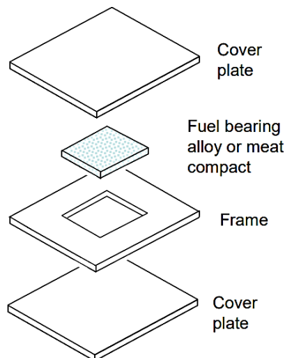
Abb. 4.19 Aufbau der Brennstoffplattenbaugruppe
