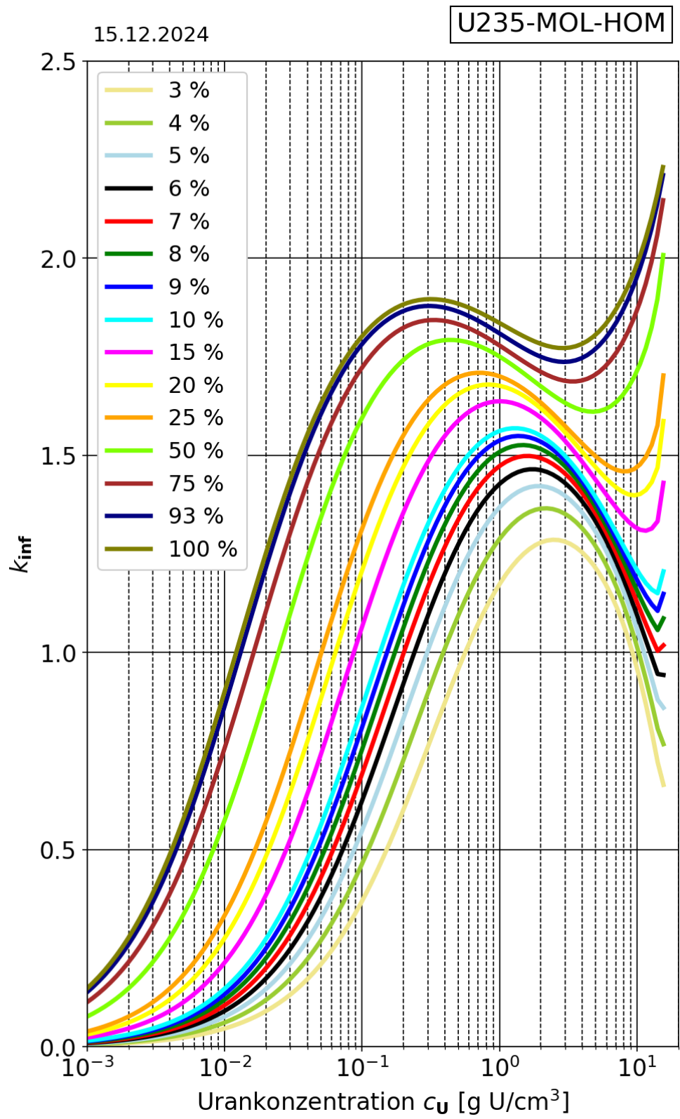
Abb. 2.25 Infiniter Multiplikationsfaktor k_{inf} für homogene Uran-Molybdän-Wasser-Systeme
