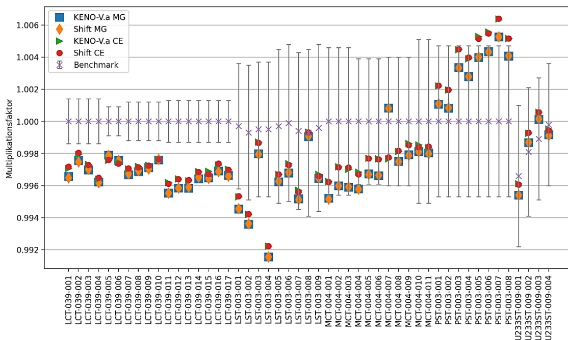
Abb. 3.3 Berechnete Multiplikationsfaktoren im Vergleich zu den gemessenen Benchmark-Ergebnissen
