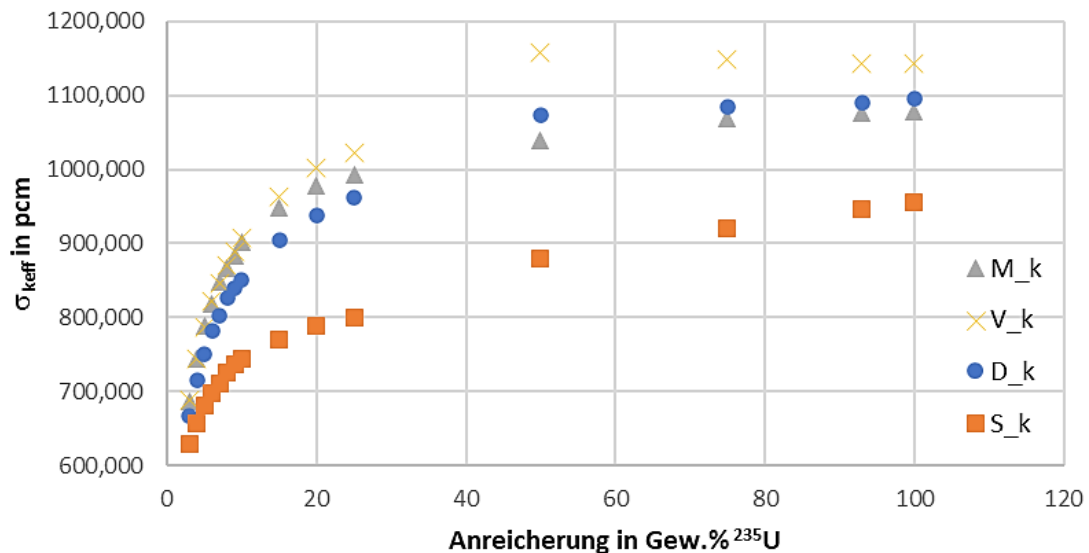
Abb. 2.28 Unsicherheit von k_{\text{eff}} für die Kurvenminima der vier kritischen Parameter ( M_k , V_k , D_k und S_k ) aufgrund von Unsicherheiten in den nuklearen Daten von Uran-Molybdän
