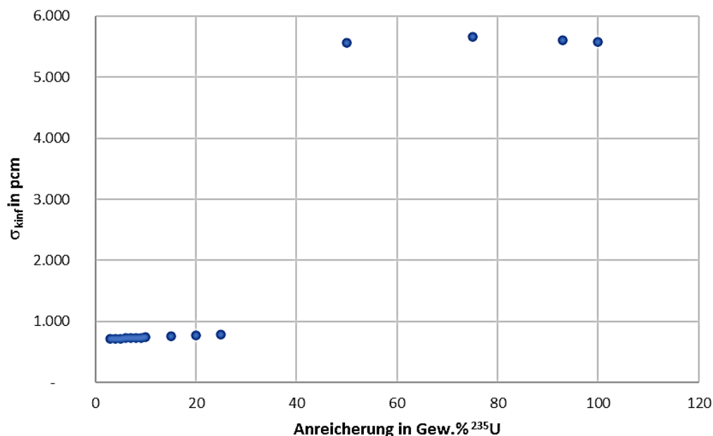
Abb. 2.27 Unsicherheit von k_{inf} für die Kurvenmaxima von Uran-Molybdän aufgrund von Unsicherheiten in den nuklearen Daten
