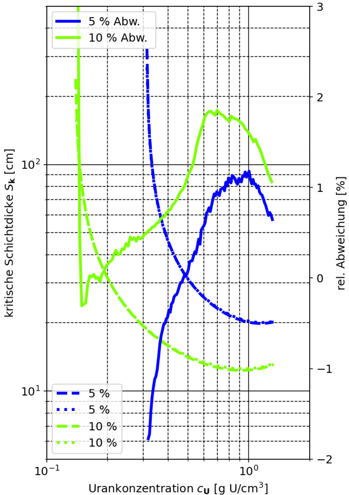
Abb. 2.5 Kritische Schichtdicke von Uranylнитrat-Wasser-Systemen. Vergleich der Rechnungen mit klassischer Volumenaddition und unter Verwendung der Dichteformel nach CRISTAL V2
