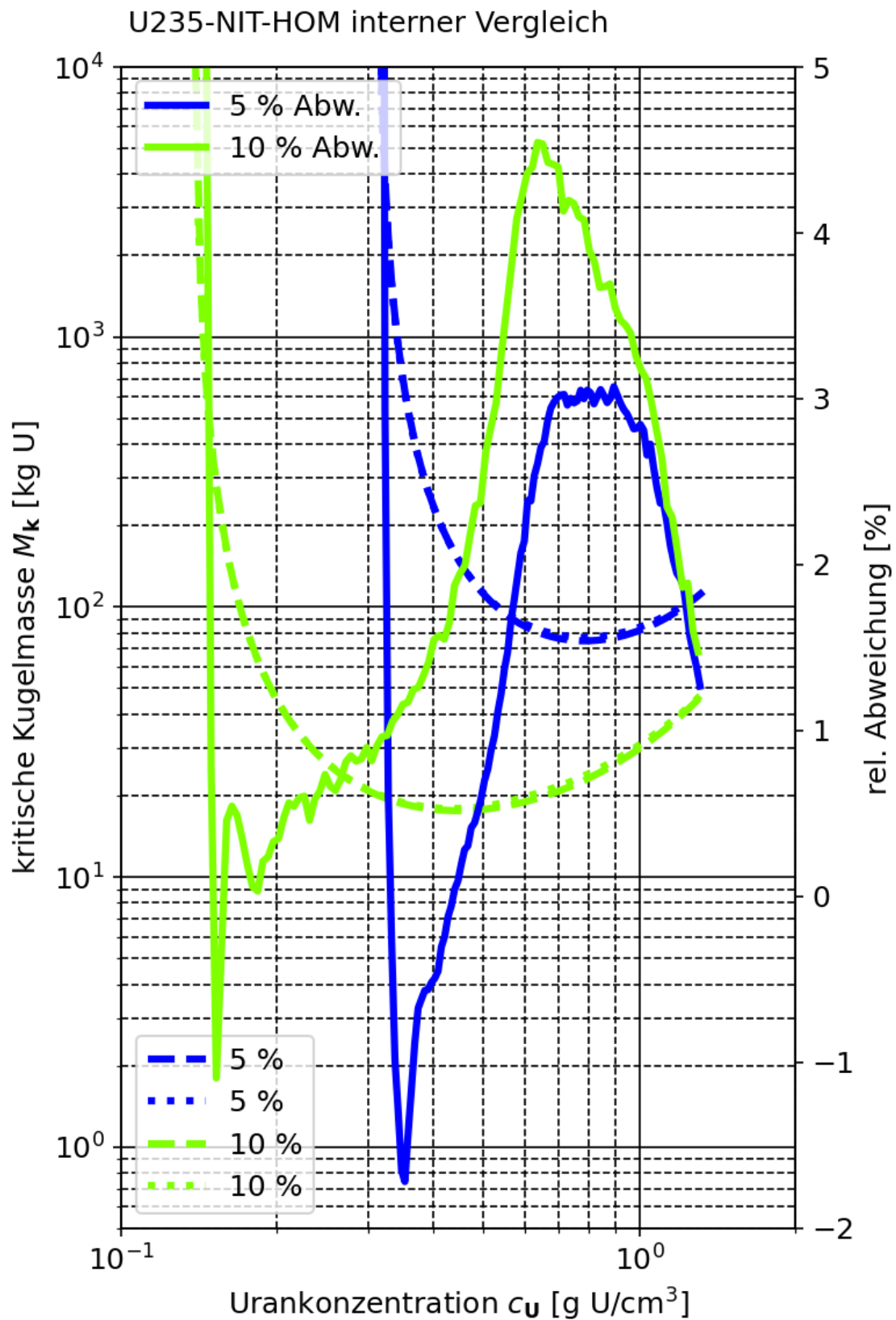
Abb. 2.2 Kritische Kugelmasse von Uranylнитrat-Wasser-Systemen. Vergleich der Rechnungen mit klassischer Volumenaddition und unter Verwendung der Dichteformel nach CRISTAL V2
