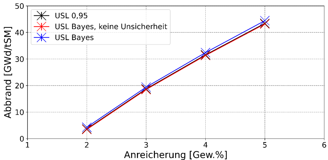
Abb. 3.24 Beladepkurven für Fall 1 (schwarz), Fall 2 ohne Betrachtung der Unsicherheit (rot) und Fall 2 nach dem Bayes Verfahren (blau)
