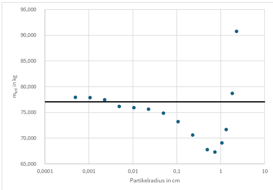
Abb. 2.6 Kritische Kugelmasse eines Uranylinitrat-Wasser-Systems mit 5 Gew.% Anreicherung in Abhängigkeit des Partikelradius
