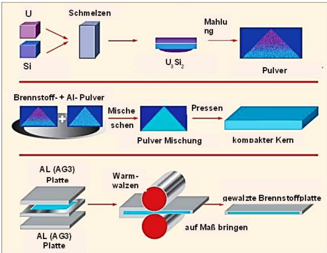
Abb. 4.13 Schematische Darstellung des gesamten Herstellungsprozesses von U_3Si_2 und der Herstellung der Brennelementplatten (unterer Bildteil) im Besonderen
