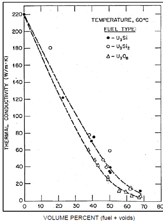
Abb. 4.14 Wärmeleitfähigkeiten der Uransilicide \text{U}_3\text{Si} , \text{U}_3\text{Si}_2 und von \text{U}_3\text{O}_8 als Funktion des Volumenanteils der Brennstoffpartikel plus Hohlräume (Porosität) bei 60 °C
