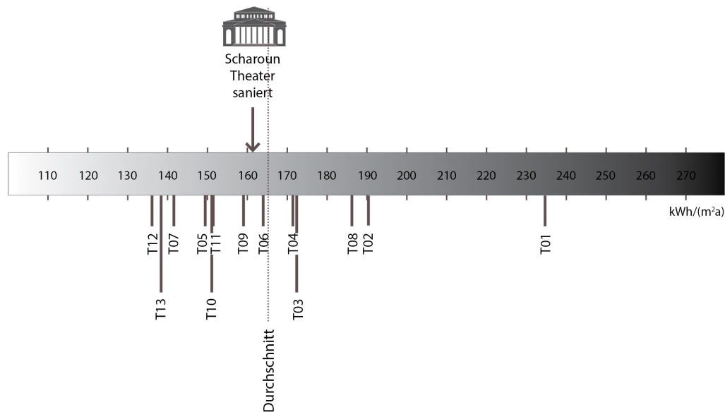
Abb. 356 Einordnung des Scharoun Theaters in das Benchmarking zum Gesamtenergieverbrauch
