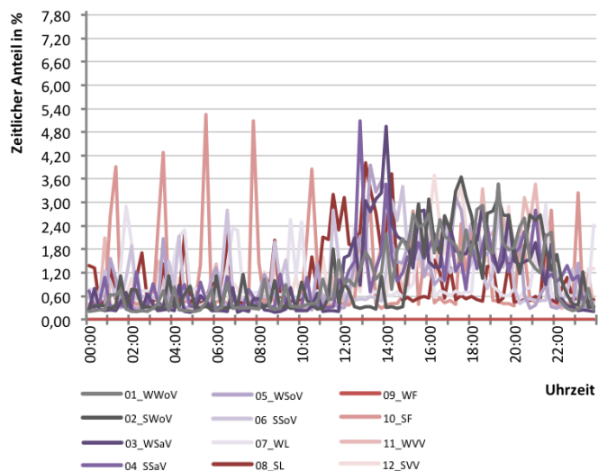
Abb. 323 Tageslastverläufe verschiedener Typtage für S02 Kantine
