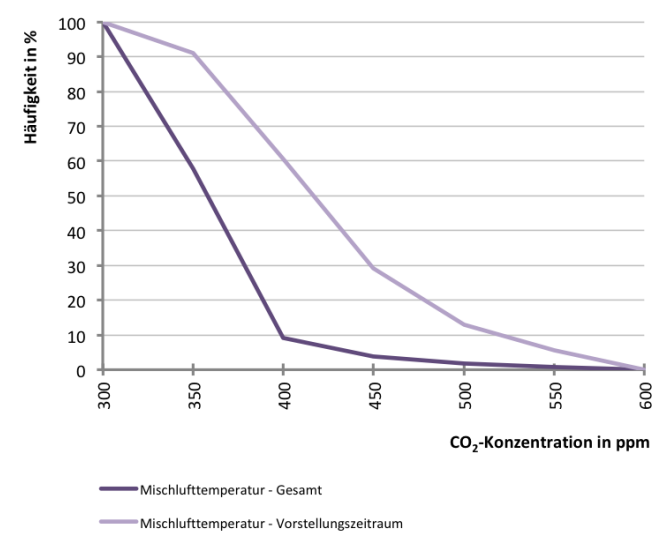
Abb. 331 Summenhäufigkeit der CO 2 -Konzentration in der Abluft
