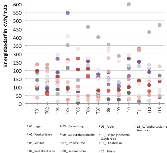
Abb. 113 Spezifischer Energiebedarf für Heizung nach Zonen
