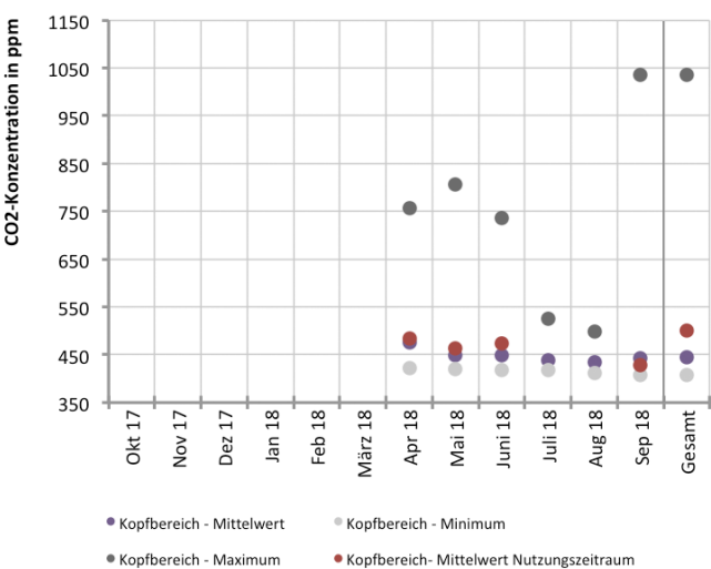
Abb. 400 Raumluftqualität während des Messzeitraums im Foyer
