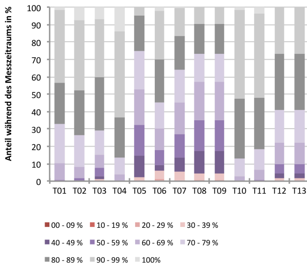
Abb. 47 Prozentuale Verteilung der gemessenen relativen Luftfeuchte
