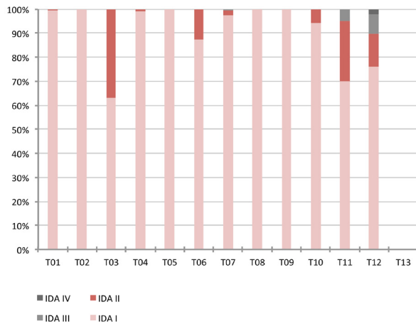
Abb. 130 Einordnung der Messwerte zur CO 2 -Konzentration in die Kategorien der Raumluftqualität
