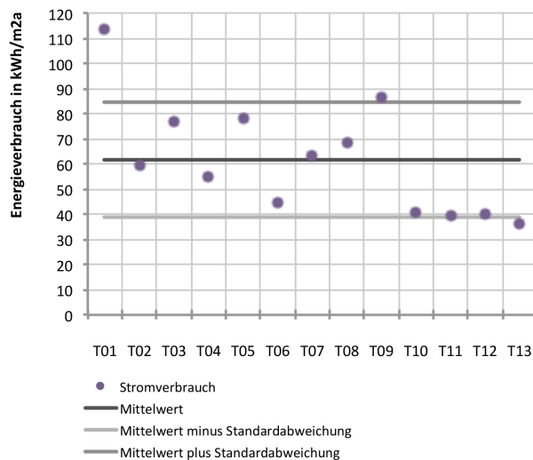
Abb. 84 Endenergieverbrauchskennwerte für Strom
