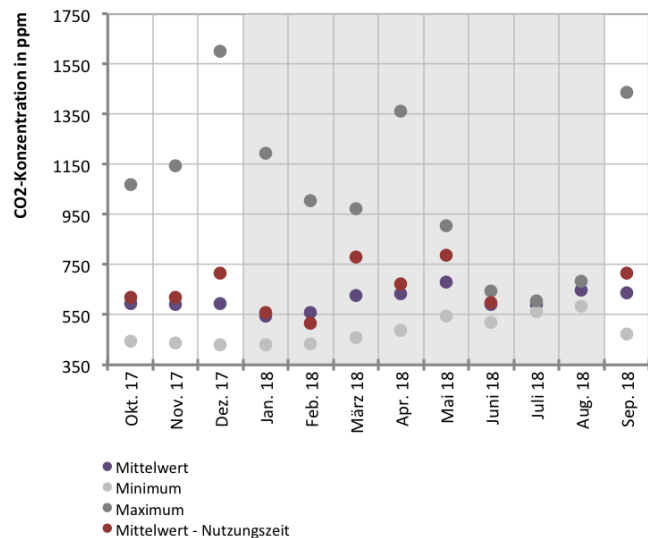
Abb. 420 CO 2 -Konzentration in der Raumluft des Proberaums während des Messzeitraums
