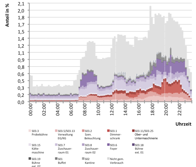
Abb. 305 Gesamter Tageslastverlauf für Typtag 03_WSaV
