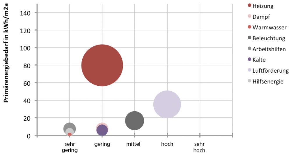
Abb. 365 TEK-Bewertung der einzelnen Verbraucher
