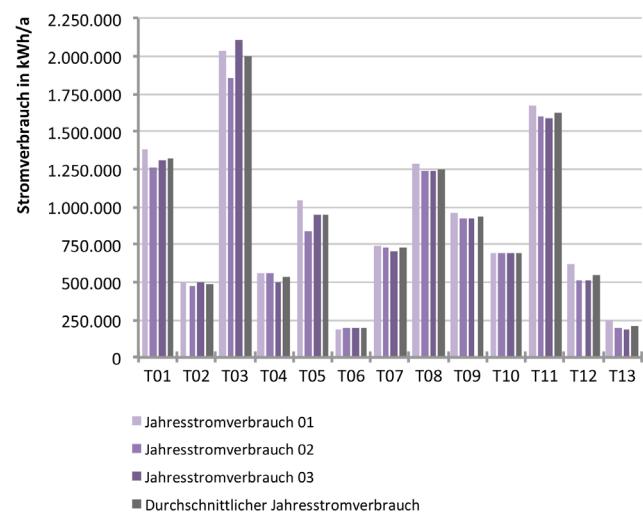
Abb. 82 Bildung des durchschnittlichen Stromverbrauchs aus drei aufeinanderfolgenden Jahren
