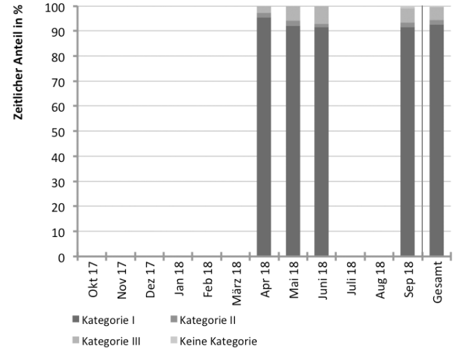
Abb. 402 Kategorisierung der Luftgeschwindigkeit während des Messzeitraums im Foyer
