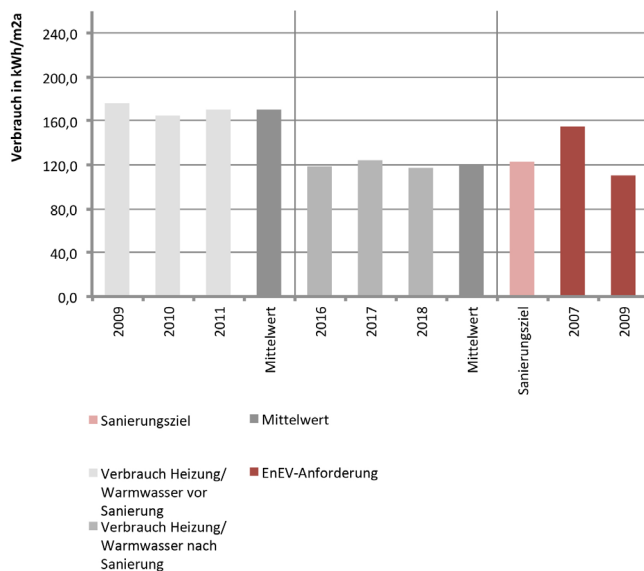
Abb. 350 Spezifischer Fernwärmeverbrauch
