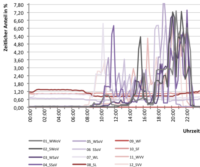
Abb. 316 Tageslastverlaufs verschiedener Typtage für S03.1 Dimmerschrank
