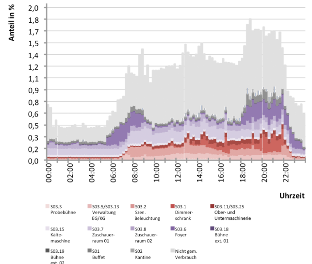
Abb. 313 Gesamtenergieverbrauch für Typtag 11_WV
