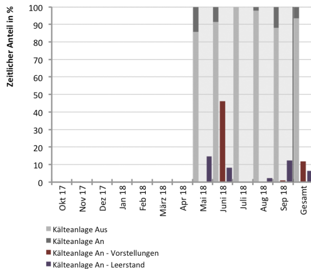
Abb. 332 Monatlicher Einschaltanteil der Kälteanlage nach Nutzungszuständen
