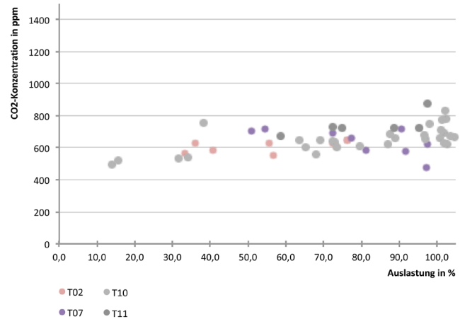
Abb. 128 Theaterspielstätten mit einem mittleren linearen Zusammenhang zwischen \text{CO}_2 -Konzentration und Auslastung
