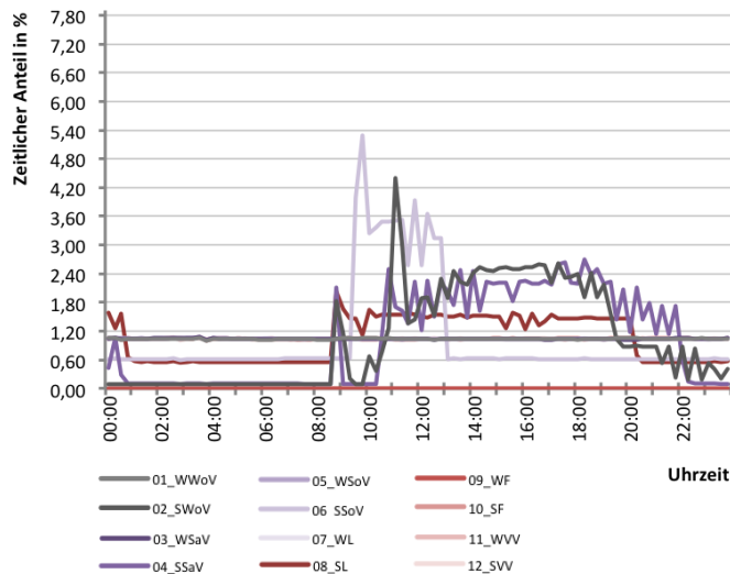
Abb. 325 Tageslastverlaufs verschiedener Typtage für S03.15 Kältemaschine
