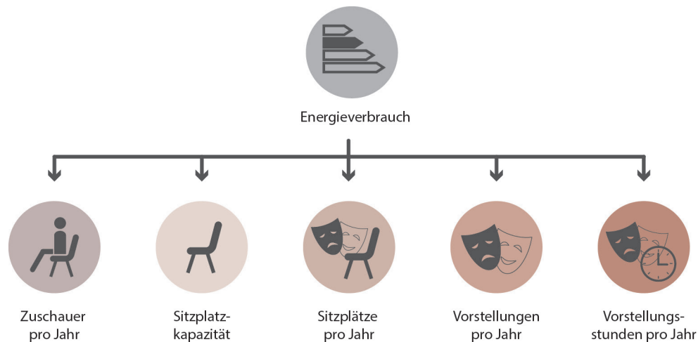
Abb. 92 Energiebezugswerte für Theaterspielstätten
