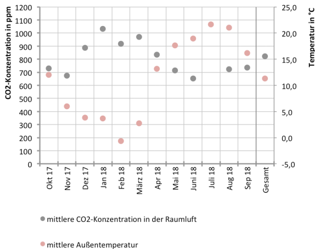
Abb. 408 Zusammenhang zwischen der mittleren CO 2 -Konzentration und der mittleren Außenlufttemperatur im beispielhaften Büroraum
