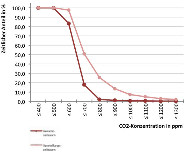
Abb. 417 Summenhäufigkeit der CO 2 -Konzentration in der Garderobe im gesamten Messzeitraum
