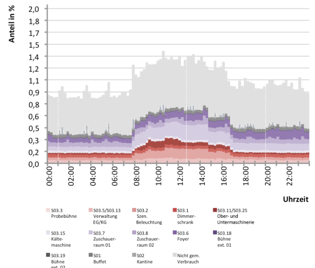
Abb. 293 Gesamter Tageslastverlauf für Typtag 10_SF
