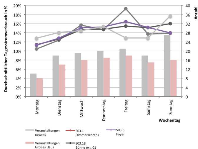
Abb. 275 Wochenstromverbrauchsanteile für S03.1 Dimmerschrank, S03.18 Bühne ext. 01 und S03.6 Foyer gegenüber der Vorstellungsanzahl
