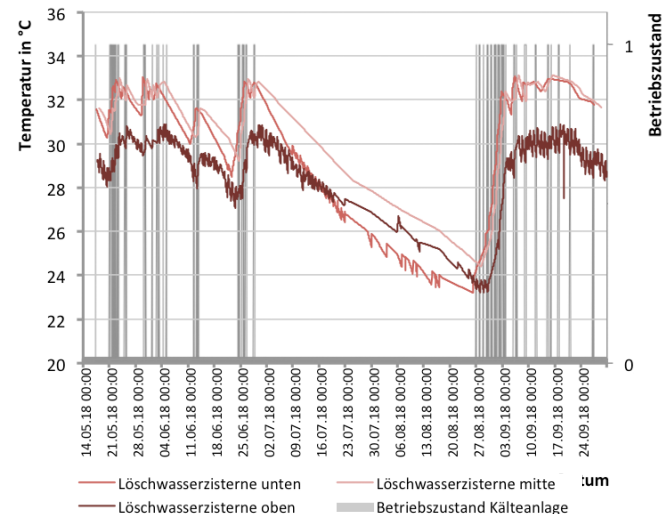
Abb. 345 Anlagenzustand gegenüber dem Temperaturverlauf in der Löschwasserzisterne im Betrachtungszeitraum
