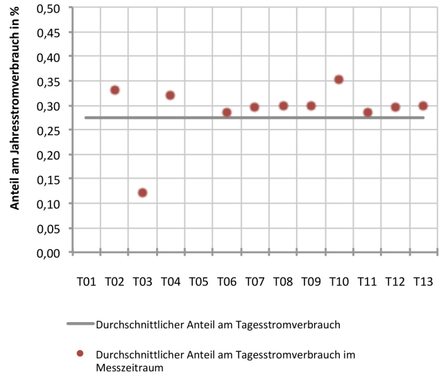
Abb. 52 Anteil des durchschnittlichen Tagesstromverbrauchs am Jahresstromverbrauch
