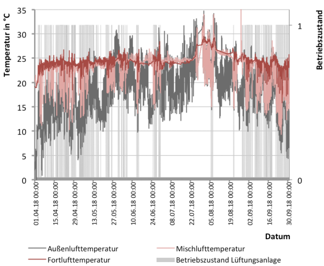
Abb. 332 Temperaturverlauf für Außen-, Fort- und Abluft in Zusammenhang mit dem Betriebszustand der Lüftungsanlage
