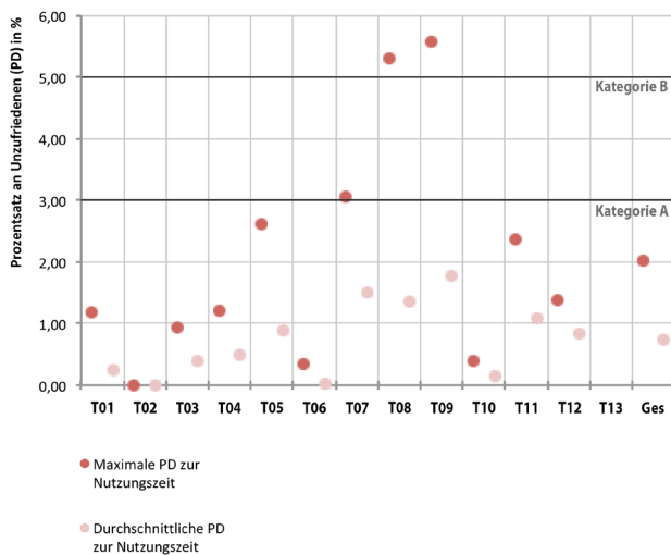
Abb. 141 Vorhergesagter prozentualer Anteil an Unzufriedenen aufgrund der vertikalen Temperaturdifferenz
