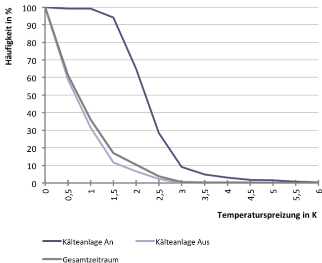
Abb. 342 Summenhäufigkeit der Temperaturspreizung zwischen Vor- und Rücklauf im Kühlkreislauf
