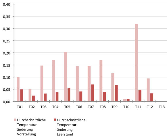
Abb. 135 Vergleich der durchschnittlichen Temperaturänderung während der Vorstellungs- und Leerstandszeiten pro Messintervall
