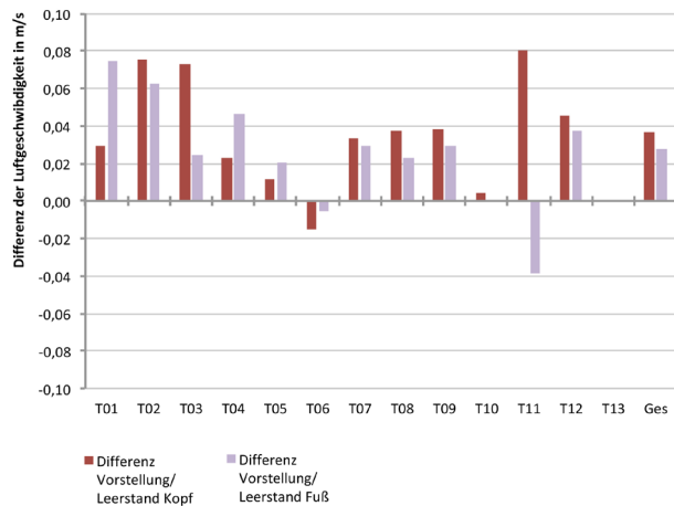
Abb. 145 Differenz der Luftgeschwindigkeit zwischen Leerstands- und Vorstellungszeiten in Abhängigkeit des Kopf- und Fußbereichs
