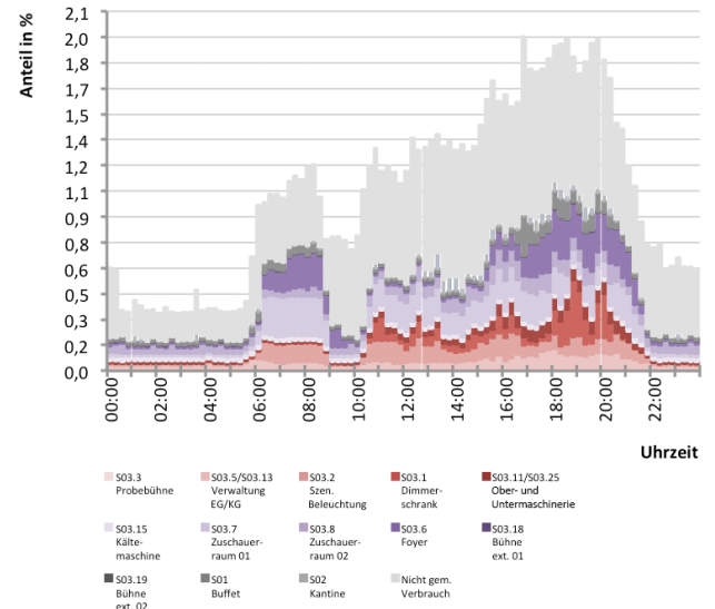
Abb. 301 Gesamtenergieverbrauch über den Tag
