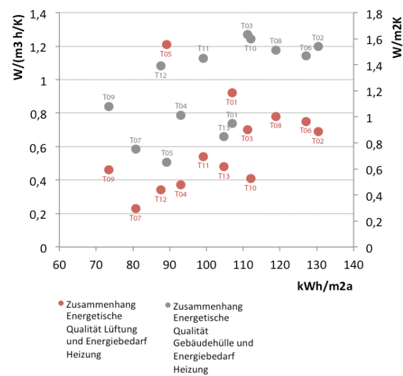
Abb. 112 Zusammenhang zwischen der Energetischen Qualität der Gebäudehülle sowie der Lüftung und dem Energiebedarf für Heizung
