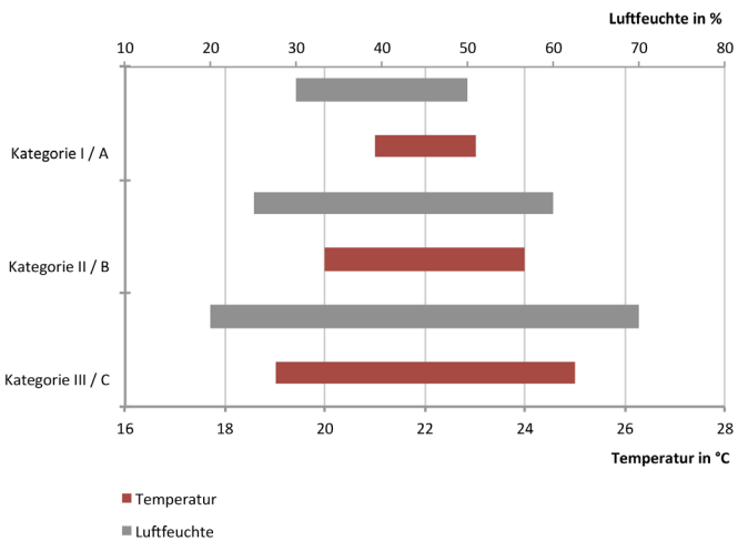
Abb. 123 Anforderungsbereiche für Relative Luftfeuchte und Operative Temperatur nach den Kategorien
