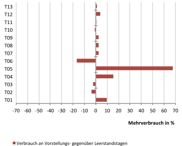
Abb. 54 Verhältnis des Verbrauchs an Vorstellungs- gegenüber Leerstandstagen
