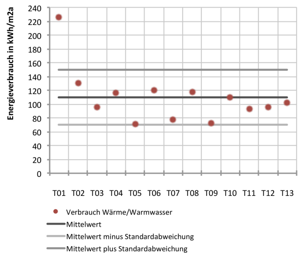
Abb. 85 Endenergieverbrauchskennwerte für Heizung/Warmwasser
