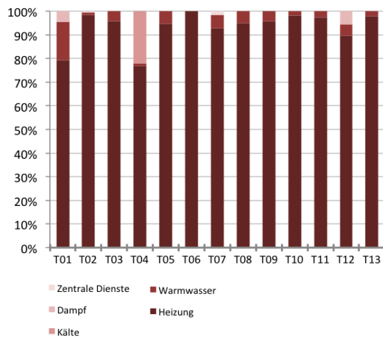
Abb. 108 Anteile der Verbraucher am Bedarf für Brennstoffe, bzw. Fernwärme
