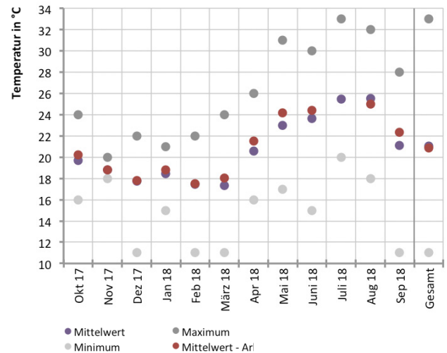
Abb. 410 Raumlufttemperatur während des Messzeitraums im beispielhaften Büroraum
