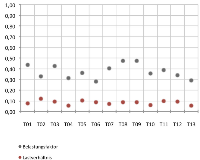
Abb. 57 Belastungsfaktor und Lastverhältnis im Stromlastgang
