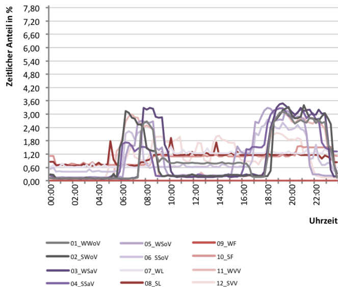
Abb. 318 Tageslastverlaufs verschiedener Typtage für S03.6 Foyer
