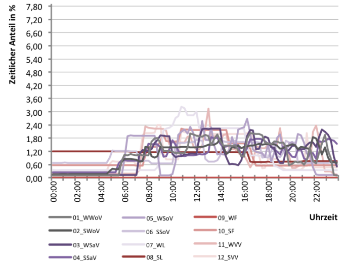
Abb. 322 Tageslastverlaufs verschiedener Typtage für S03.2 Szenische Beleuchtung
