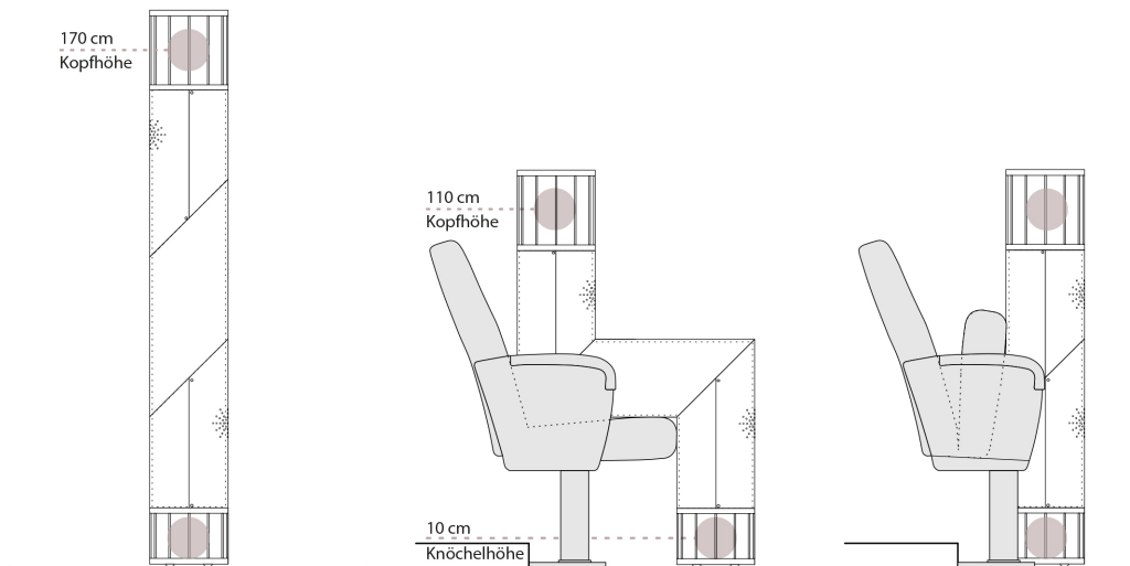
Abb. 28 Platzierung der Sensoren am Messtorso
