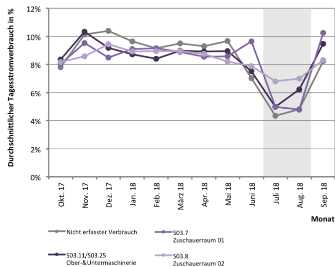
Abb. 271 Monatsstromverbrauchsanteile im Zuschauersaal und für die Bühnentechnik
