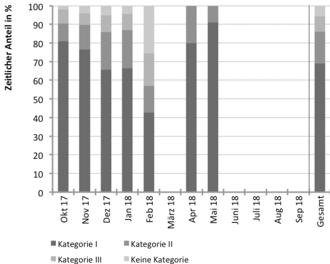
Abb. 380 Kategorisierung der Luftgeschwindigkeit während des Messzeitraums im Zuschauersaal
