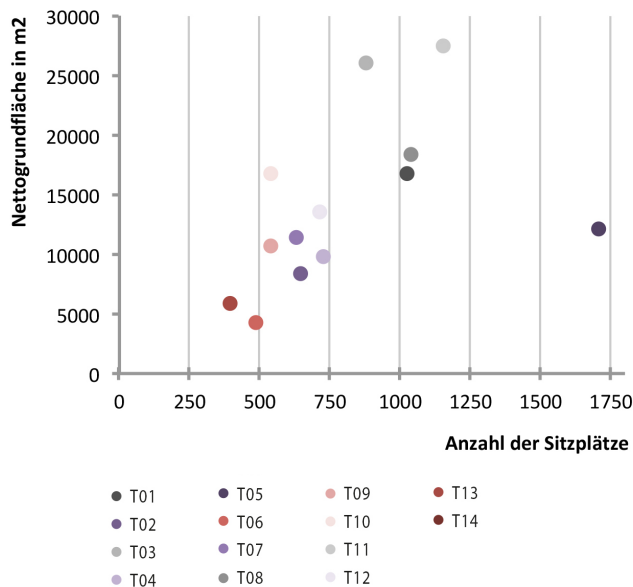
Abb. 36 Beziehung zwischen Nettogrundfläche und Sitzplatzkapazität ohne Nebenspielstätten
