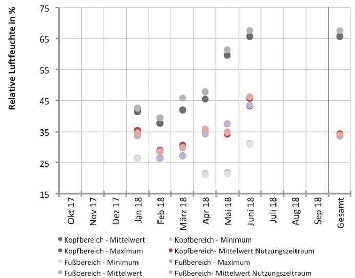
Abb. 389 Relative Luftfeuchte im Kopf- und Fußbereich während des Messzeitraums im Rang des Zuschauersaals
