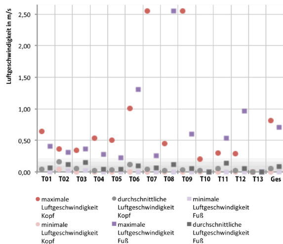
Abb. 143 Minimale, maximale und durchschnittliche Luftgeschwindigkeit im Zuschauersaal nach Fuß- und Kopfbereich
