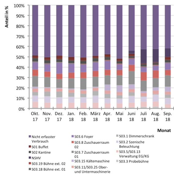
Abb. 267 Prozentuale monatliche Zusammensetzung des Stromverbrauchs nach Stromkreisen
