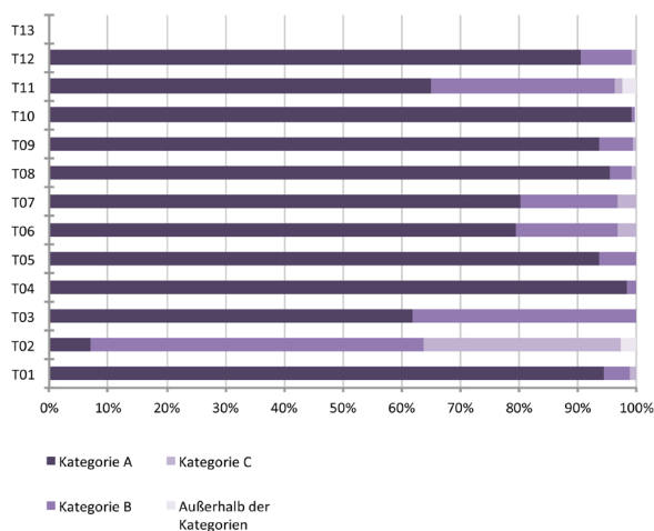
Abb. 147 Kategorisierung der Luftgeschwindigkeiten mithilfe des Draught Rating
