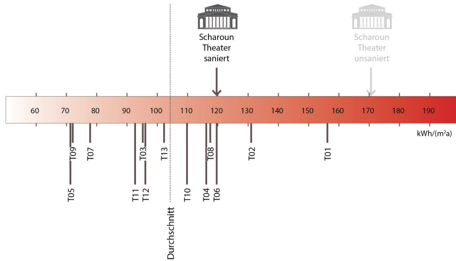
Abb. 354 Einordnung des Scharoun Theaters in das Benchmarking zum flächenbezogenen Verbrauch für Heizung/Warmwasser
