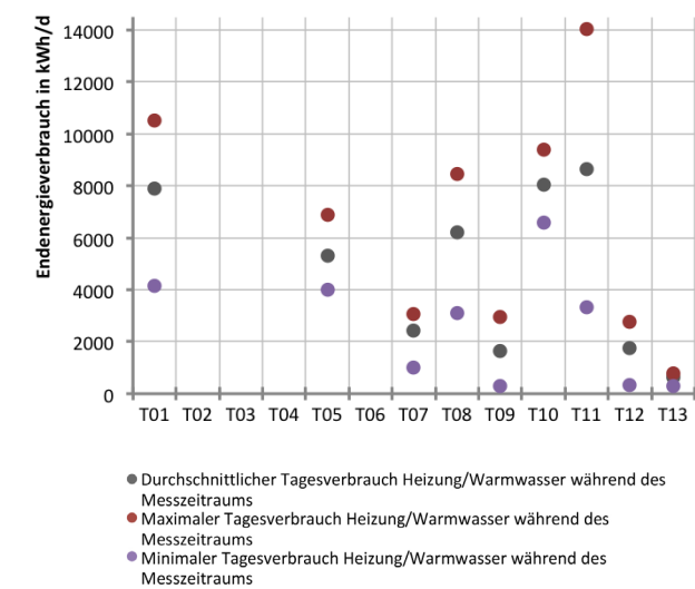
Abb. 64 Absoluter Tagesverbrauch für Heizung/Warmwasser während des Messzeitraums
