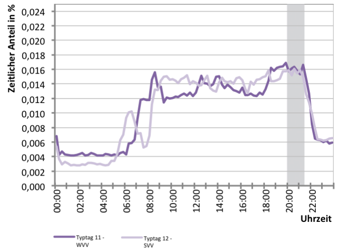
Abb. 289 Referenzlastprofil für Tage mit Vorstellungen auf der Hinterbühne
