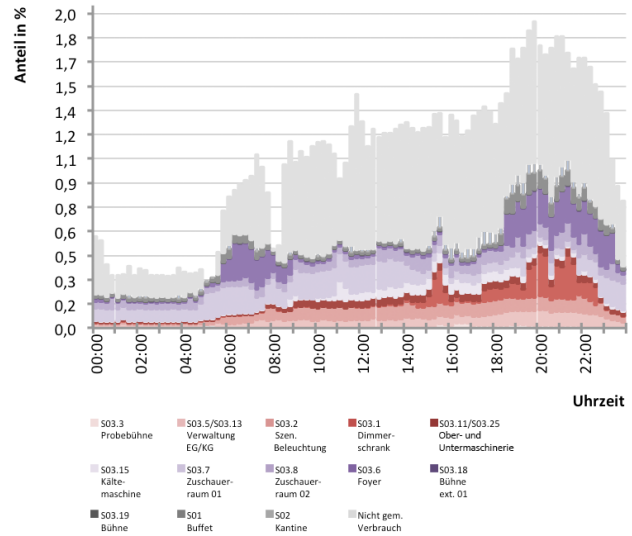
Abb. 307 Gesamter Tageslastverlauf für Typtag 02_SWoV
