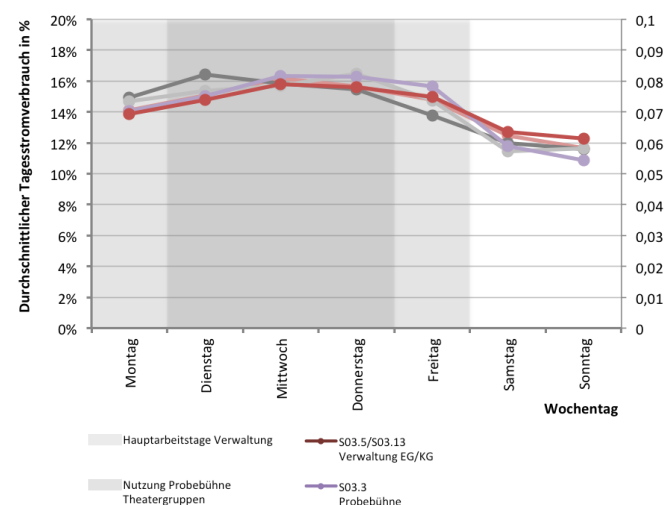
Abb. 276 Wochenstromverbrauchsanteile für S03.5/S03.13 Verwaltung EG/KG sowie S03.3 Probebühne gegenüber der Nutzungszeit
