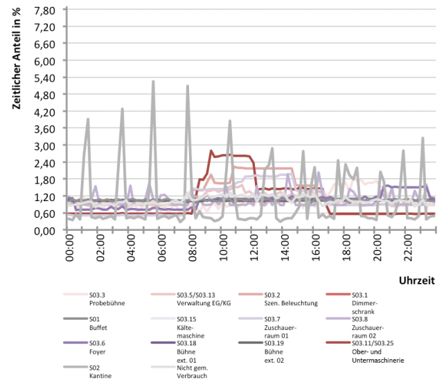
Abb. 294 Tageslastverlauf der einzelnen Stromkreise für Typtag 10_SF
