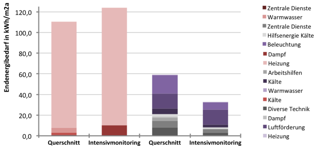
Abb. 367 Spezifischer Bedarf der einzelnen Verbraucher nach Energieträger
