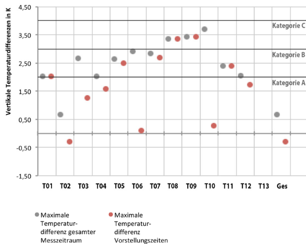
Abb. 139 Vertikale Temperaturdifferenz nach Nutzungszustand
