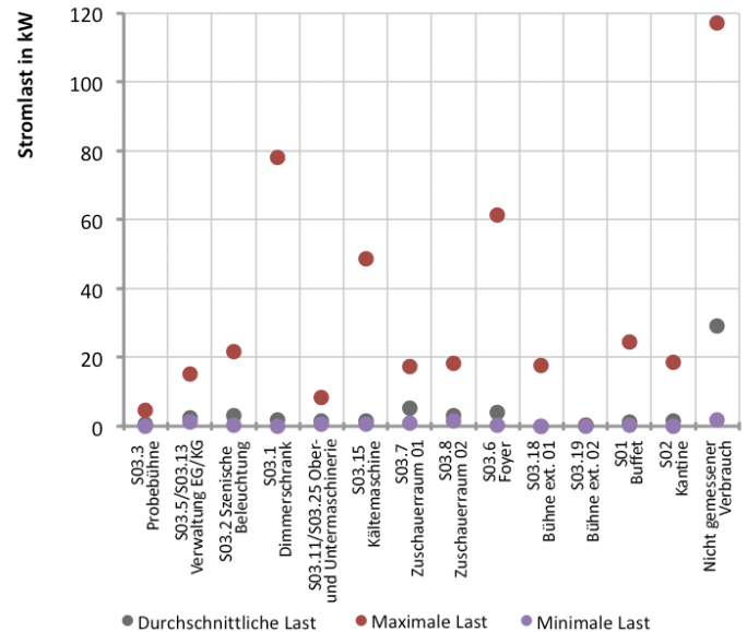
Abb. 284 Maximale, minimale und durchschnittliche Lasten in den einzelnen Stromkreisen
