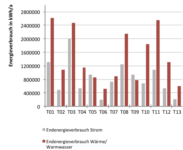
Abb. 83 Absoluter Endenergieverbrauch für Strom und Wärme/Warmwasser
