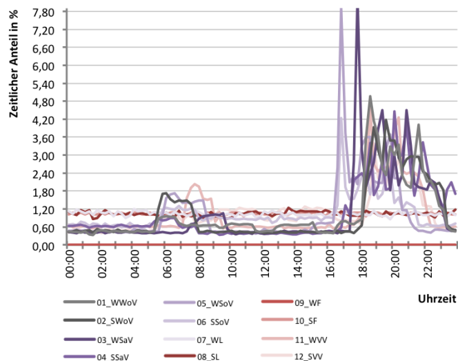
Abb. 324 Tageslastverläufe verschiedener Typtage für S01 Buffet
