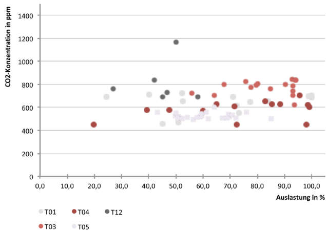
Abb. 127 Theaterspielstätten mit einem schwachen linearen Zusammenhang zwischen \text{CO}_2 -Konzentration und Auslastung
