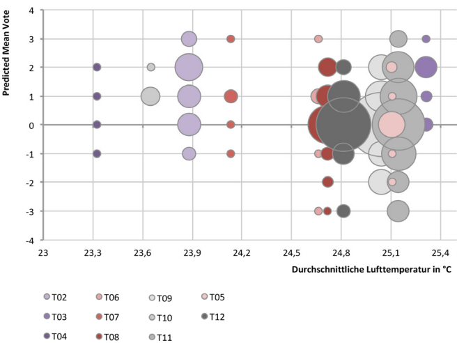
Abb. 190 Befragungsergebnisse zur empfundenen Lufttemperatur über den PMV in Abhängigkeit der durchschnittlichen Lufttemperaturen während der Vorstellungen
