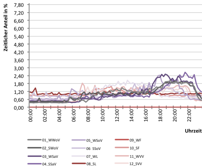
Abb. 321 Tageslastverlaufs verschiedener Typtage für S03.5/S03.13 Verwaltung EG/KG
