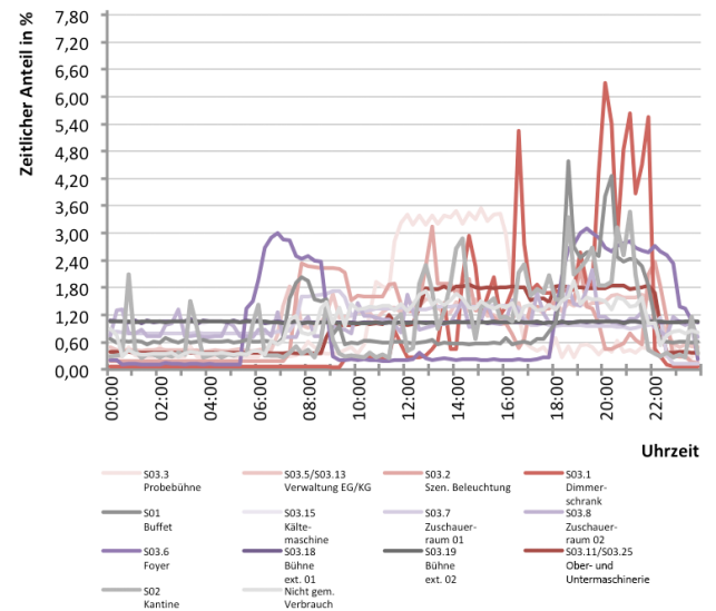
Abb. 314 Tageslastverlauf der einzelnen Stromkreise für Typtag 11_WV
