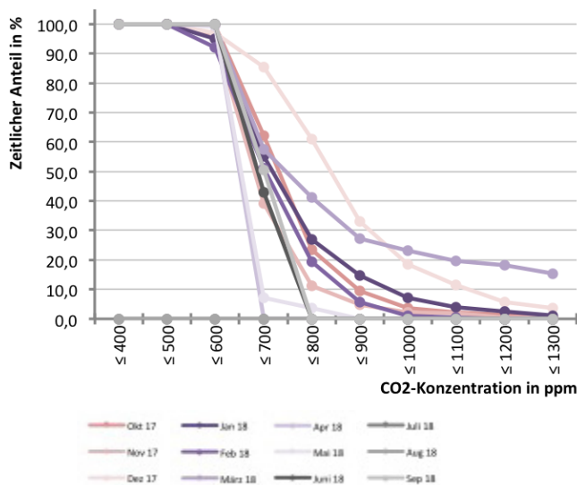
Abb. 418 Summenhäufigkeit der \text{CO}_2 -Konzentration in der Garderobe nach Monaten
