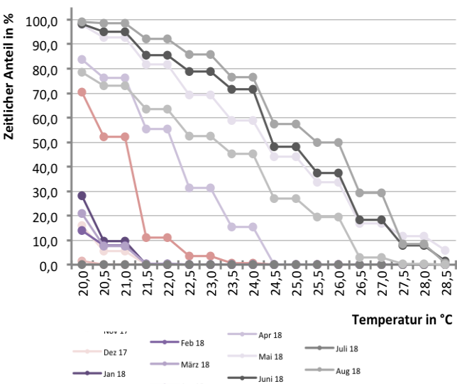
Abb. 412 Summenhäufigkeit der Raumlufttemperatur im beispielhaften Büroraum
