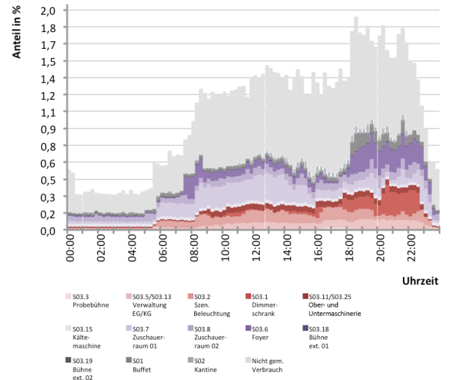
Abb. 309 Gesamter Tageslastverlaufs für Typtag 01_WWoV
