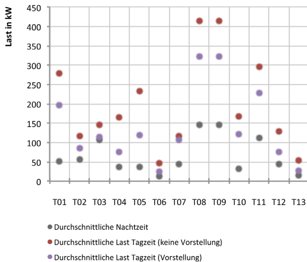
Abb. 59 Durchschnittslasten in Abhängigkeit der Tageszeiten
