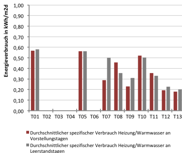
Abb. 68 Durchschnittlicher spezifischer Verbrauch für Heizung/ Warmwasser an Vorstellungstagen und Leerstandstagen
