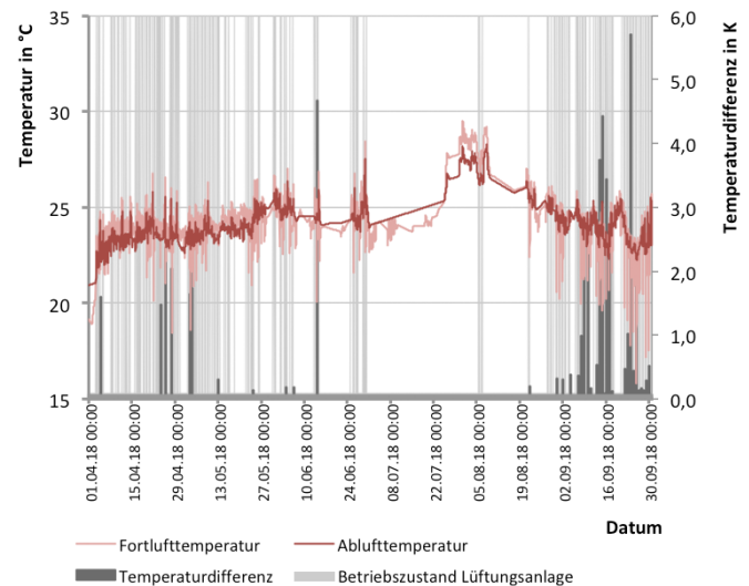
Abb. 334 Temperaturverlaufs der Ab- und Fortluft sowie der Temperaturdifferenzen
