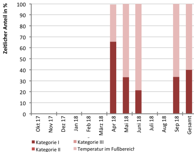
Abb. 403 Kategorisierung der vertikalen Temperaturdifferenz während des Messzeitraums im Foyer
