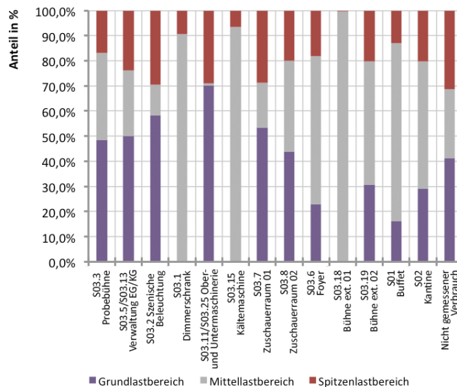
Abb. 286 Anteilige Lastverteilung auf Grund-, Mittel- und Spitzenlastbereich für die einzelnen Stromkreise
