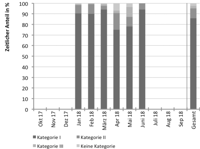
Abb. 393 Kategorisierung der Vertikalen Temperaturdifferenz während des Messzeitraums im Rang des Zuschauersaals
