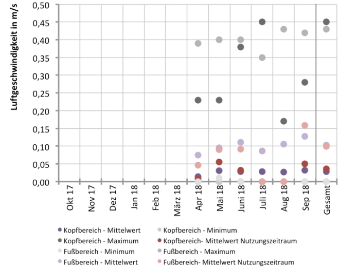
Abb. 401 Luftgeschwindigkeit im Kopf- und Fußbereich während des Messzeitraums im Foyer
