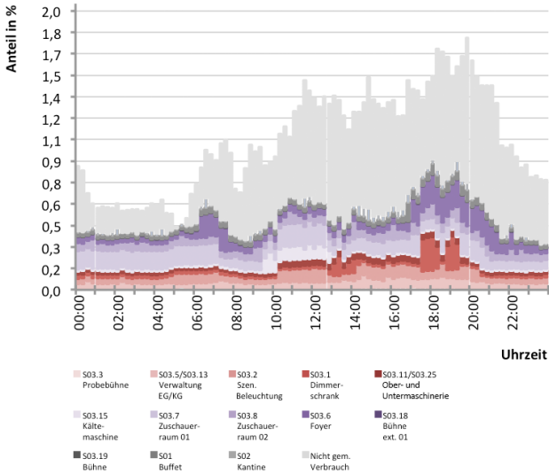
Abb. 299 Gesamter Tageslastverlauf für Typtag 06_SSoV
