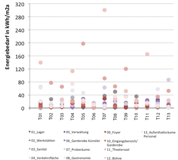
Abb. 114 Spezifischer Energiebedarf für Beleuchtung nach Zonen
