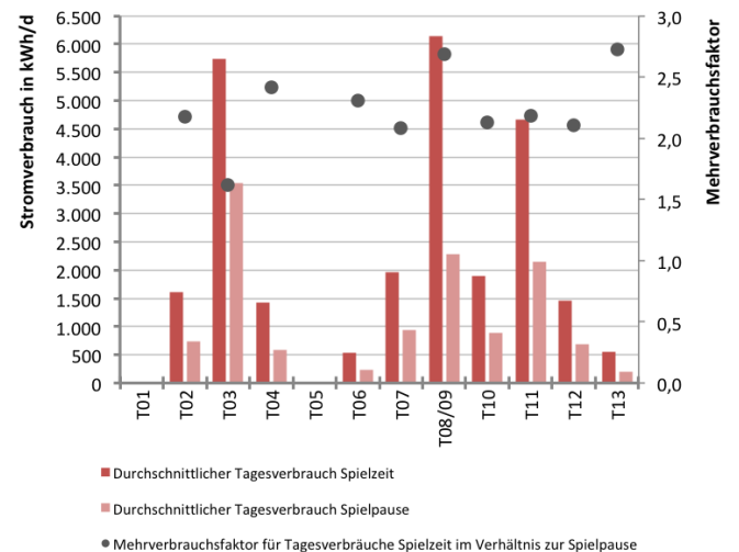
Abb. 72 Durchschnittlicher Tagesstromverbrauch während der Spielzeit und der Spielpause
