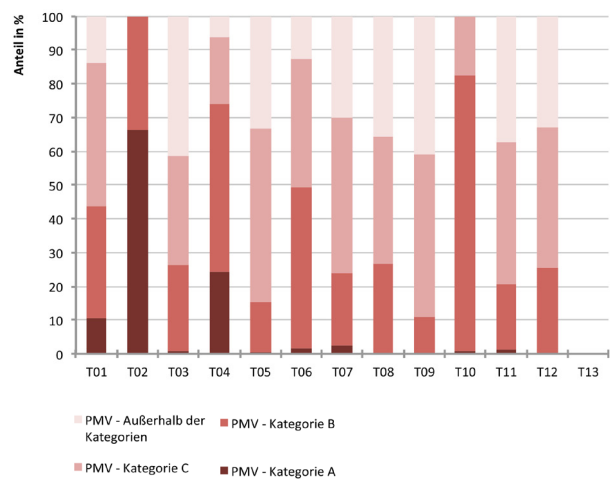
Abb. 155 Kategorisierung nach PMV in den Theaterspielstätten
