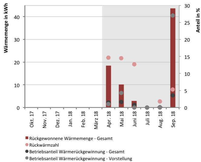
Abb. 335 Monatlicher Nutzungsanteils der Wärmerückgewinnung während der Betriebszeiten der Lüftungsanlage und rückgewonnene Wärmemenge
