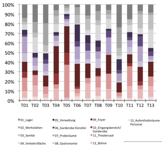
Abb. 110 Anteile der Zonen am Endenergiebedarf
