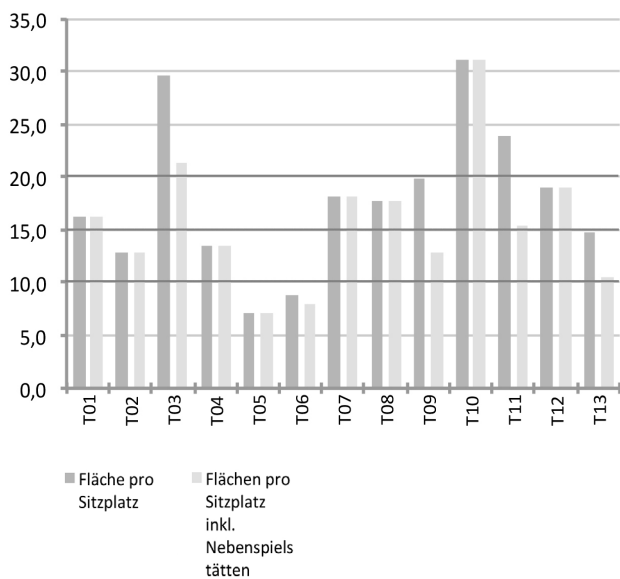
Abb. 35 Nettogrundfläche bezogen auf die Sitzplatzkapazität der Theaterspielstätten
