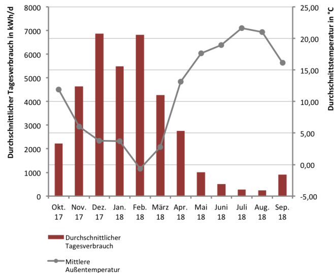
Abb. 281 Durchschnittlicher Tagesverbrauch für Heizung/ Warmwasser gegenüber der mittleren Außentemperatur
