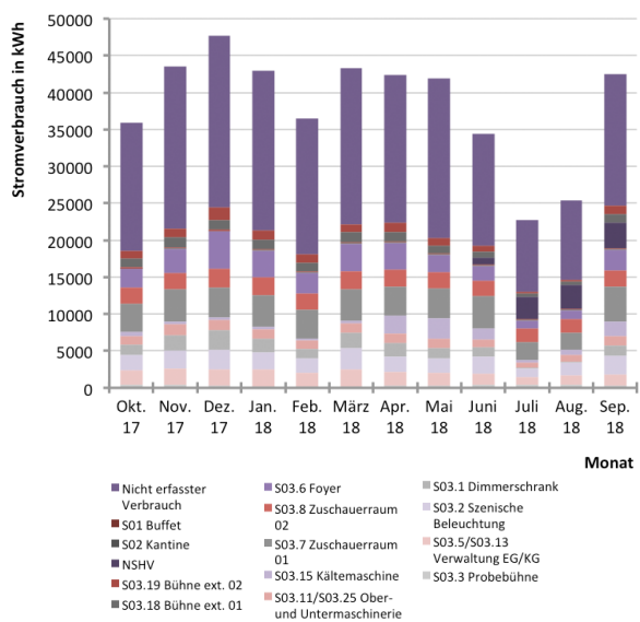
Abb. 268 Absolute monatliche Zusammensetzung des Stromverbrauchs nach Stromkreisen
