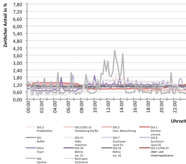
Abb. 298 Tageslastverlaufs der einzelnen Stromkreise für Tytag 08_SL
