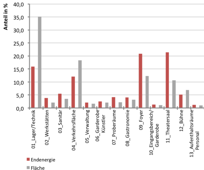
Abb. 362 Anteile der Zonen am Endenergiebedarf gegenüber des Anteils an der beheizten Nettogrundfläche
