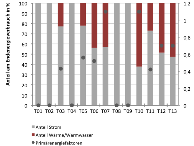
Abb. 90 Gegenüberstellung der Verbrauchsanteile für Strom und Wärme/Warmwasser auf primärenergetischer Ebene
