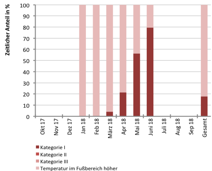
Abb. 394 Kategorisierung der vertikalen Temperaturdifferenz während des Messzeitraums
