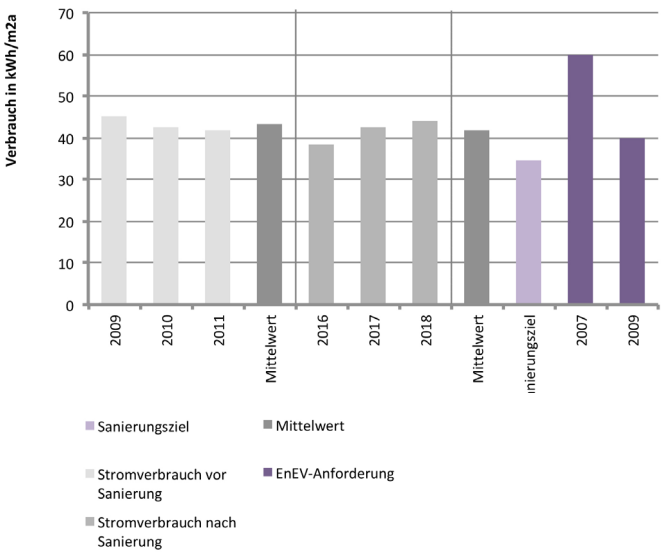
Abb. 348 Spezifischer Stromverbrauch
