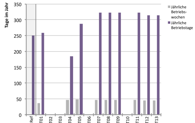
Abb. 206 Jährlichen Betriebswochen und –Tage der RLT-Anlage für das Theater-Foyer
