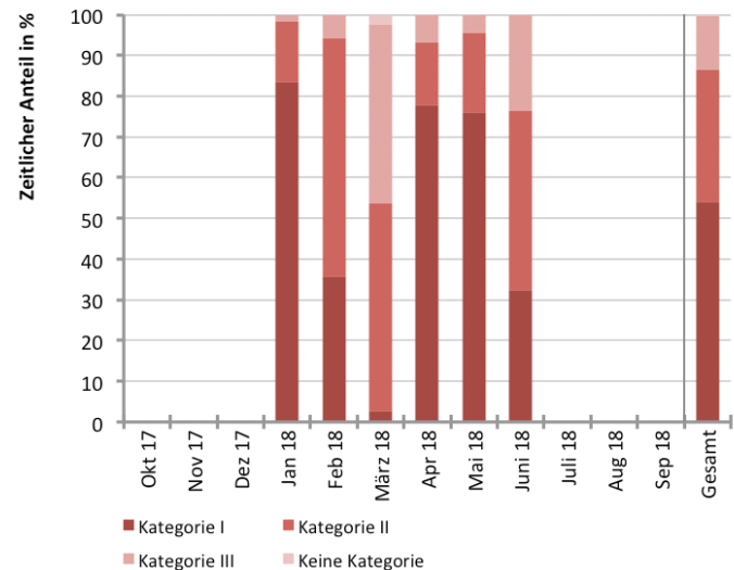
Abb. 387 Kategorisierung der Lufttemperatur während des Messzeitraums im Rang des Zuschauersaals
