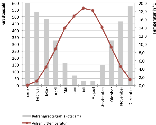
Abb. 41 Referenzklima des Standorts Potsdam
