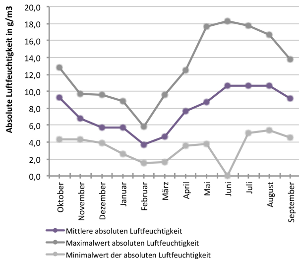
Abb. 258 Monatliche absolute Luftfeuchte im Messzeitraum am Standort Wolfsburg
