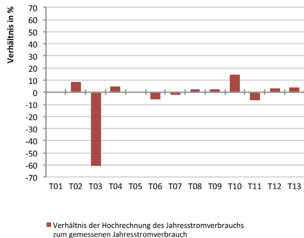
Abb. 77 Verhältnis des hochgerechneten zum gemessenen Jahresstromverbrauch
