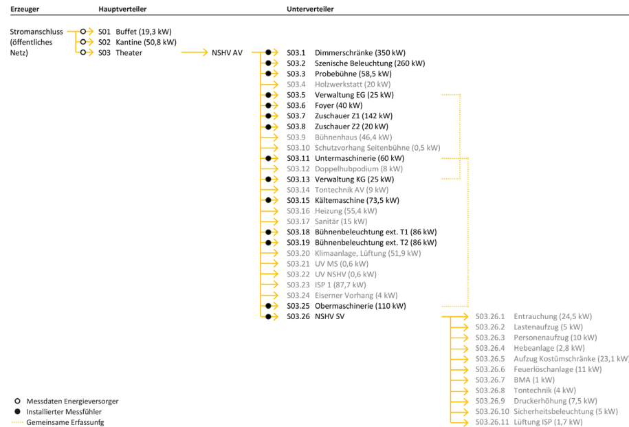
Abb. 249 Messstellen Stromverbrauch
