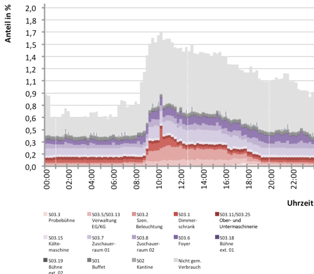
Abb. 295 Gesamtenergieverbrauch über den Tag für Typtag 07_WL
