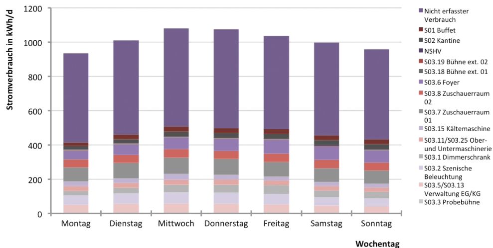
Abb. 274 Absolute wöchentliche Zusammensetzung des Stromverbrauchs aus den Stromkreisen
