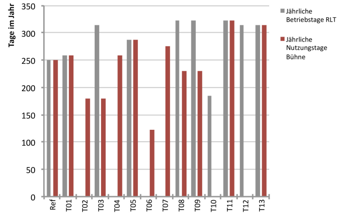
Abb. 208 Jährlichen Nutzungs- und Betriebstage für die Bühne
