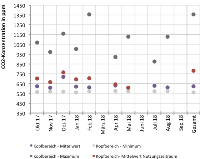
Abb. 384 Raumlufthqualität während des Messzeitraums im Zuschauersaal
