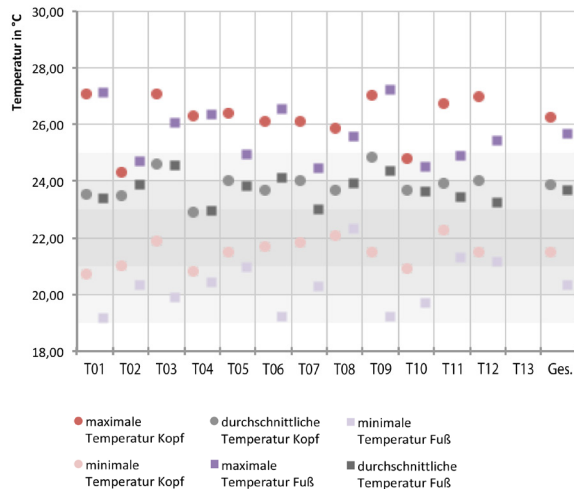
Abb. 131 Minimale, maximale und durchschnittliche Lufttemperaturen in den Theaterspielstätten
