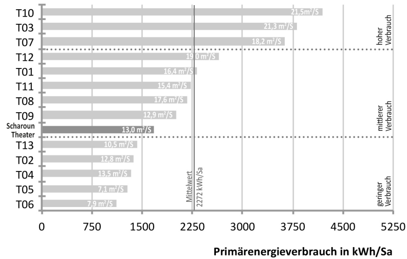
Abb. 357 Einordnung des Scharoun Theaters in das Benchmarking zum sitzplatzbezogenen Primärenergieverbrauch
