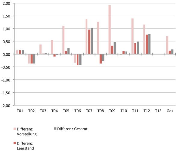
Abb. 138 Temperaturdifferenz zwischen Kopf- und Fußbereich nach Nutzungszustand
