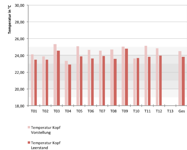
Abb. 133 Vergleich der durchschnittlichen Lufttemperaturen während der Vorstellungen und der Leerstandszeiten
