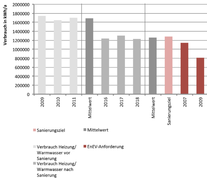
Abb. 351 Absoluter Fernwärmeverbrauch
