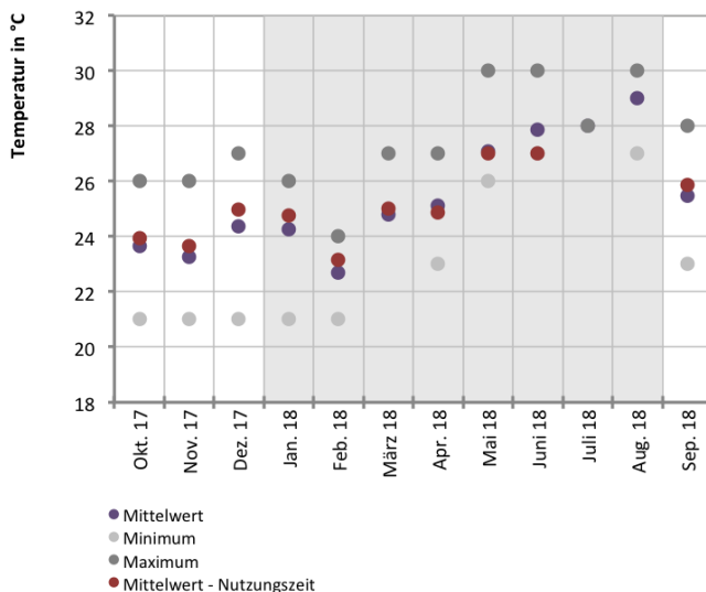
Abb. 421 Raumlufttemperatur im Proberaum während des Messzeitraums
