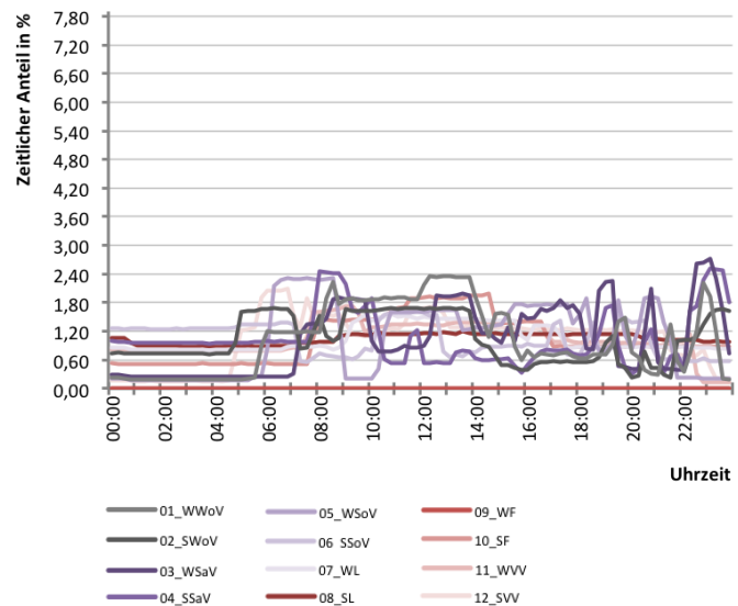
Abb. 317 Tageslastverlaufs verschiedener Typtage für S03.7 Zuschauerraum 01
