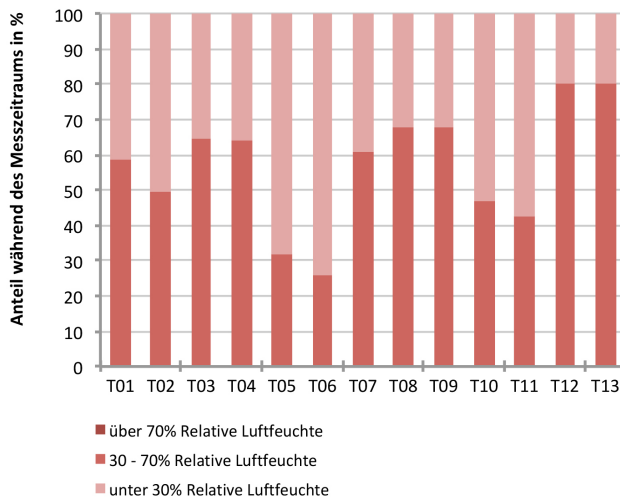
Abb. 49 Potentieller zeitlicher Anteil relativer Luftfeuchten für die Norminnenraumtemperatur in Abhängigkeit der absoluten Außenluftfeuchte
