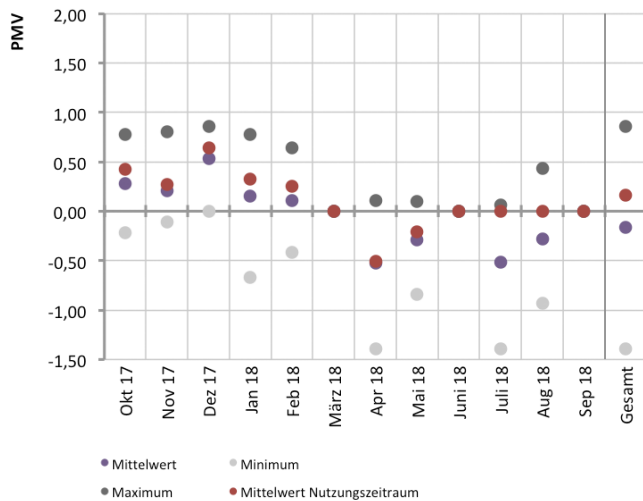
Abb. 382 Durchschnittliches PMV während des Messzeitraums im Zuschaueraal
