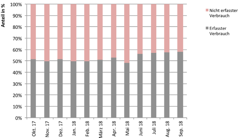
Abb. 265 Monatlicher Anteil des erfassten und nicht erfassten Stromverbrauchs
