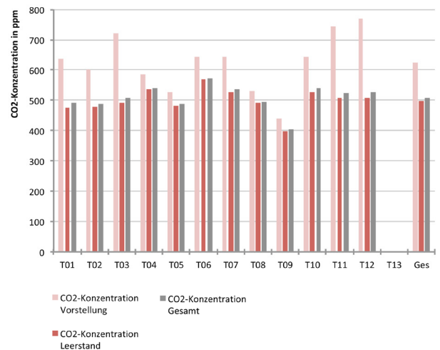
Abb. 126 Durchschnittlichen \text{CO}_2 -Konzentrationen während der Nutzungs- und des Leerstandszeiten
