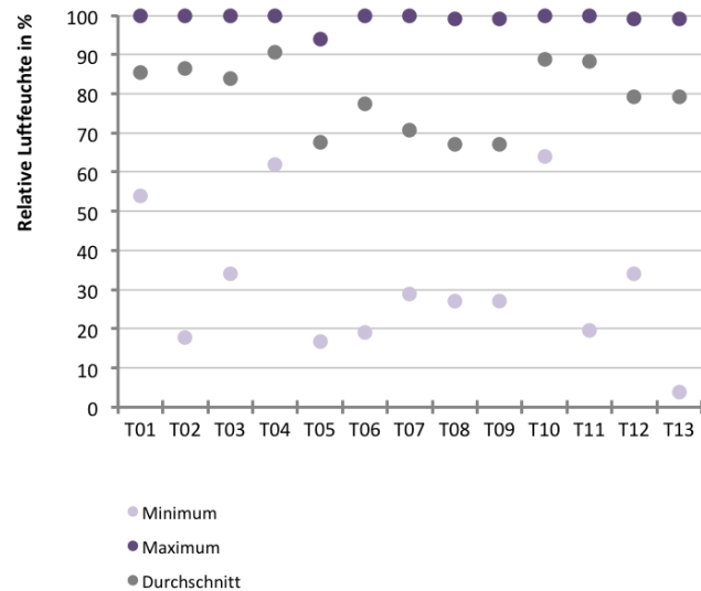
Abb. 46 Relative Außenluftfeuchte am Standort der Theaterspielstätten während des Messzeitraums
