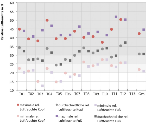
Abb. 148 Minimale, maximale und durchschnittliche relative Luftfeuchte im Zuschauersaal nach Fuß- und Kopfbereich
