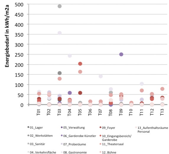
Abb. 115 Spezifischer Energiebedarf für Luftförderung nach Zonen
