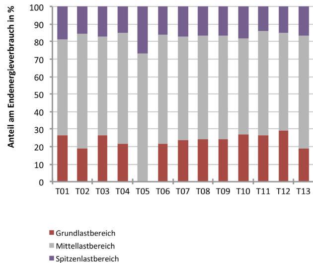
Abb. 58 Prozentuale Verteilung der Lasten auf Grund-, Mittel- und Spitzenlastbereich
