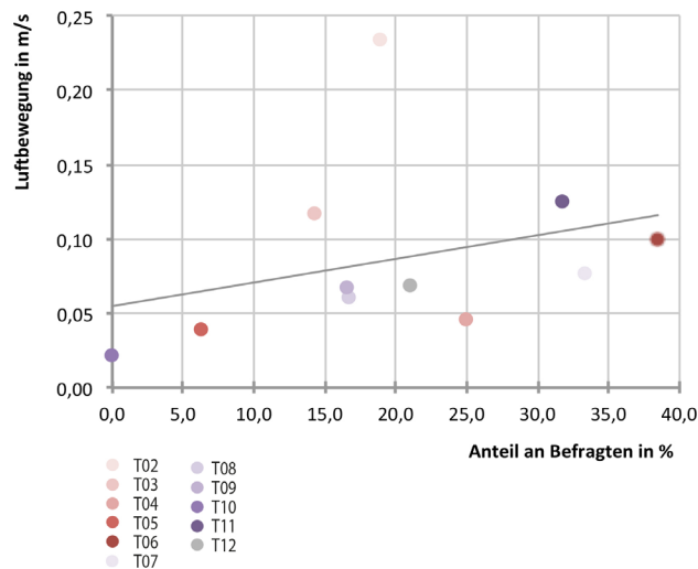
Abb. 183 Durchschnittliche gemessene Luftgeschwindigkeit während der Vorstellungszeiten gegenüber dem Anteil an Befragten, die angegeben haben, Zugerscheinungen wahrzunehmen
