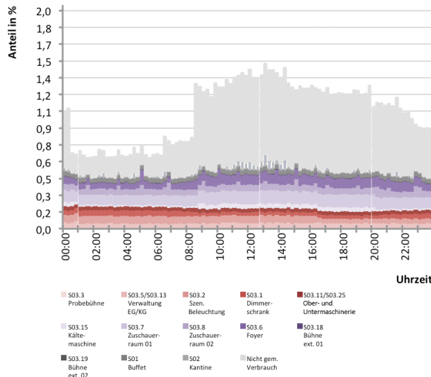
Abb. 297 Gesamtenergieverlaufs für Tytag 08_SL
