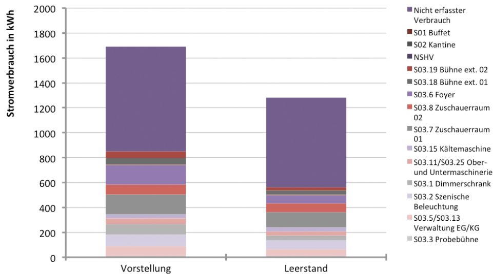
Abb. 279 Durchschnittlichen täglichen Stromverbrauchs zusammensetzung aus den Stromkreisen für Vorstellung- und Leerstandstage
