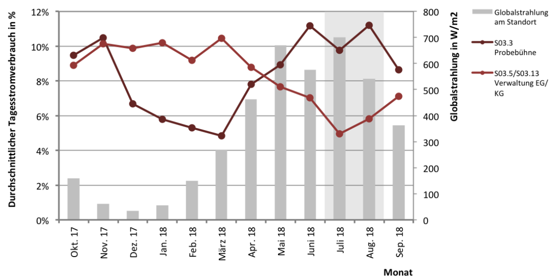
Abb. 273 Monatsstromverbrauchsanteile der Probebühne gegenüber der Globalstrahlung
