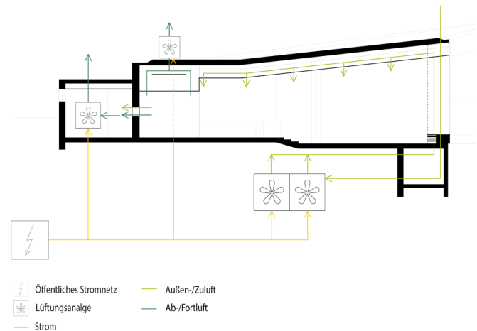
Abb. 236 Funktionsschema der Lüftungsanlage „03 Foyer/Cafeteria/Sanitärbereich“
