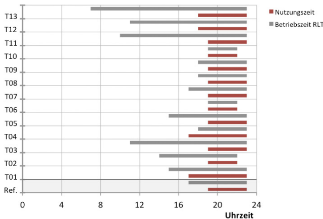
Abb. 196 Nutzungs- und Betriebszeiten der RLT-Anlagen für den Zuschauerbereich
