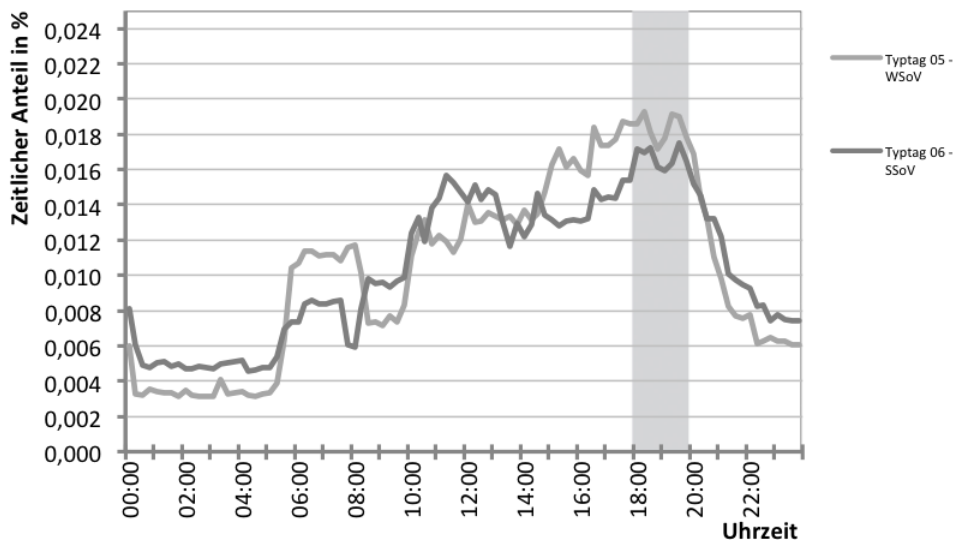
Abb. 292 Referenzlastprofils für Tage mit Vorstellungen an Sonntagen
