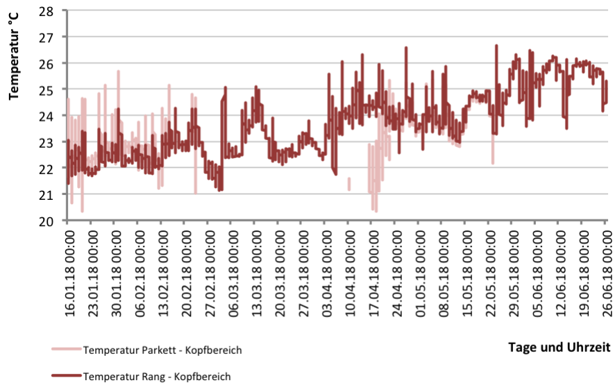
Abb. 388 Lufttemperaturverlauf im Rang und im Parkett für den Kopfbereich
