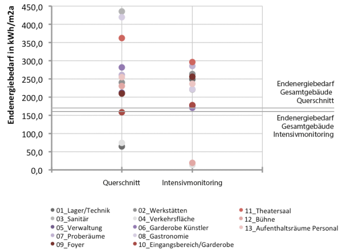
Abb. 369 Spezifischer Endenergiebedarf der einzelnen Zonen
