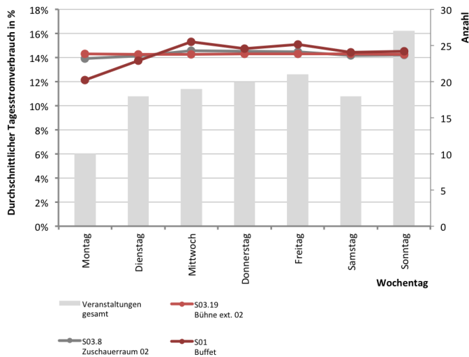
Abb. 277 Wochenstromverbrauchsanteil verschiedener Stromkreise gegenüber der Vorstellungsanzahl
