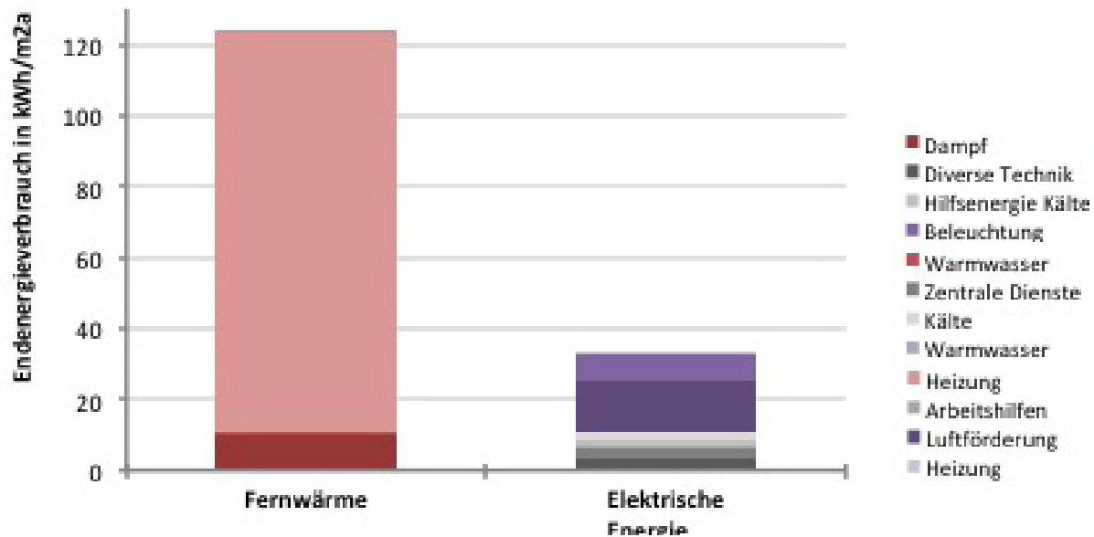
Abb. 360 Zusammensetzung der Bedarfsanteile
