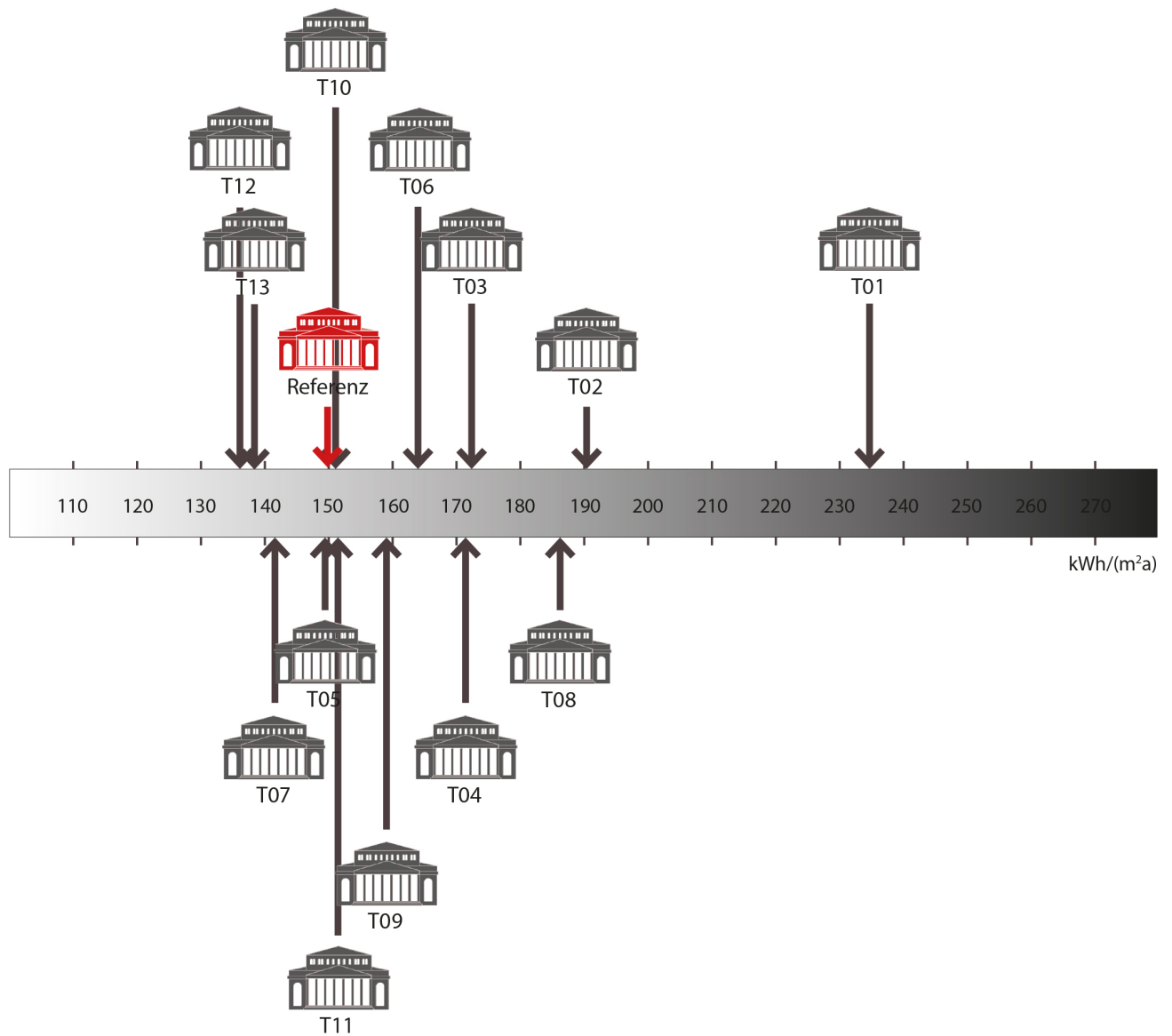
Abb. 98 Benchmarking des flächenbezogenen Gesamtenergieverbrauchs auf endenergetischer Ebene
