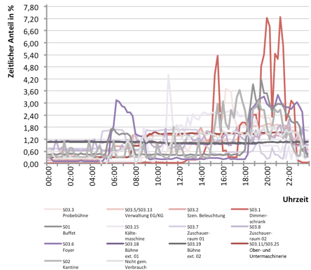
Abb. 308 Tageslastverlauf der einzelnen Stromkreise für Typtag 02_SWoV
