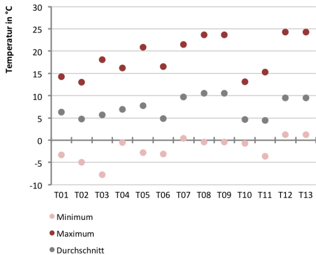
Abb. 42 Außenlufttemperatur am Standort der Theaterspielstätten während des Messzeitraums
