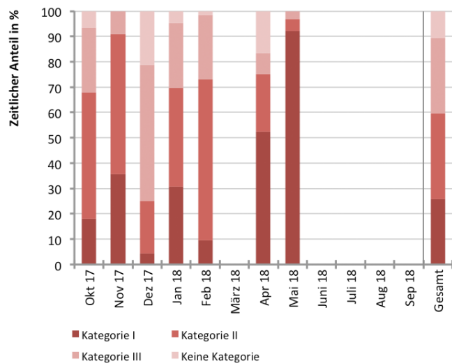
Abb. 375 Kategorisierung der Lufttemperatur während des Messzeitraums im Zuschauersaal
