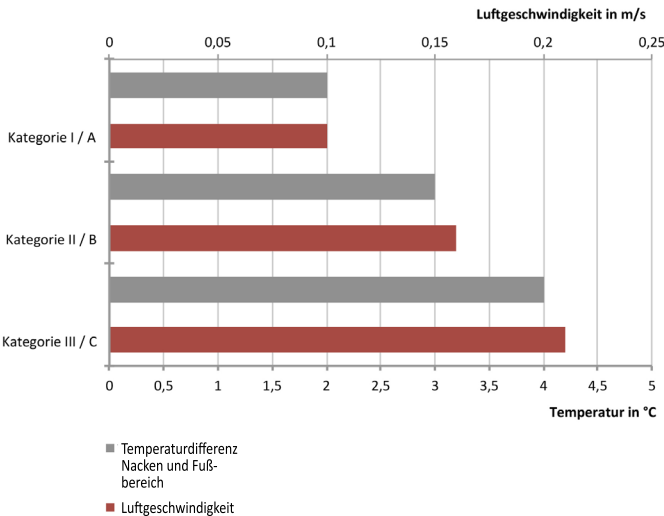
Abb. 124 Anforderungsbereiche für Zugluft und Vertikale Temperaturunterschiede nach den Kategorien
