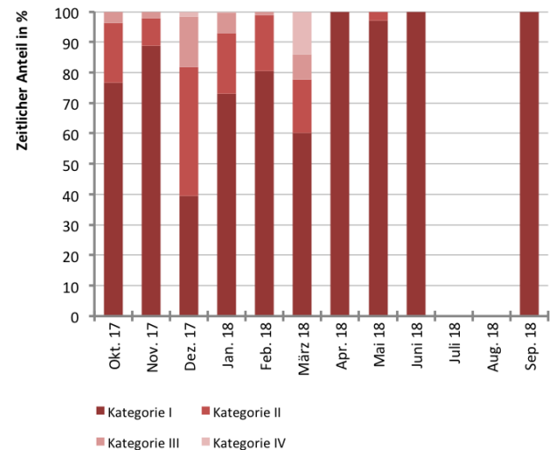
Abb. 419 Kategorisierung der \text{CO}_2 -Konzentration in der Garderobe
