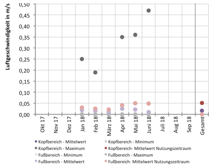
Abb. 392 Luftgeschwindigkeit im Kopf- und Fußbereich während des Messzeitraums im Rang des Zuschauersaals
