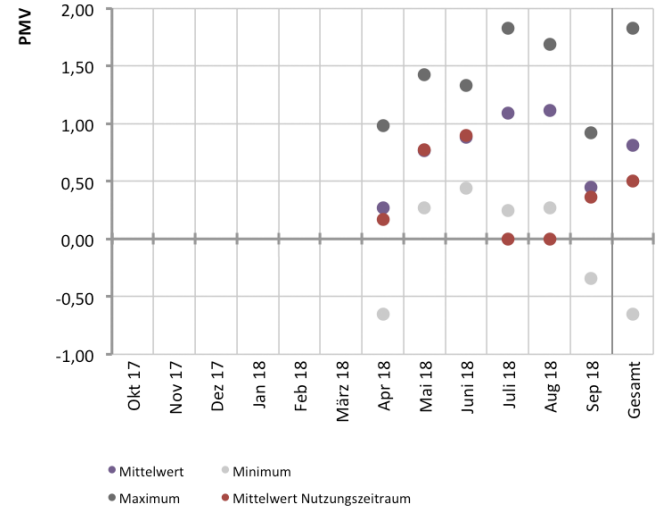
Abb. 405 Durchschnittliches PMV während des Messzeitraums im Foyer
