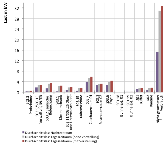
Abb. 287 Durchschnittslasten zu verschiedenen Tageszeiträumen für die einzelnen Stromkreise
