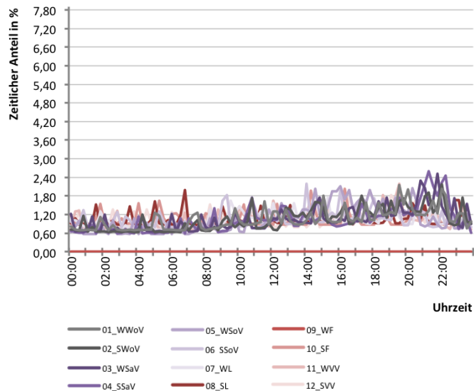
Abb. 319 Tageslastverlaufs verschiedener Typtage für S03.8 Zuschauerraum 02
