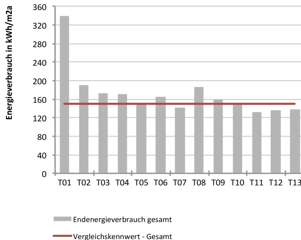
Abb. 88 Gesamtendenergieverbrauchskennwerte gegenüber des Vergleichskennwerts
