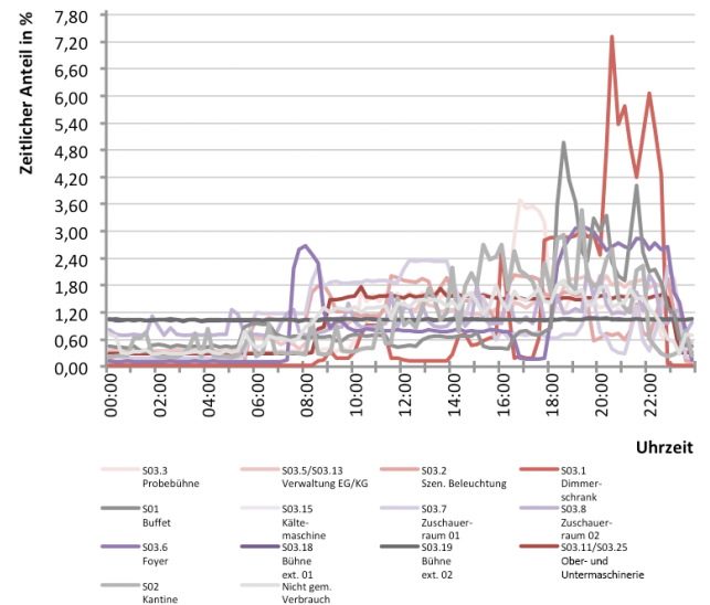
Abb. 310 Tageslastverlaufs der einzelnen Stromkreise für Typtag 01_WWoV
