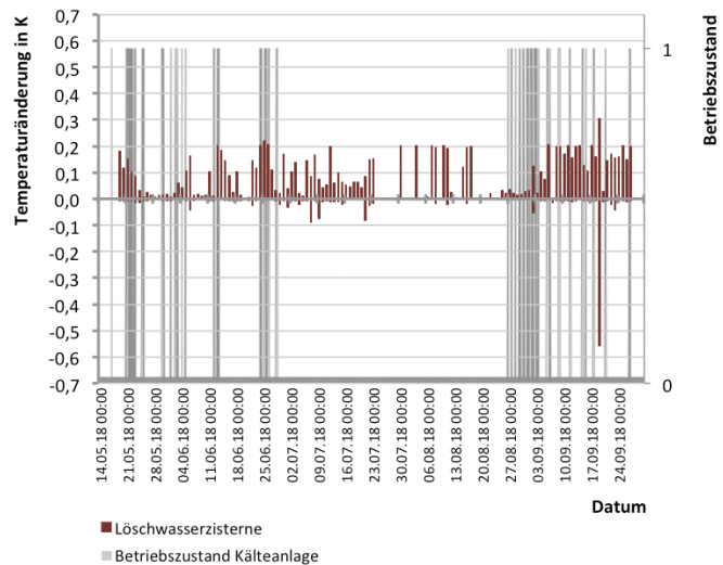
Abb. 346 Anlagenzustands gegenüber der Temperaturänderung in der Löschwasserzisterne
