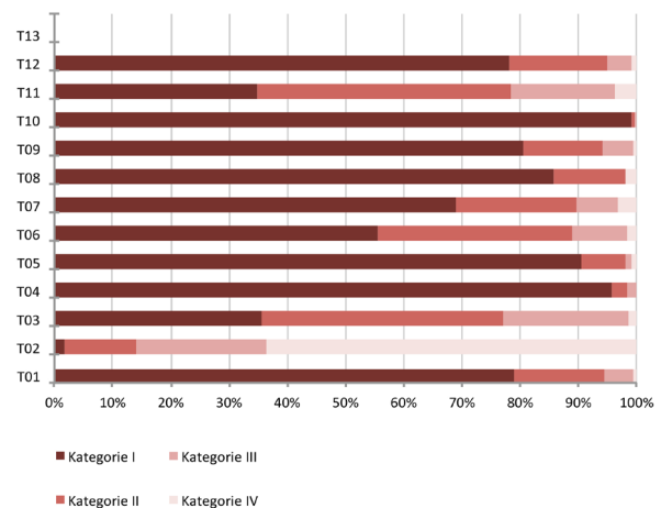
Abb. 146 Kategorisierung der Luftgeschwindigkeiten anhand der Beispiele für Gestaltungskriterien aus DIN EN ISO 7730 für den Raumtyp „Auditorium“
