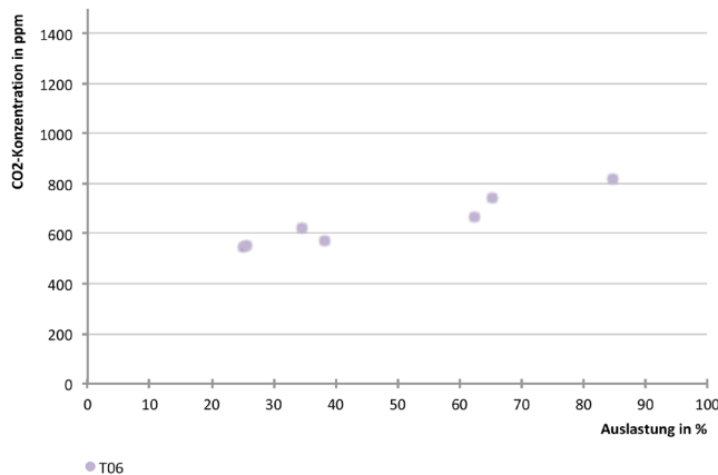
Abb. 129 Theaterspielstätten mit einem starken linearen Zusammenhang zwischen \text{CO}_2 -Konzentration und Auslastung
