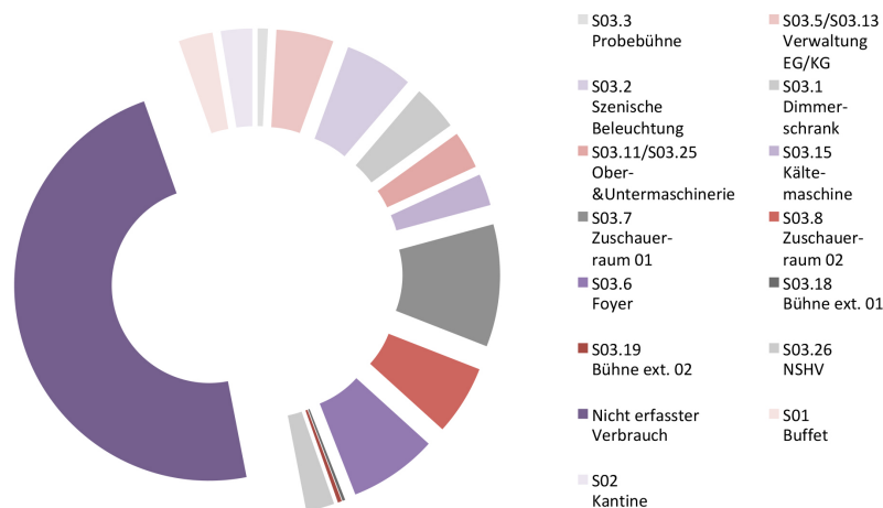
Abb. 266 Jährliche Zusammensetzung des Stromverbrauchs nach Stromkreisen
