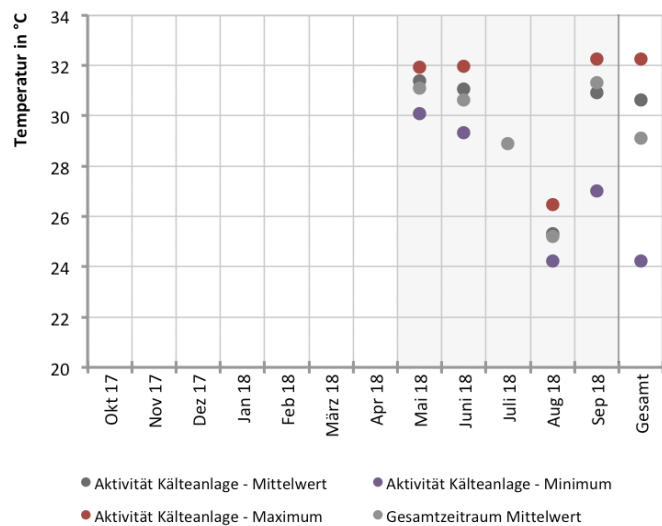
Abb. 343 Monatliche Minimal-, Maximal- und Durchschnittstemperaturen in der Löschwasserzisterne
