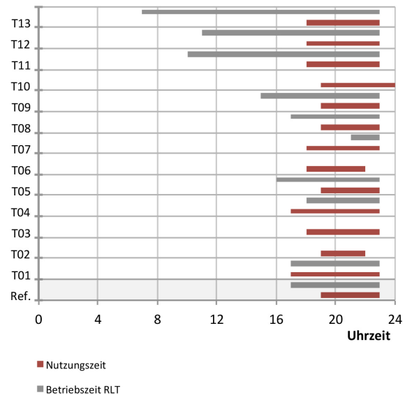
Abb. 204 Nutzungs- und Betriebszeiten der RLT-Anlagen für das Theater-Foyer
