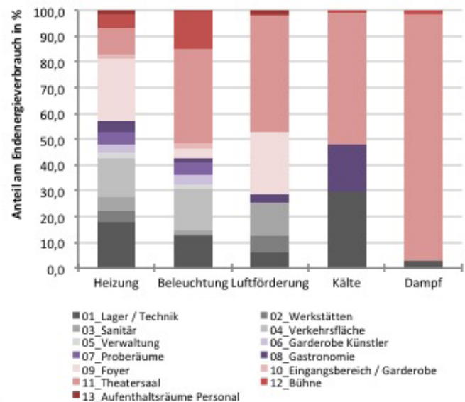
Abb. 363 Anteil der Zonen am Endenergiebedarf der größten Verbraucher
