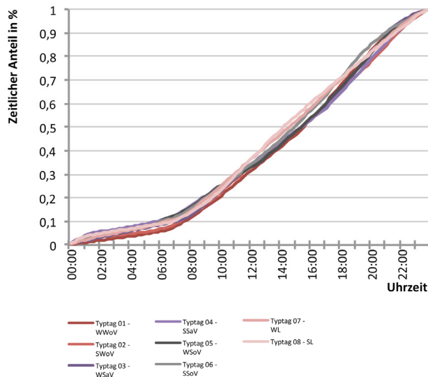
Abb. 63 Kumulativer Energieverbrauch in Abhängigkeit der Typtage
