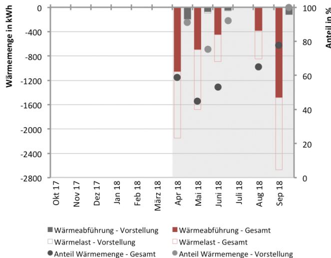
Abb. 337 Monatliche durch Lüftung abgeführten Wärmemenge im Verhältnis zu den Wärmelasten
