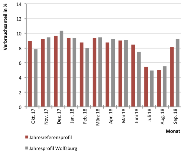
Abb. 262 Jahresreferenzprofils der Querschnittserhebung gegenüber dem Jahresstromverbrauch des Scharoun Theaters
