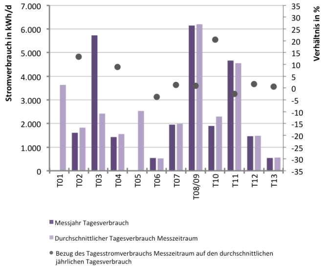
Abb. 76 Durchschnittliche Tagesstromverbräuche im Messzeitraum gegenüber der des Jahresdurchschnitts
