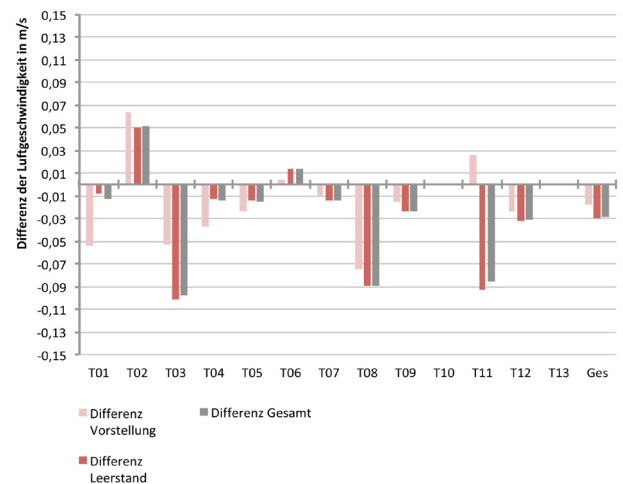
Abb. 144 Differenz von Luftgeschwindigkeit im Kopf- und Fußbereich in Abhängigkeit des Nutzungszustands
