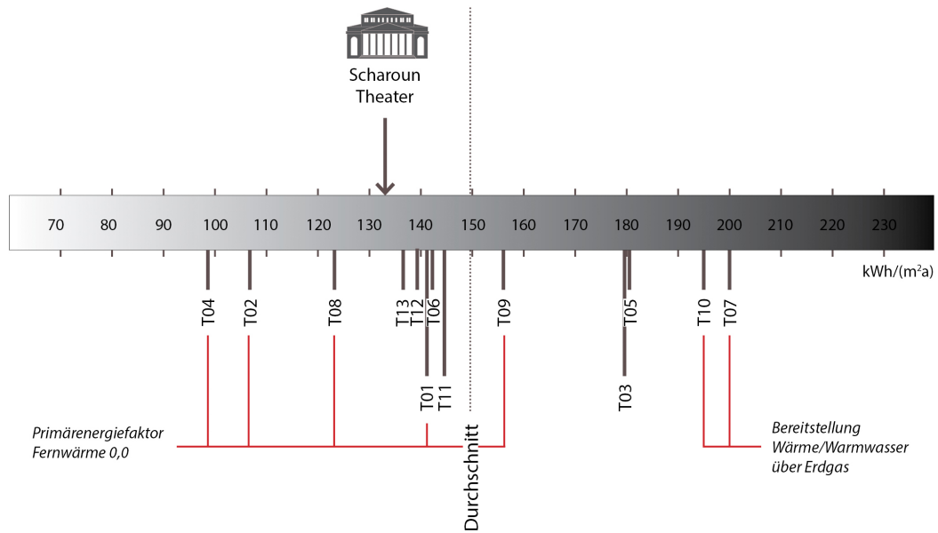
Abb. 358 Einordnung des Scharoun Theaters in das Benchmarking zum flächenbezogenen Primärenergieverbrauch
