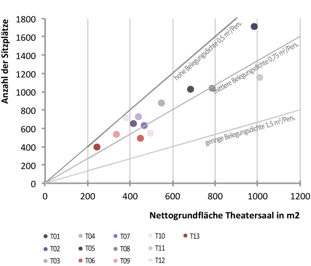
Abb. 201 Belegungsdichte in den Theaterspielstätten für den Zuschauerbereich
