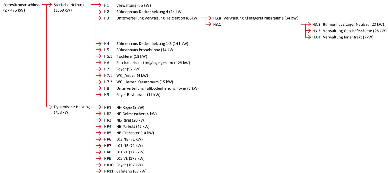
Abb. 230 Heizungsverteilung
