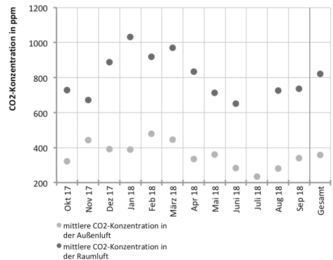
Abb. 407 Zusammenhang zwischen der CO 2 -Konzentration in der Raum- und der Außenluft im beispielhaften Büroraum
