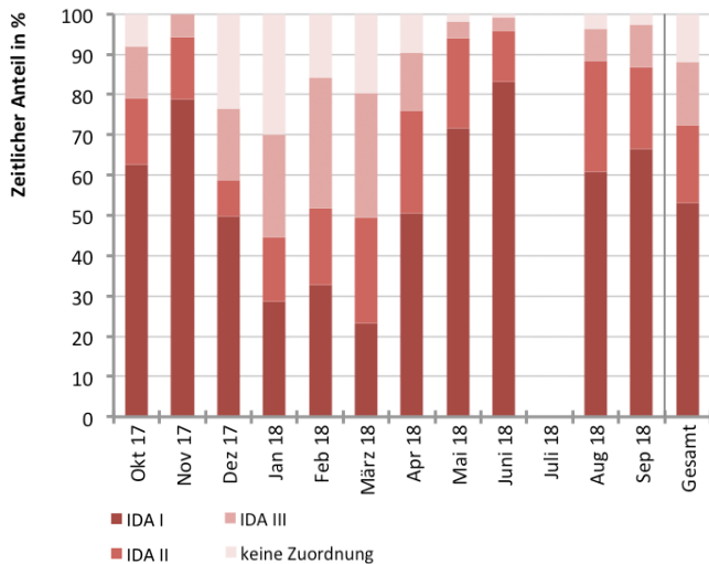
Abb. 409 Kategorisierung der Raumluftqualität anhand der CO 2 -Konzentration im beispielhaften Büroraum
