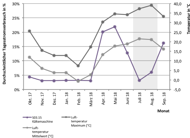
Abb. 269 Monatsstromverbrauchsanteile für S03.15 Kältemaschine gegenüber der Außenlufttemperatur
