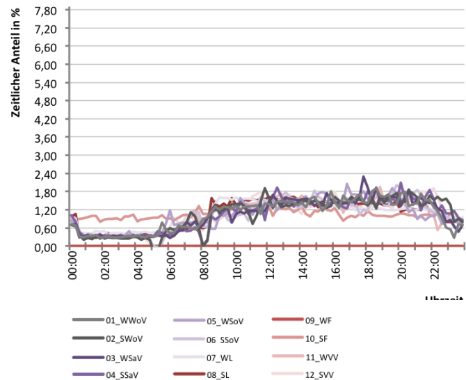
Abb. 315 Tageslastverlaufs verschiedener Typtage für den „Nicht gemessenen Verbrauch“
