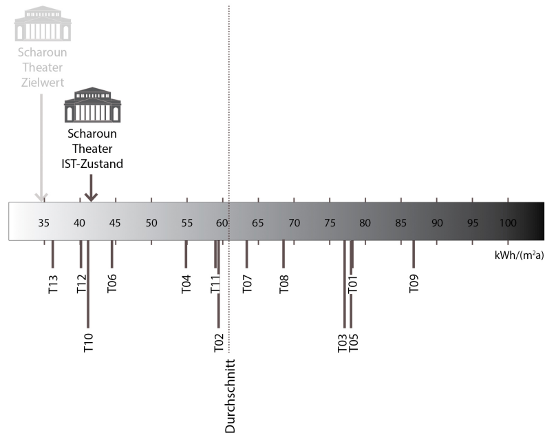
Abb. 352 Einordnung des Scharoun Theaters in das Benchmarking zum flächenbezogenen Stromverbrauch
