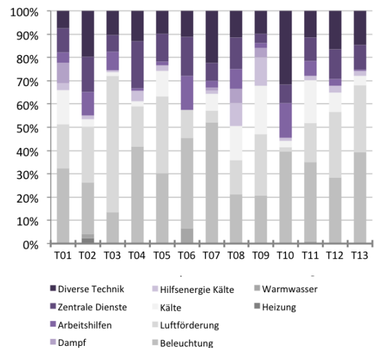
Abb. 109 Anteile der Verbraucher am Bedarf für elektrische Energie
