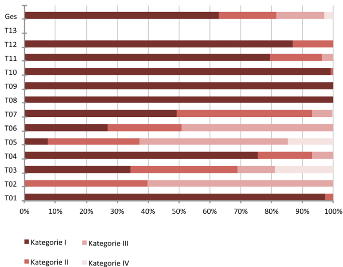
Abb. 152 Einordnung der Messwerte zur relativen Luftfeuchte in die Komfortkategorien
