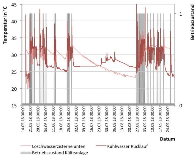
Abb. 347 Anlagenzustand gegenüber der Rücklauftemperatur sowie der Temperatur im unteren Bereich der Löschwasserzisterne
