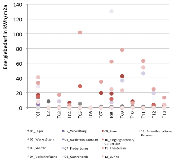
Abb. 116 Spezifischer Energiebedarf für Kälte nach Zonen
