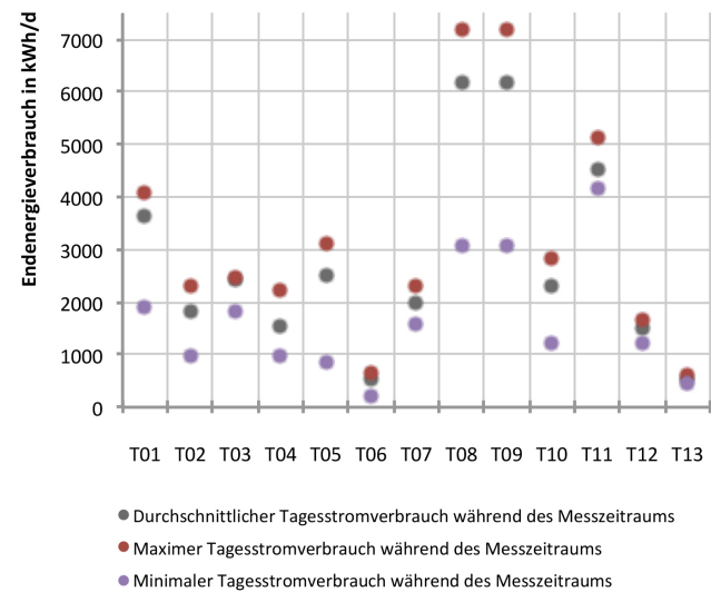
Abb. 51 Absoluter Tagesstromverbrauch während des Messzeitraums
