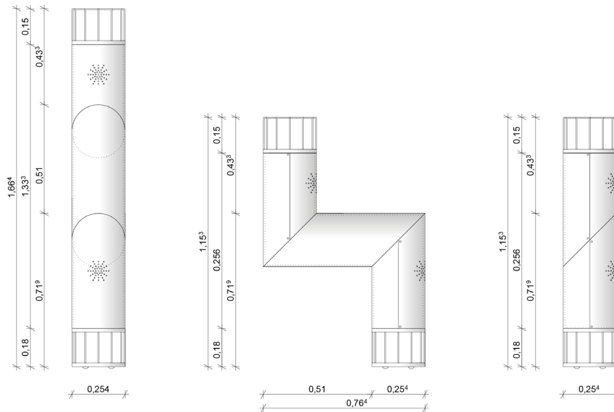
Abb. 25 Aufbaumöglichkeiten des Messtorsos
