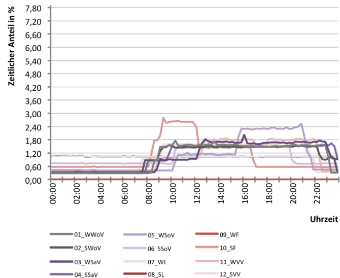
Abb. 320 Tageslastverlaufs verschiedener Typtage für S03.11/S03.25 Maschinerie
