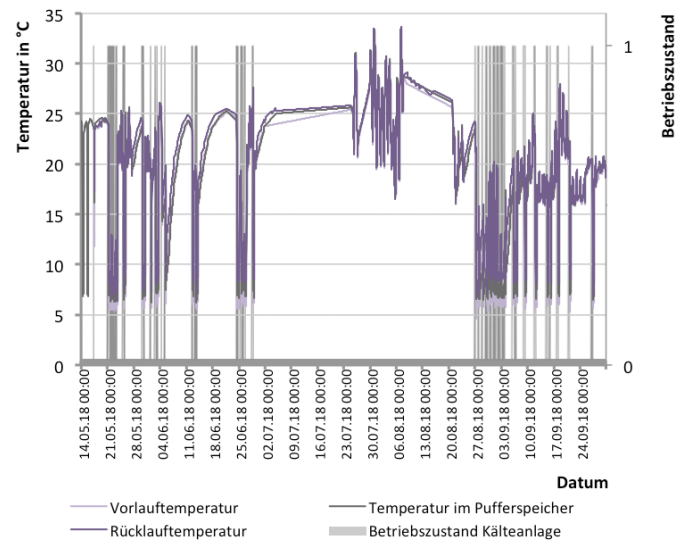
Abb. 341 Gegenüberstellung des Anlagenzustands mit den Vor- und Rücklauftemperaturen im Betrachtungszeitraum
