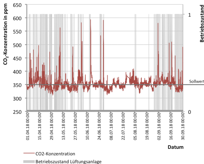
Abb. 330 \text{CO}_2 -Konzentration in der Abluft
