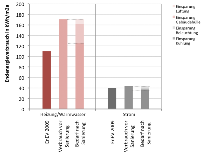
Abb. 210 Energetische Zielsetzung für das Scharoun Theater
