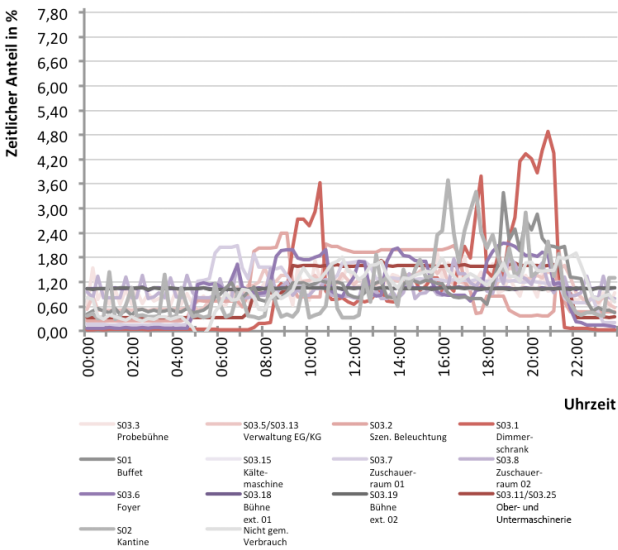
Abb. 311 Tageslastverlauf der einzelnen Stromkreise für Typtag 12_SVV
