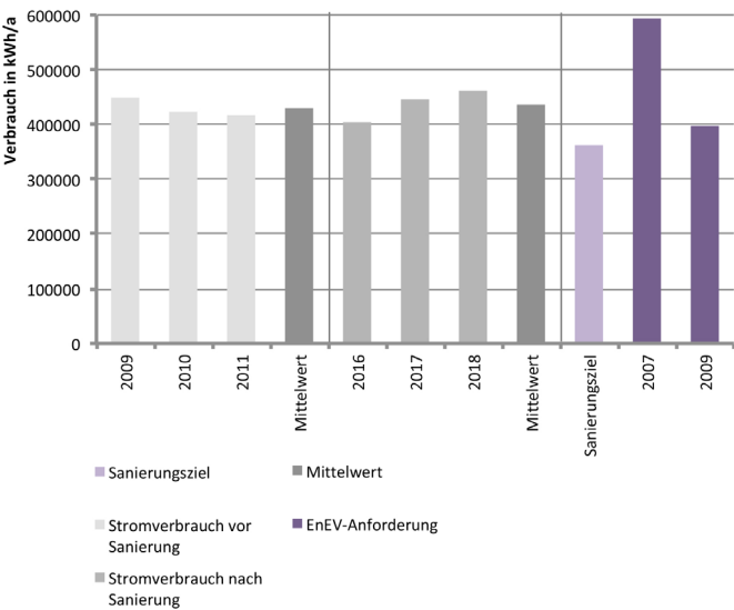
Abb. 349 Absoluter Stromverbrauch
