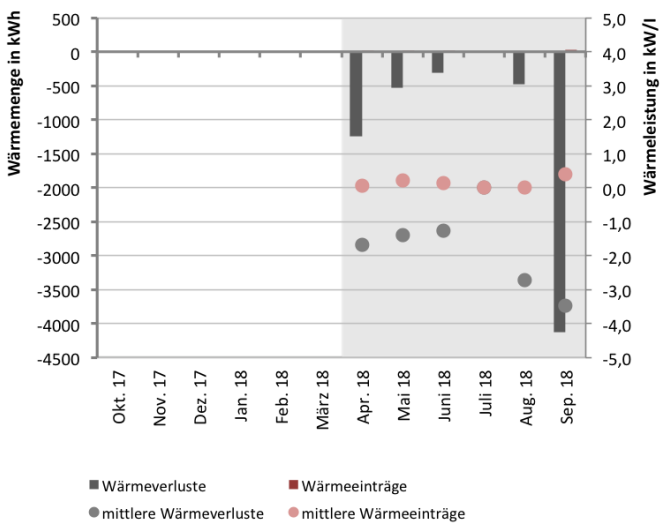
Abb. 336 Monatliche Wärmeeinträge und -verluste
