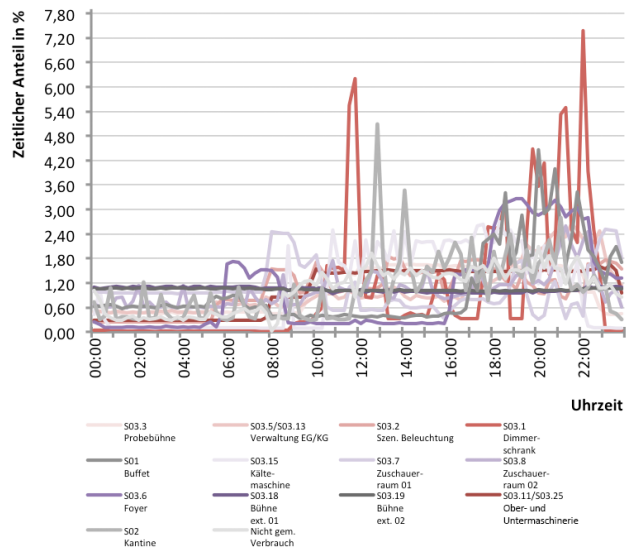
Abb. 304 Tageslastverlauf der einzelnen Stromkreise für Typtag 04_SSaV
