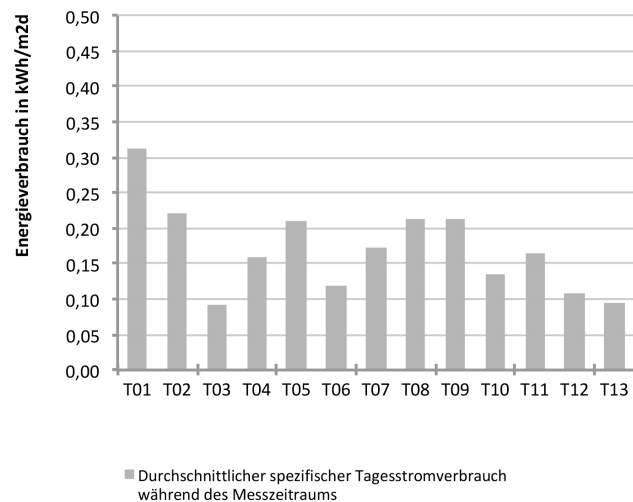
Abb. 55 Durchschnittlicher spezifischer Tagesstromverbrauch während des Messzeitraums
