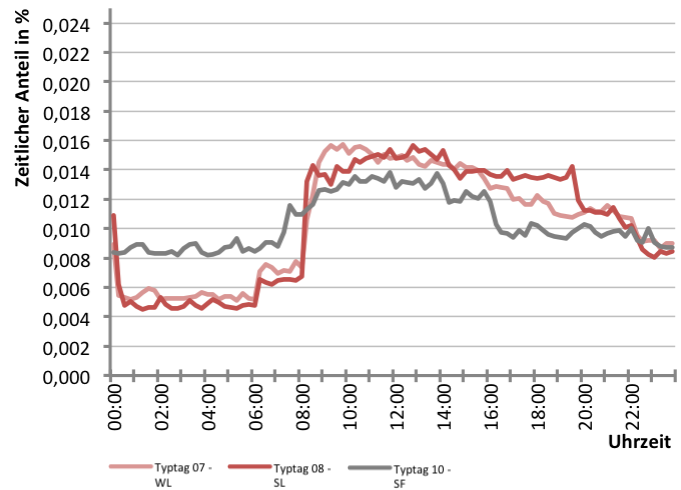
Abb. 288 Referenzlastprofil für Tage ohne Vorstellungen
