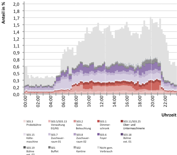
Abb. 312 Gesamter Tageslastverlauf für Typtag 12_SVV
