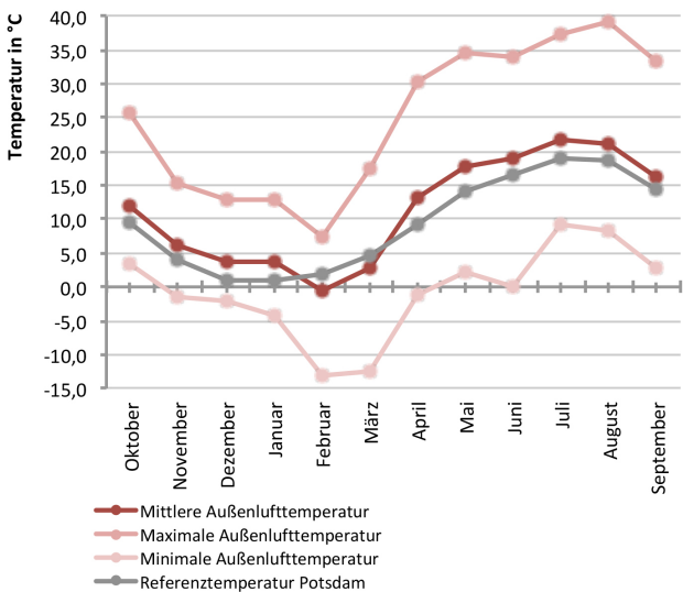
Abb. 257 Monatliche Lufttemperaturen im Messzeitraum am Standort Wolfsburg
