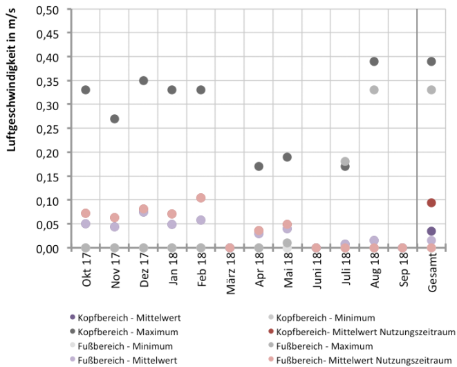
Abb. 379 Luftgeschwindigkeit im Kopf- und Fußbereich während des Messzeitraums im Zuschauersaal
