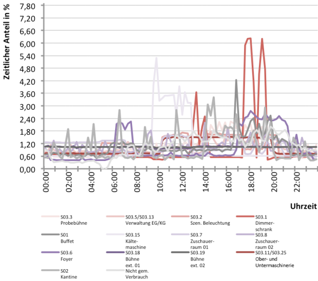
Abb. 300 Tageslastverlauf der einzelnen Stromkreise für Typtag 06_SSoV
