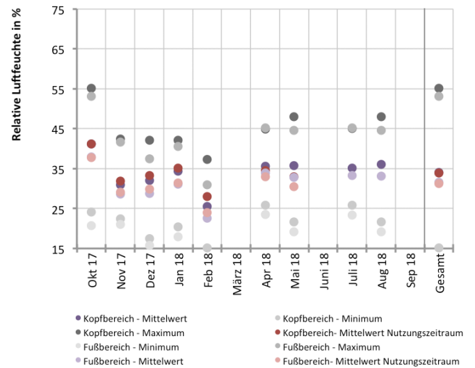
Abb. 377 Relative Luftfeuchte im Kopf- und Fußbereich während des Messzeitraums im Zuschauersaal
