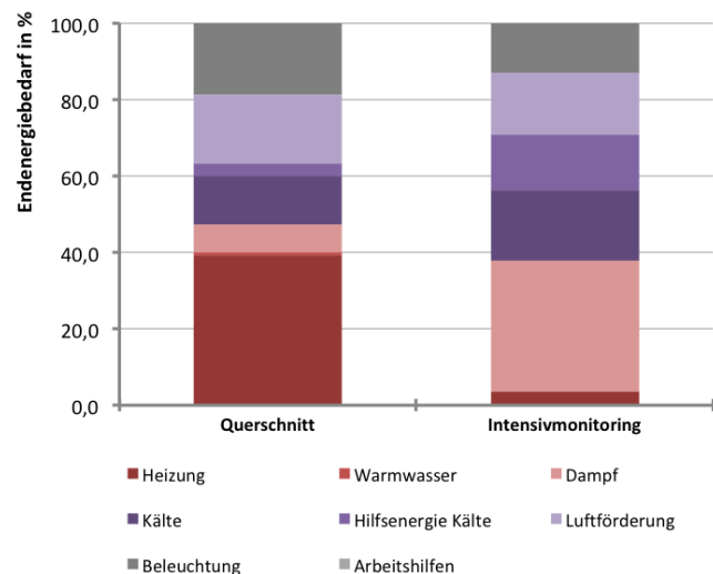
Abb. 370 Prozentualer Bedarf der einzelnen Verbraucher für die Zone 11_Theatersaal
