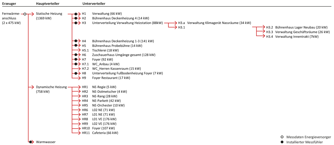
Abb. 250 Messstellen Fernwärmeverbrauch
