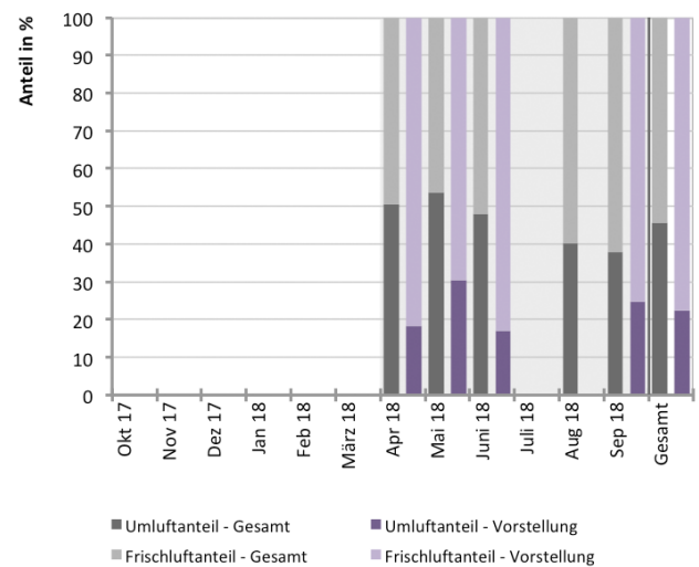
Abb. 338 Durchschnittlicher Frisch- und Umluftanteil in Abhängigkeit des Nutzungszustands
