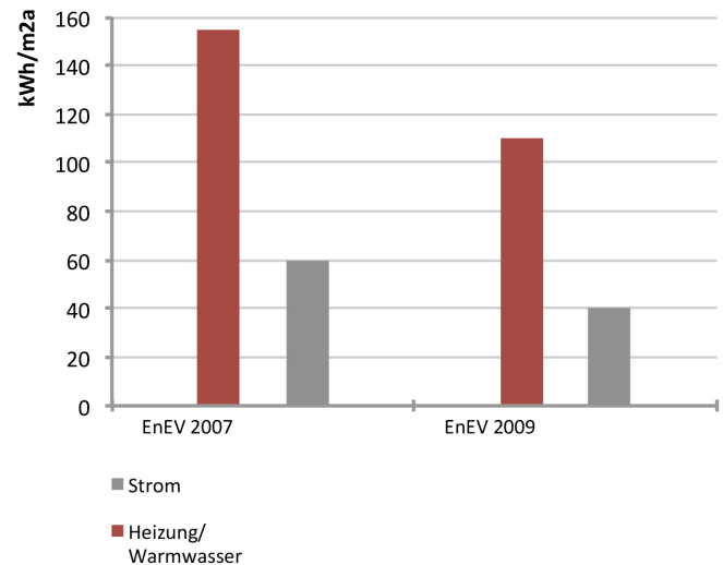
Abb. 50 Energieverbrauchskennwerte für die Nutzung „Opernhäuser, Theatergebäude“
