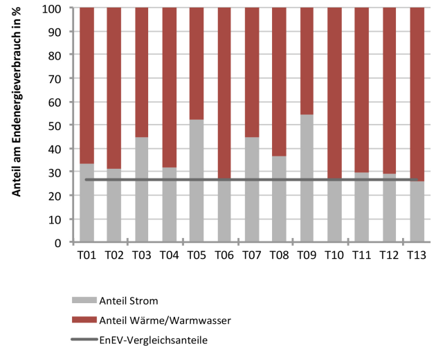
Abb. 89 Verbrauchsanteile für Strom und Heizung/Warmwasser auf endenergetischer Ebene
