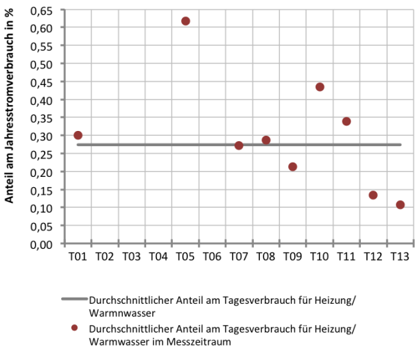
Abb. 65 Anteil des durchschnittlichen Tagesverbrauchs für Heizung/Warmwasser am Jahresverbrauch
