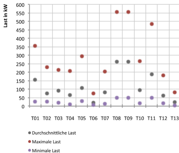
Abb. 56 Maximal-, Minimal- und Durchschnittslasten im Stromlastgang
