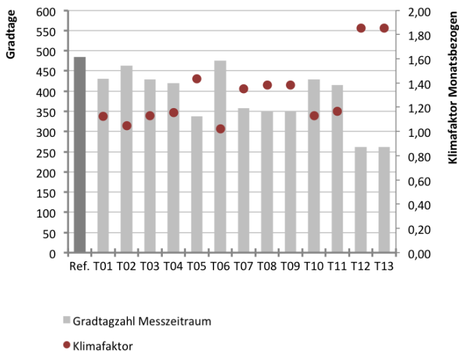
Abb. 45 Gradtage und Monatsklimafaktoren im Verhältnis zum Referenzmonat März für den Standort Potsdam
