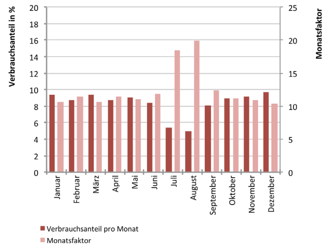
Abb. 71 Monatsprofil des Stromverbrauchs und Faktoren zur Hochrechnung des Monatsverbrauchs auf ein ganzes Jahr
