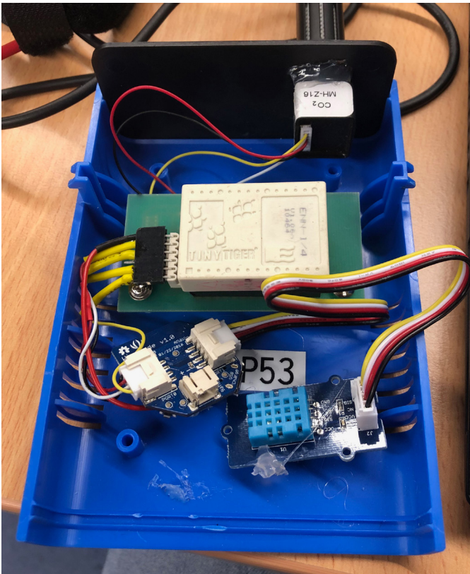
Abb. 255 Innere Struktur der Messboxen
