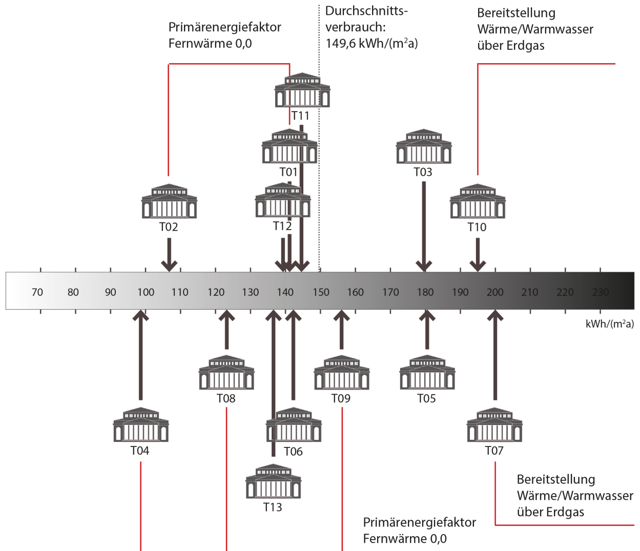
Abb. 100 Benchmarking des flächenbezogenen Gesamtverbrauchs auf primärenergetischer Ebene
