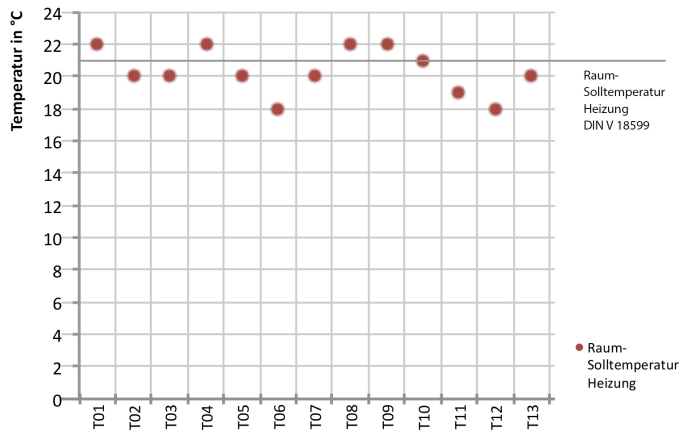
Abb. 207 Raum-Solltemperaturen im Heizfall für das Theater-Foyer
