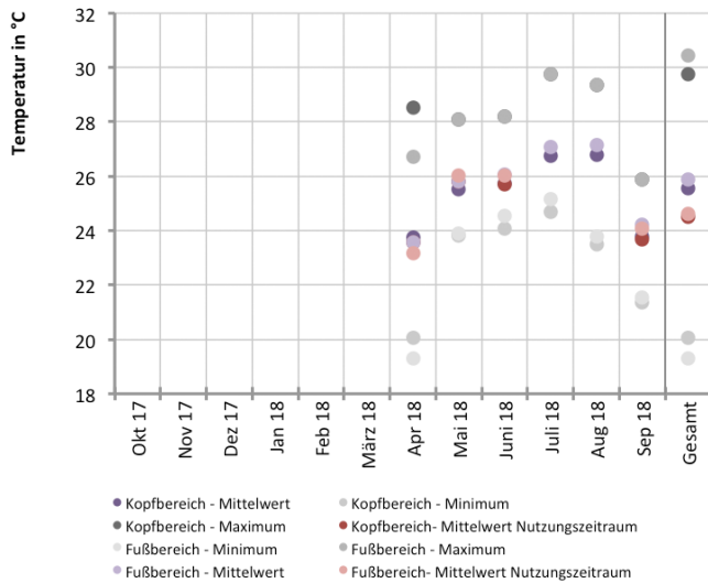
Abb. 397 Lufttemperatur des Foyers im Kopf- und Fußbereich während des Messzeitraums
