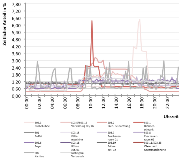
Abb. 296 Tageslastverläufe der einzelnen Stromkreise für Typtag 07_WL
