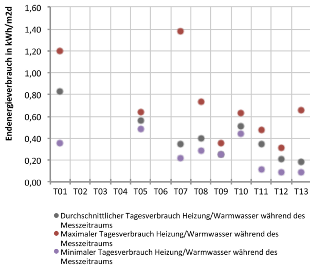
Abb. 66 Spezifischer und klimabereinigter Tagesverbrauch für Heizung/Warmwasser während des Messzeitraums
