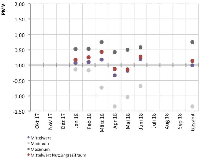
Abb. 395 Durchschnittliches PMV während des Messzeitraums im Rang des Zuschauersaals
