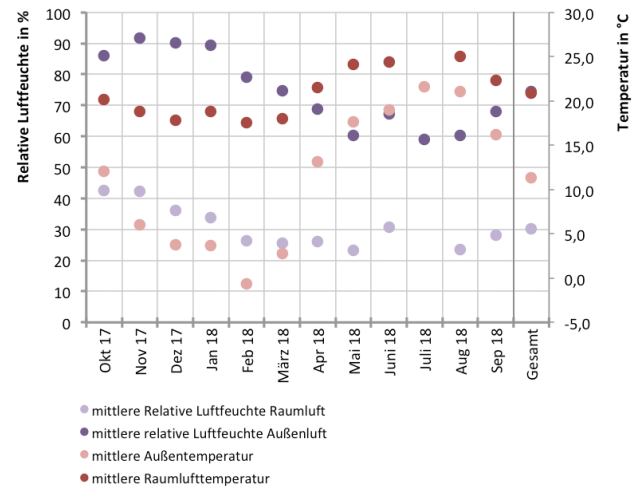
Abb. 411 Zusammenhang zwischen relativer Luftfeuchte und Temperatur der Raum- und Außenluft im beispielhaften Büroraum
