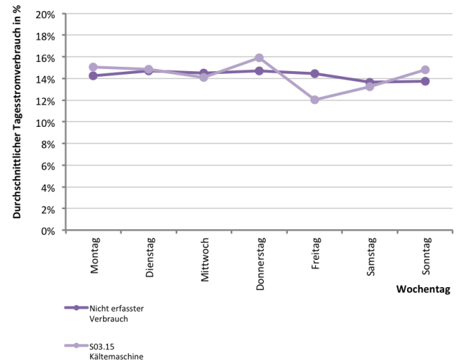
Abb. 278 Wochenstromverbrauchsanteil für S03.15 Kältemaschine und dem nicht erfassten Verbrauch
