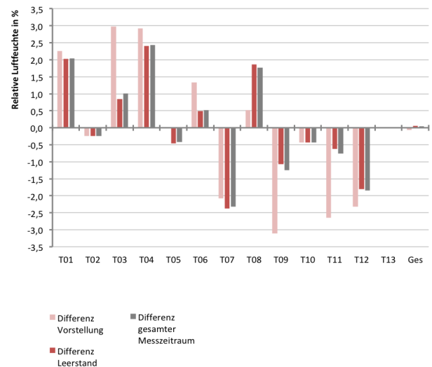
Abb. 151 Differenz der relativen Luftfeuchte zwischen Kopf- und Fußbereich nach Nutzungszustand
