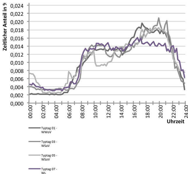
Abb. 61 Standardlastprofile für Theaterspielstätten auf Basis der Messergebnisse für den Winter
