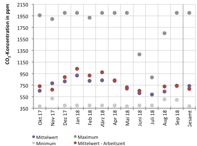
Abb. 406 CO 2 -Konzentration im beispielhaften Büroraum während des Messzeitraums
