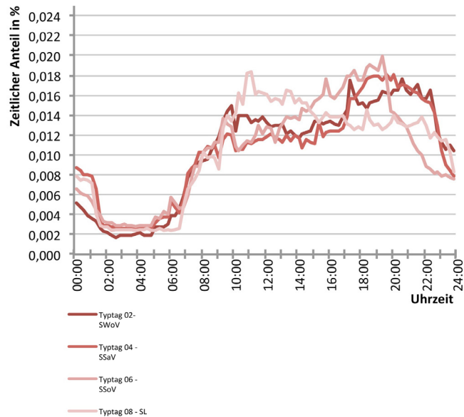
Abb. 62 Standardlastprofile für Theaterspielstätten auf Basis der Messergebnisse für den Sommer
