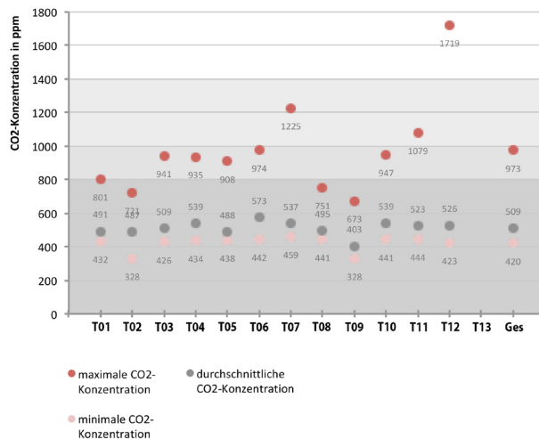
Abb. 125 Minimale, maximale und durchschnittliche \text{CO}_2 -Konzentrationen in den Theaterspielstätten
