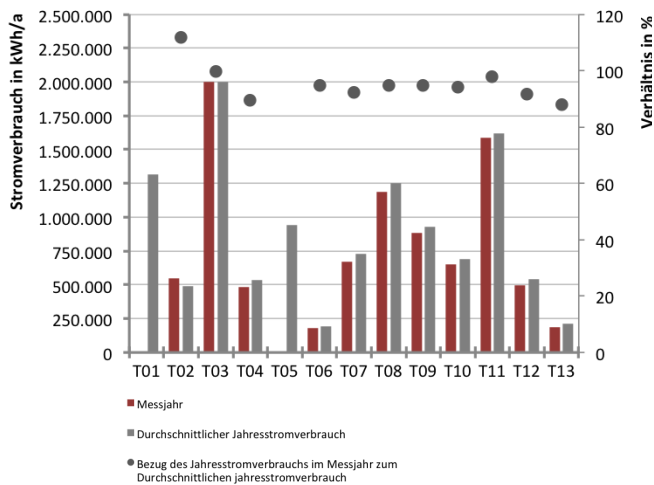
Abb. 69 Stromverbrauch im Messjahr gegenüber des durchschnittlichen Jahresstromverbrauchs
