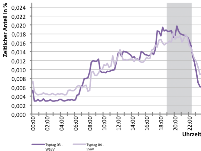
Abb. 291 Referenzlastprofil für Tage mit Vorstellungen an Samstagen
