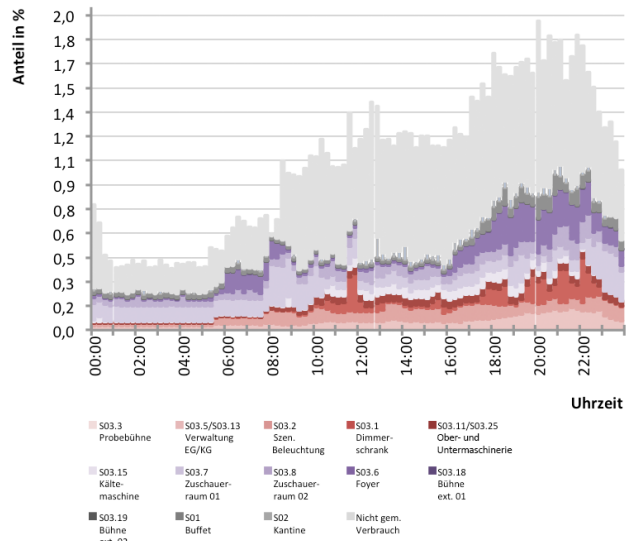
Abb. 303 Gesamter Tageslastverlauf für Typtag 04_SSaV
