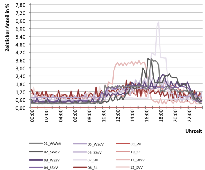
Abb. 328 Tageslastverlaufs verschiedener Typtage für S03.3 Probebühne
