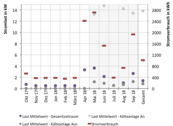
Abb. 339 Monatlicher Stromverbrauch und –Lasten nach Betriebszustand der Kälteanlage
