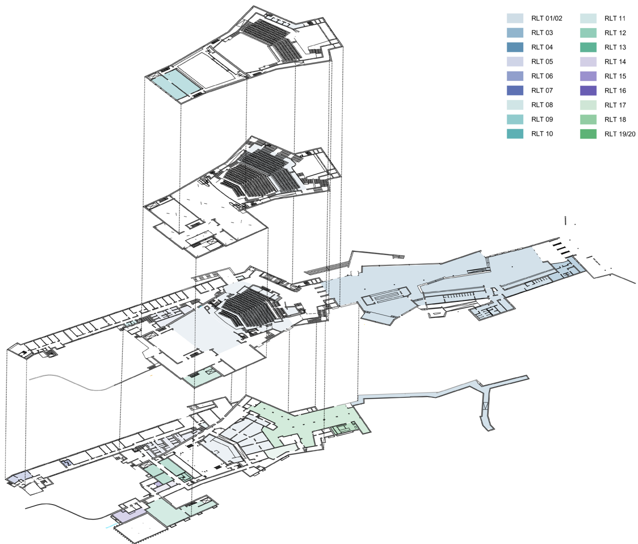
Abb. 234 Zonierung der Lüftungsanlagen
