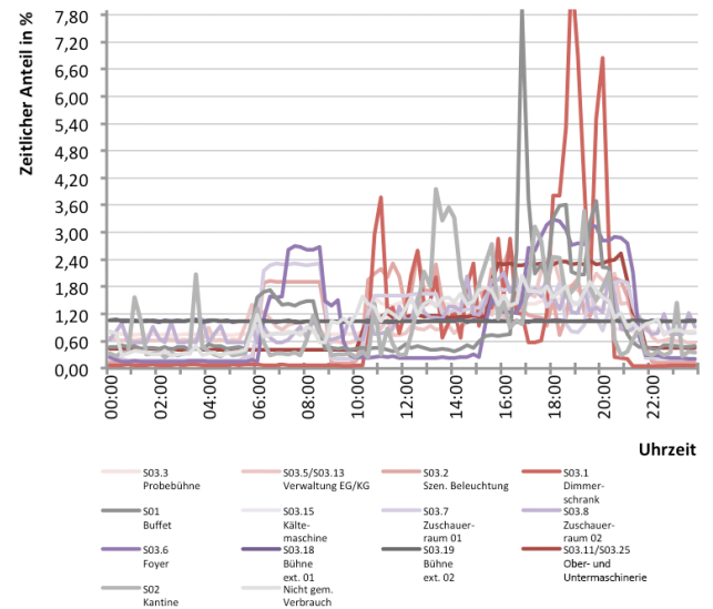
Abb. 302 Tageslastverlauf der einzelnen Stromkreise für Typtag 05_WSoV
