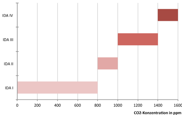
Abb. 120 Darstellung Raumluftklassen (IDA)
