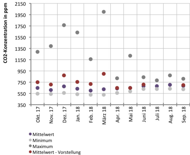
Abb. 416 CO 2 -Konzentration in der Raumlufth der Garderobe während des Messzeitraums
