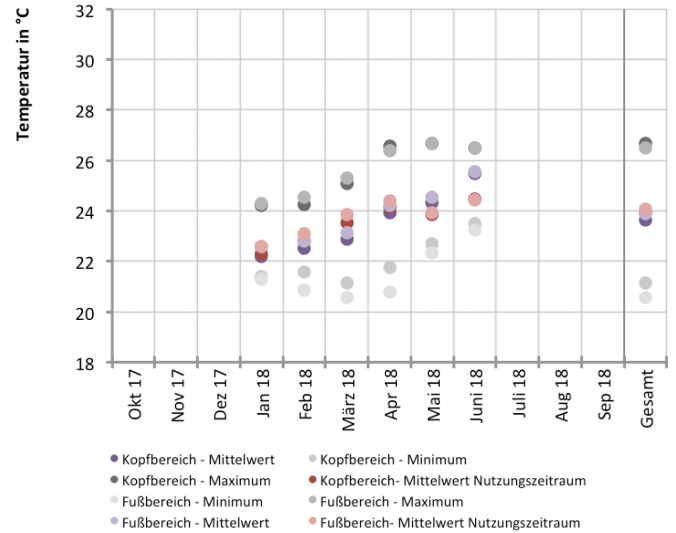
Abb. 386 Lufttemperatur im Kopf- und Fußbereich während des Messzeitraums im Rang des Zuschauersaals
