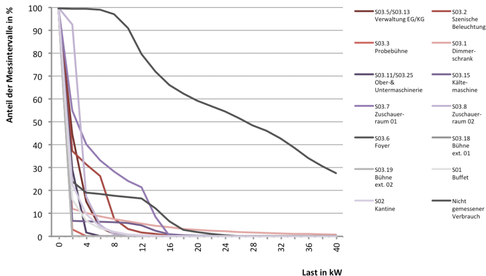
Abb. 285 Summenhäufigkeit von Lasten in den einzelnen Stromkreisen
