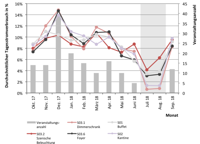
Abb. 270 Monatsstromverbrauchsanteile gegenüber der Veranstaltungsanzahl
