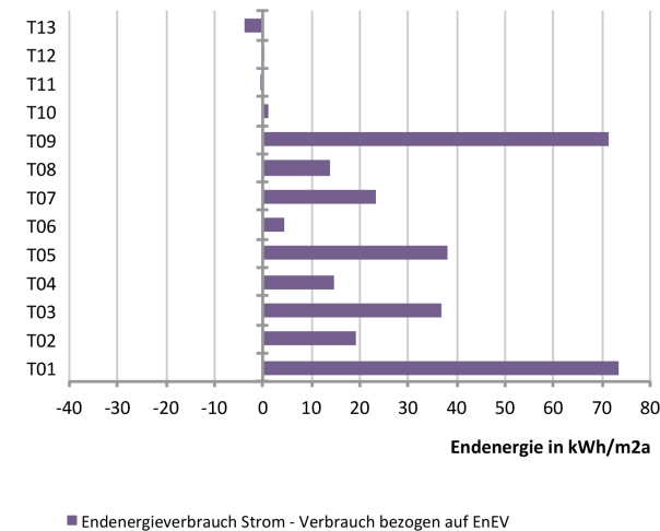
Abb. 86 Endenergieverbrauchskennwerte für Strom gegenüber des Vergleichskennwerts
