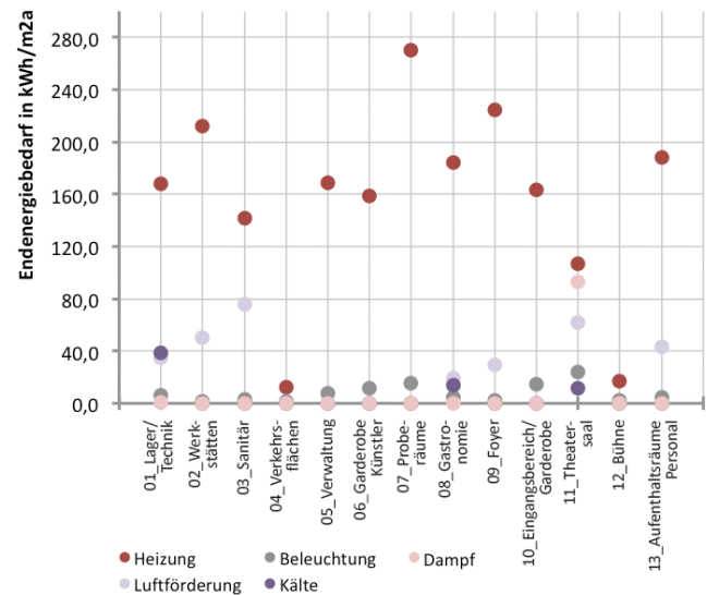
Abb. 364 Spezifischer Endenergiebedarf der einzelnen Zonen bezogen auf die größten Verbraucher
