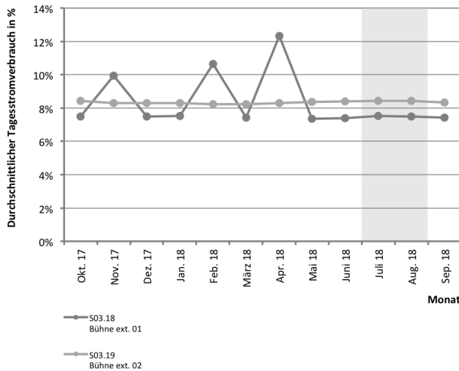
Abb. 272 Monatsstromverbrauchsanteile für die Bespielung der Bühne
