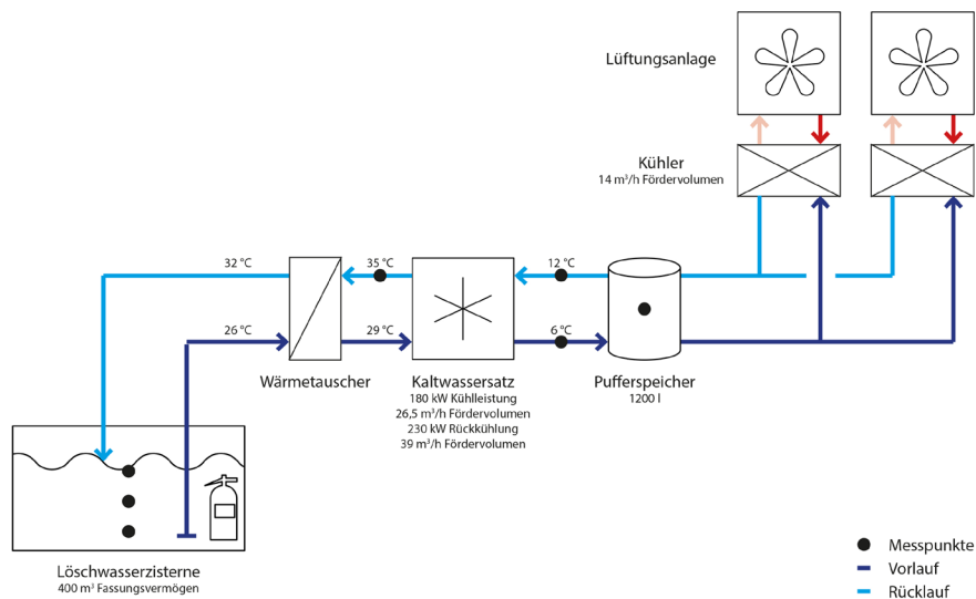
Abb. 340 Schema der Kälteanlage mit Eintragung der Messpunkte
