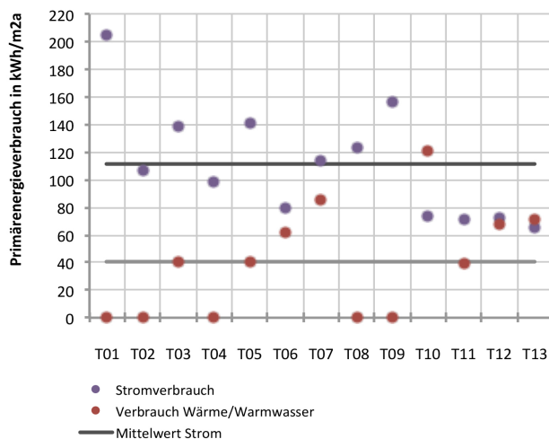
Abb. 91 Primärenergieverbrauchskennwerte für Strom und Heizung/Warmwasser
