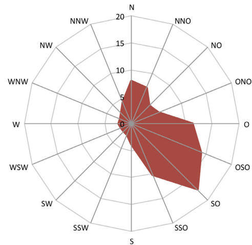
Abb. 261 Häufigkeit der Windrichtung während des Messzeitraums am Standort Wolfsburg
