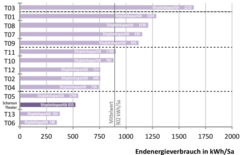
Abb. 353 Einordnung des Scharoun Theaters in das Benchmarking zum sitzplatzbezogenen Stromverbrauch
