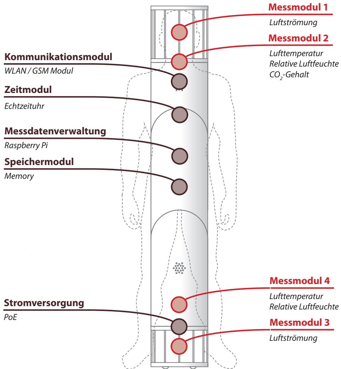
Abb. 27 Schematische Darstellung des technischen Konzepts des Messtorsos
