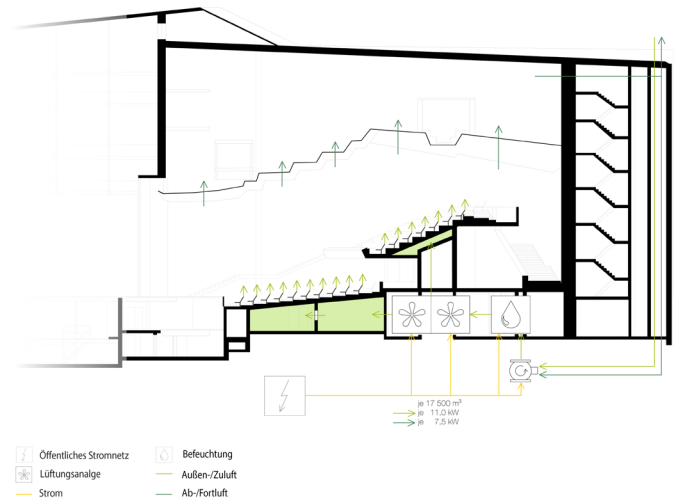
Abb. 235 Abb. 229 Funktionsschema der Lüftungsanlage „01/02 Zuschauersaal“
