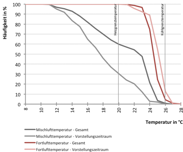
Abb. 333 Summenhäufigkeit für Misch- und Fortlufttemperatur in Abhängigkeit des Nutzungszeitraums
