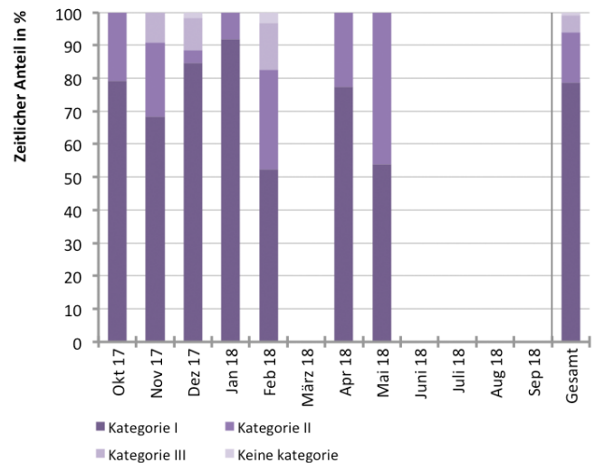
Abb. 378 Kategorisierung der Relativen Luftfeuchte während des Messzeitraums im Zuschauersaal
