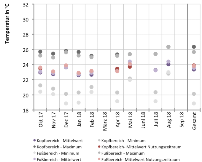
Abb. 374 Lufttemperatur im Kopf- und Fußbereich während des Messzeitraums im Zuschauersaal
