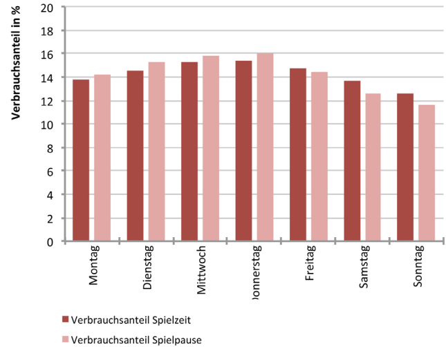
Abb. 75 Wochenprofil des Stromverbrauchs
