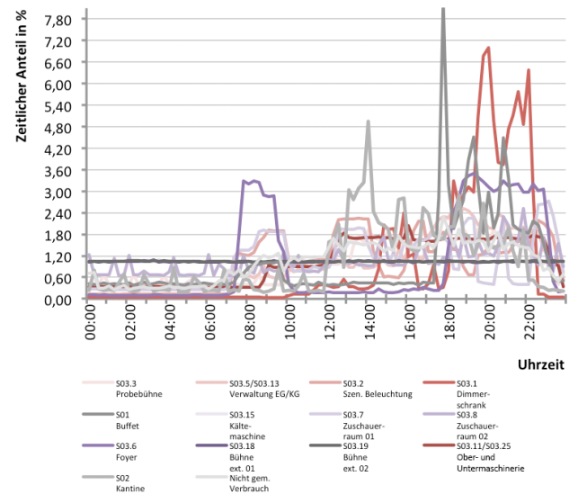
Abb. 306 Tageslastverlauf der einzelnen Stromkreise für Typtag 03_WSaV
