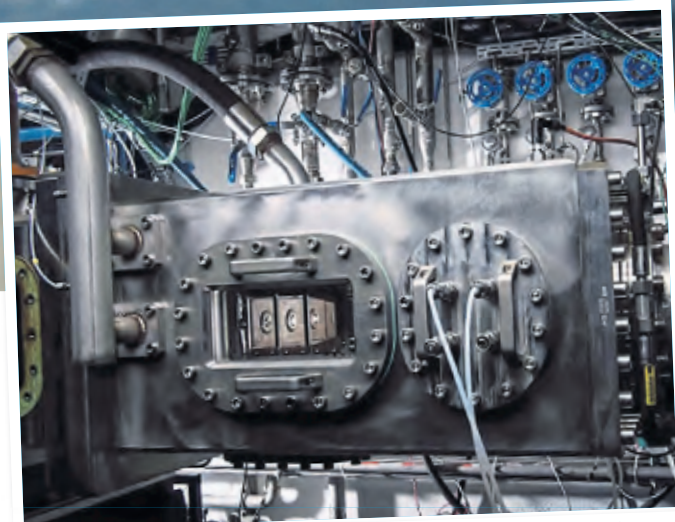
In einer Brennkammer kann die Verbrennung genau unter die Lupe genommen werden. Foto: DLR (CC BY-NC-ND 3.0)
