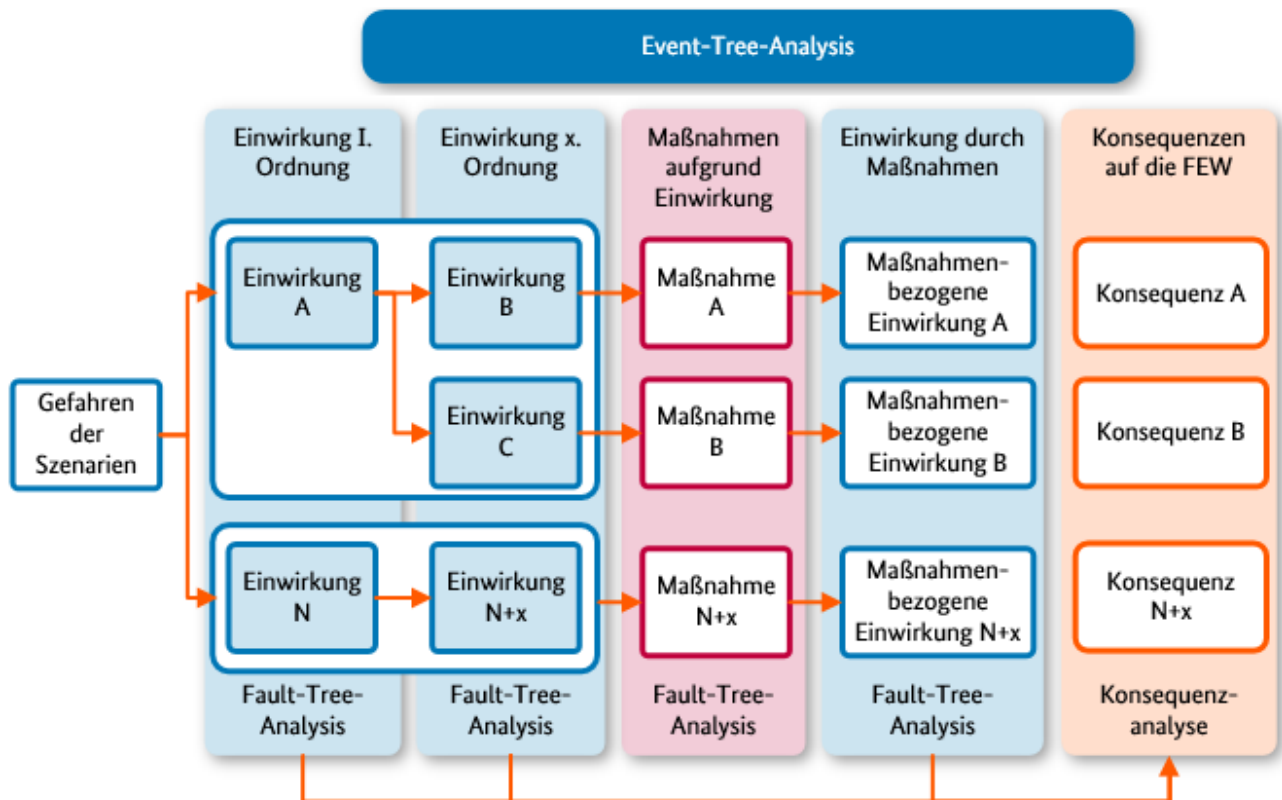
Abbildung 13: Erweiterte Event-Tree-Analyse
