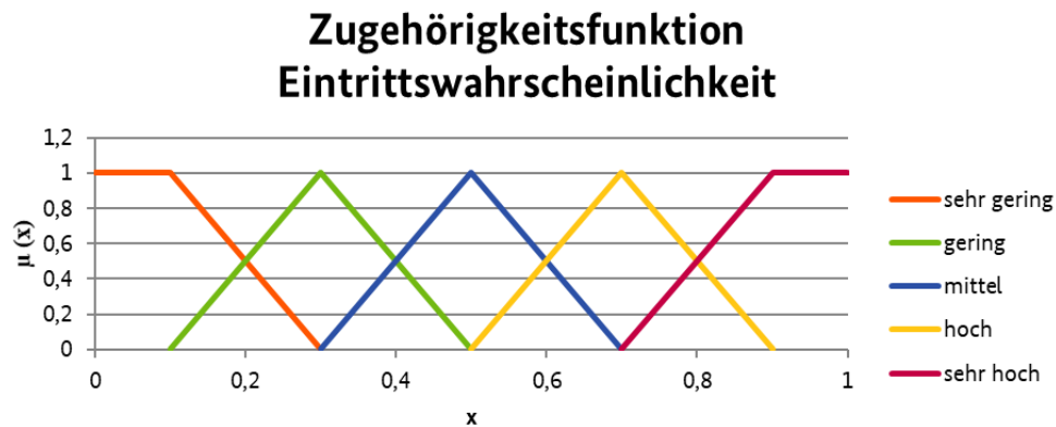
Abbildung 17: Zugehörigkeitsfunktion Eintrittswahrscheinlichkeit (Quelle: angelehnt an Society of Actuaries (2015, S. 24))
