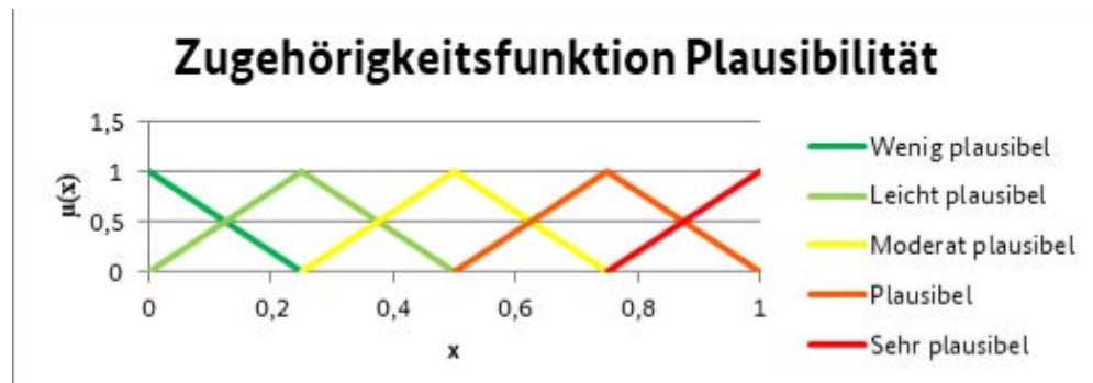
Abbildung 20: Zugehörigkeitsfunktion Plausibilität
