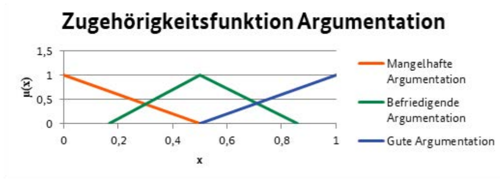
Abbildung 18: Zugehörigkeitsfunktion Argumentation (angelehnt an Tchórzewska-Cieślak (2011, S. 143))
