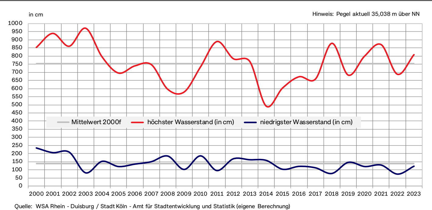
Grafik 005: Wasserstände des Rheins am Kölner Pegel (Rheinkilometer 688)
