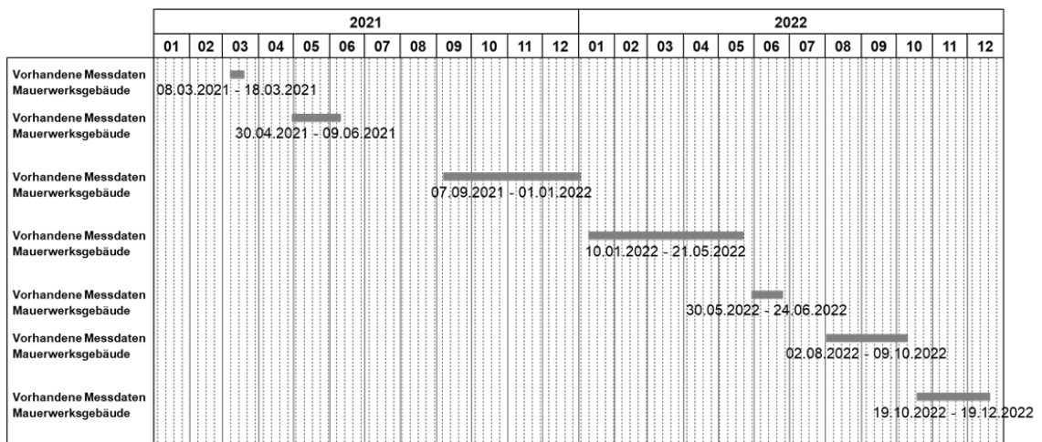
Abbildung 7: Vorhandene Messdaten für Temperatur, relative Luftfeuchte und Wärmestrom im Mauerwerksgebäude, Tinker-Forge-Messtechnik sowie Außenlufttemperatur der Wetterstation
