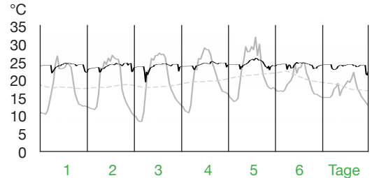
Innen- und Außenlufttemperatur, Messungen einer Augustwoche, Gebäude Holz, 2,5-Zimmer-Wohnung mit Fenstern Richtung Süden, Osten und Westen
