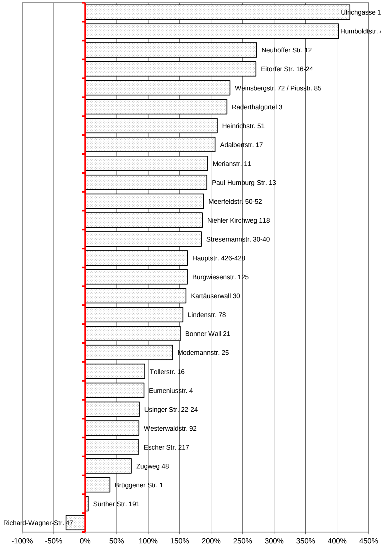
Abbildung A2.11: Berufsbildende und Gesamtschulen, Heizung
