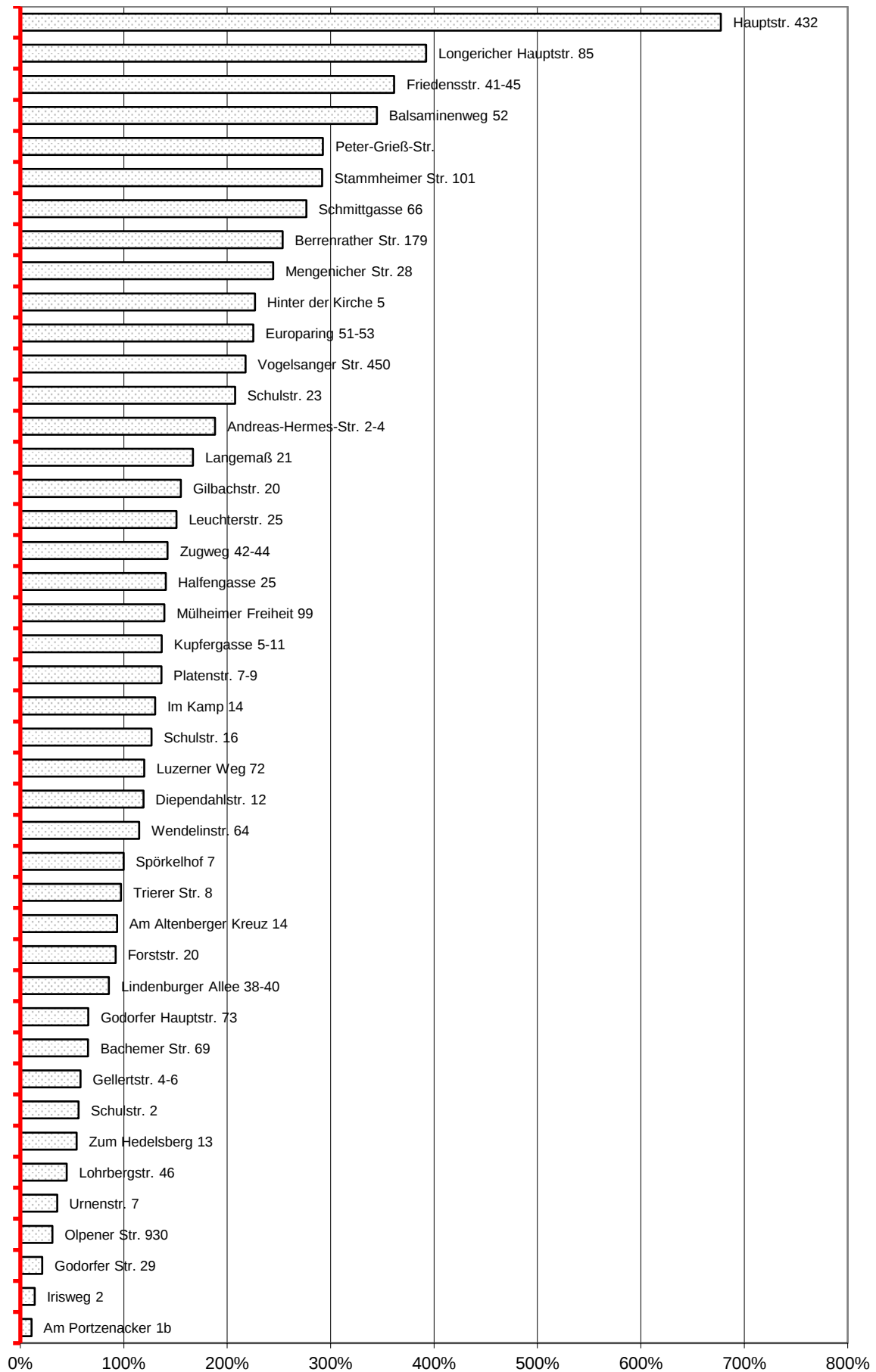
Abbildung A2.5: Grundschulen <3.500 m², Heizung
