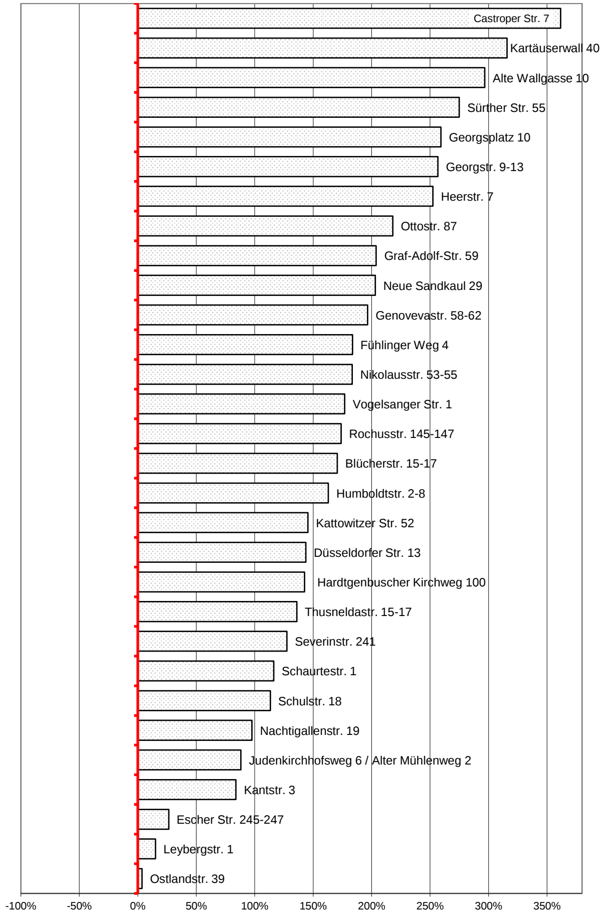
Abbildung A2.7: Gymnasien, Heizung
