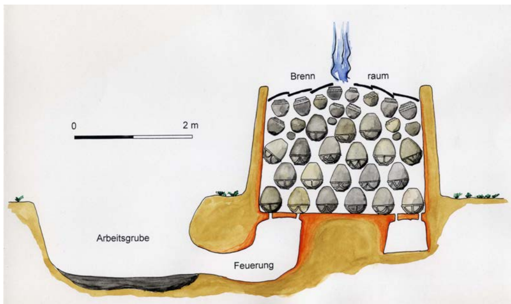
Abb. 2: Rekonstruktion eines Brennofens nach Grabungsbefunden an der Rheinldorfer Burg, Bornheim-Walberberg (nach Böhner, Bonner Jahrbuch 155/156, Abb.3)
