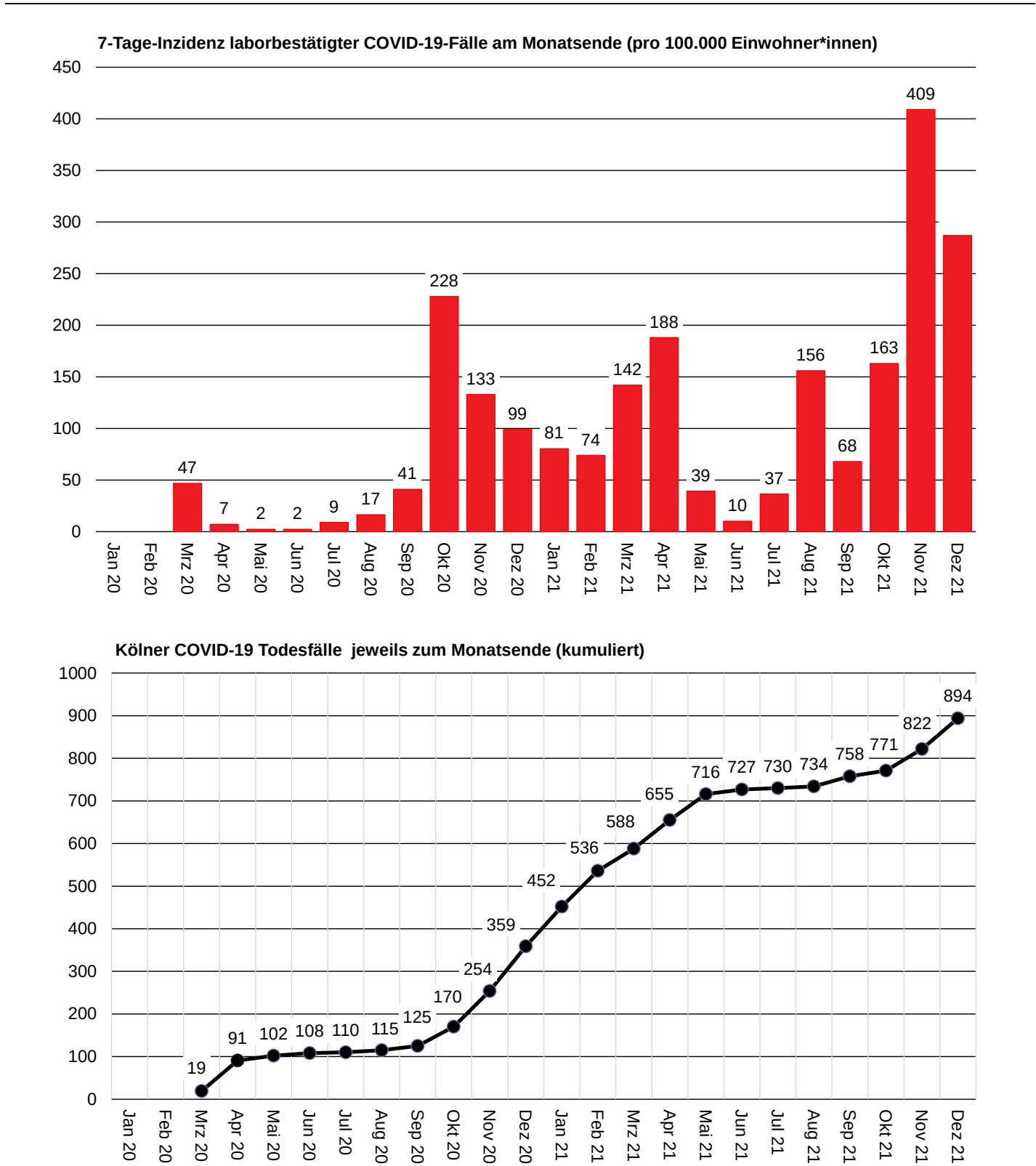
Grafik 225: 7-Tage-Inzidenz laborbestätigter COVID-19-Fälle und Kölner Todesfälle ab Januar 2020 in Köln
