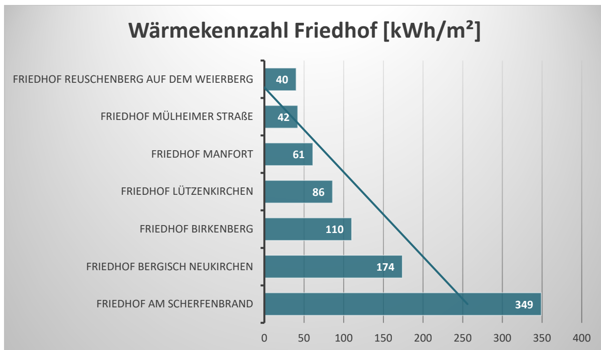
Abb. 22: Wärmekennzahl Friedhöfe 2020
