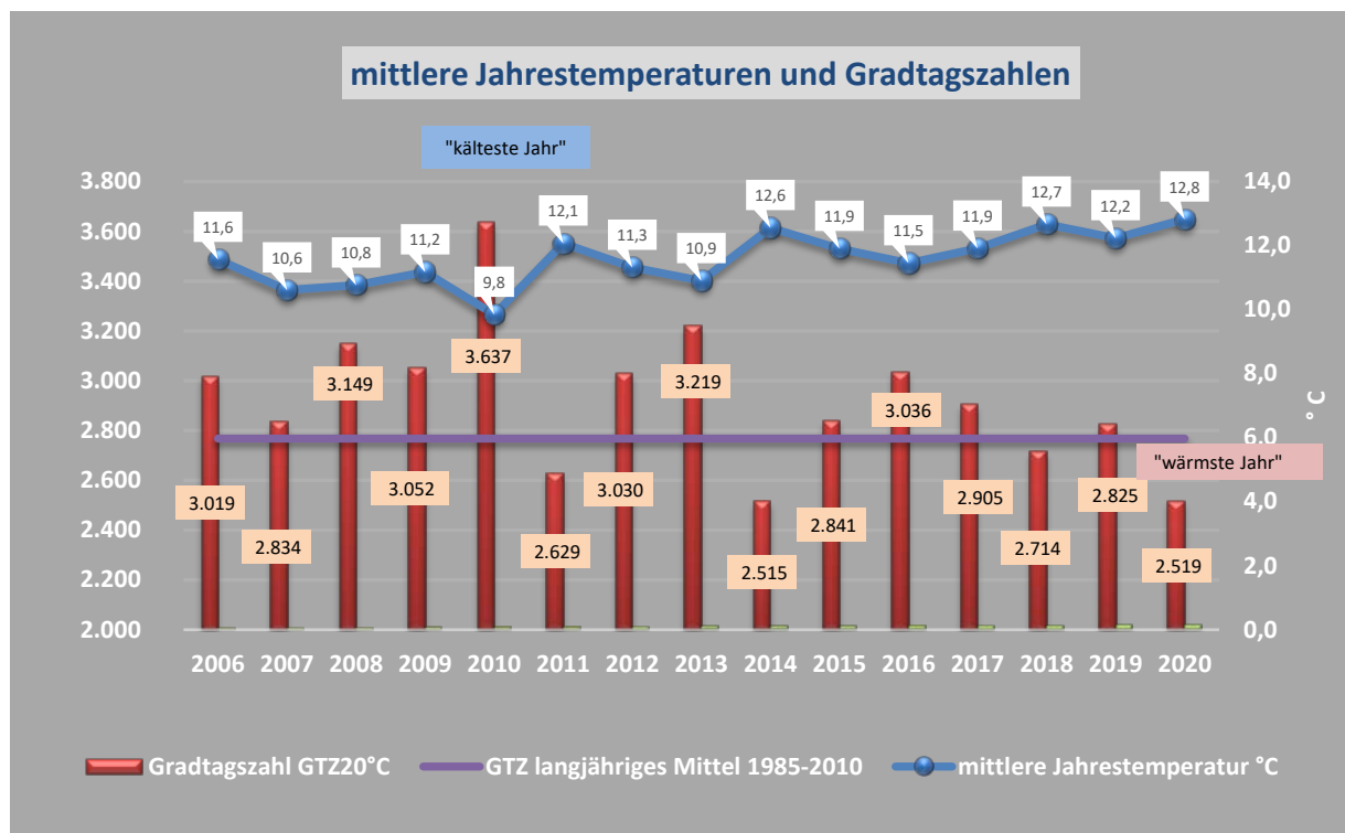
Abb. 3: mittlere Jahrestemperaturen und Gradtagszahl 2 für Leverkusen
