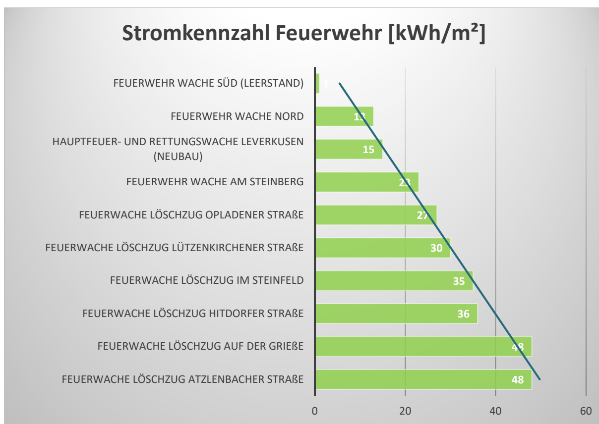
Abb. 18: Stromkennzahl Feuerwehr 2020
