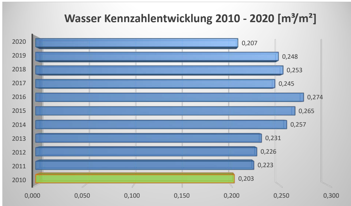
Abb. 7: Entwicklung der Wasserkennzahlen 2010 - 2020
