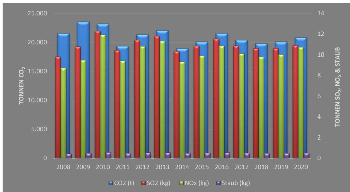
Abb. 27: Entwicklung der Emissionen von 2008 - 2020
