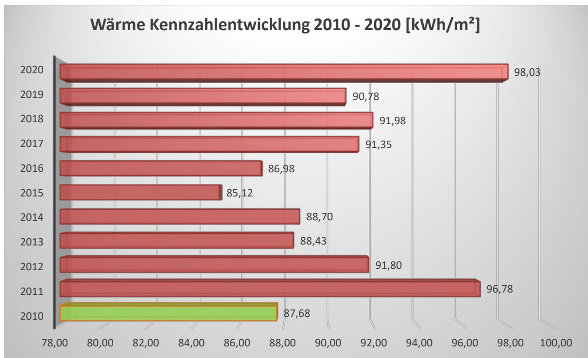
Abb. 5: Entwicklung der Wärme Kennzahlen 2010 – 2020 witterungsbereinigt
