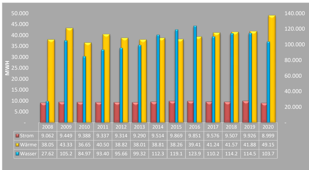
Abb. 8: Entwicklung des Medienverbrauchs städtischer Liegenschaften 2010-2020
