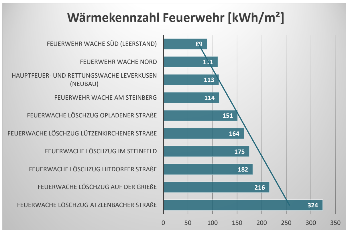
Abb. 17: Wärmekennzahl Feuerwehr 2020
