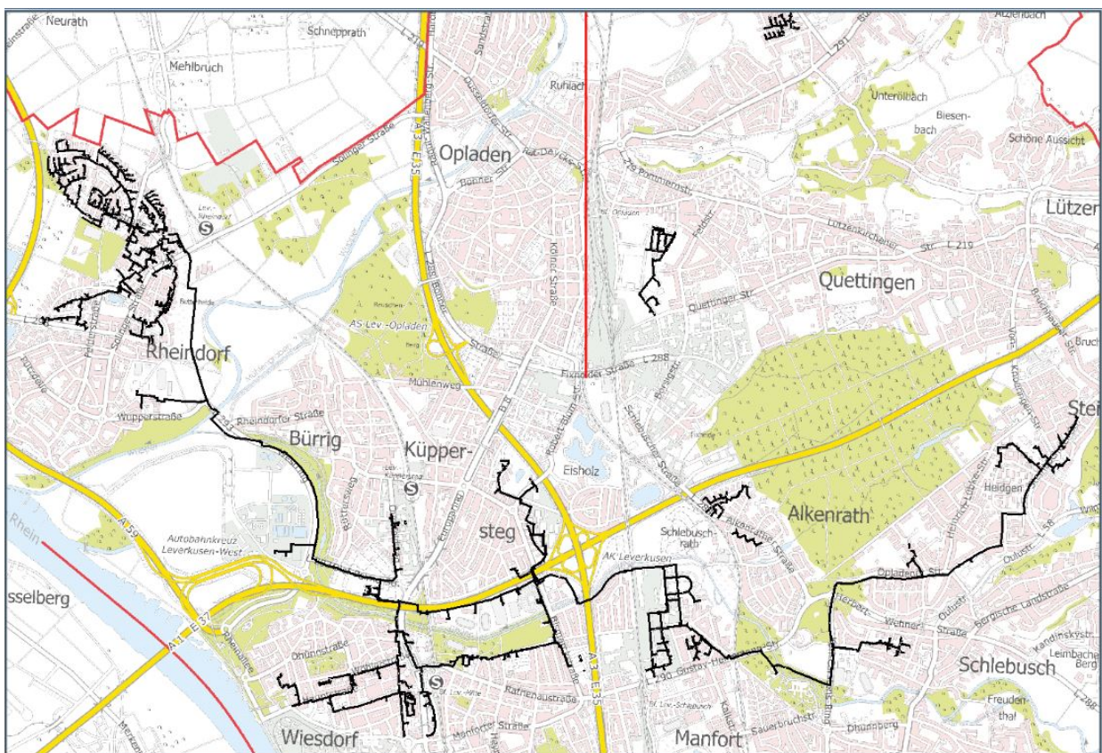
Abb. 32 Übersichtsplan Fernwärmenetze Stadtgebiet Leverkusen
