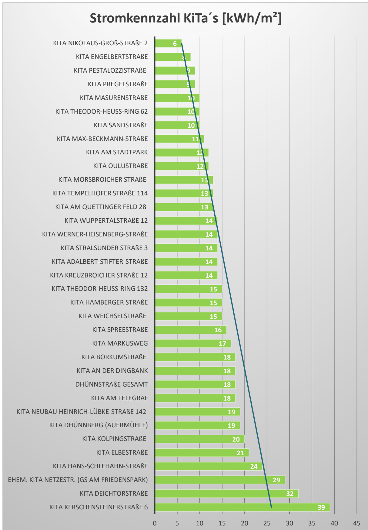
Abb. 14: Stromkennzahlen Kindertagesstätten 2020
