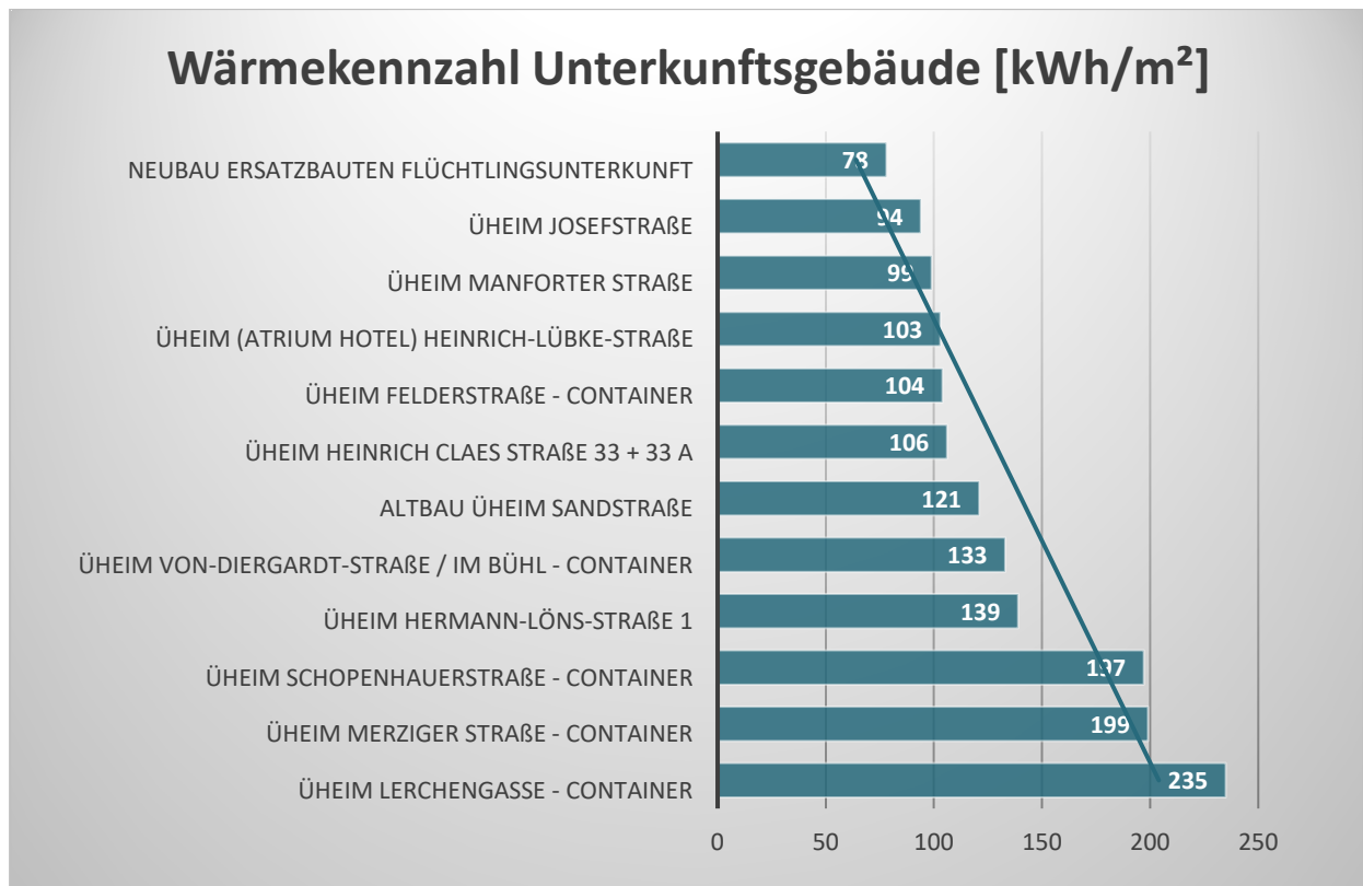
Abb. 21: Wärmekennzahl Unterkünfte 2020
