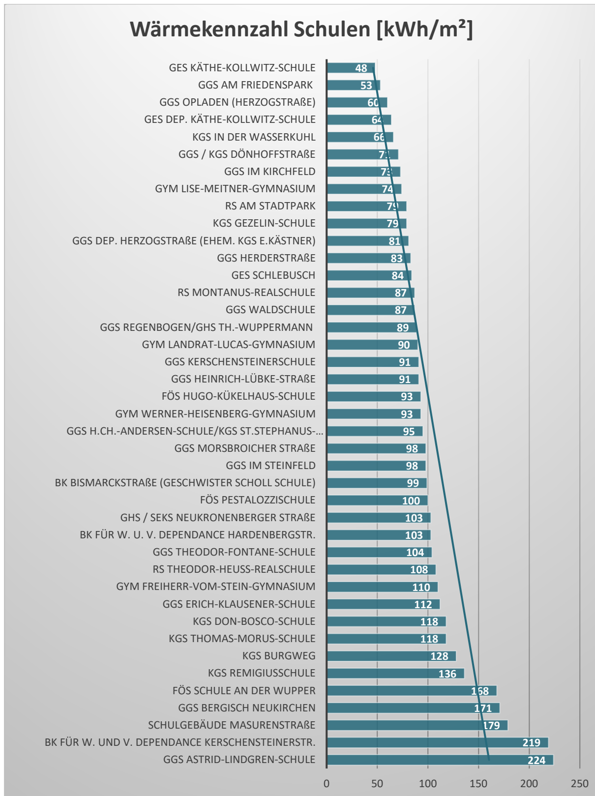
Abb. 11: Wärmekennzahl Schulen 2020
