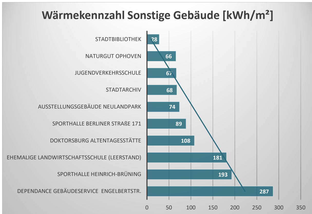
Abb. 24: Wärmekennzahl Sonstige Gebäude 2020
