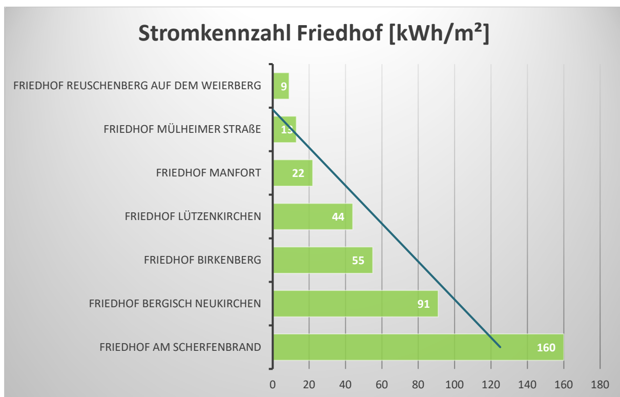
Abb. 23: Stromkennzahl Friedhöfe 2020
