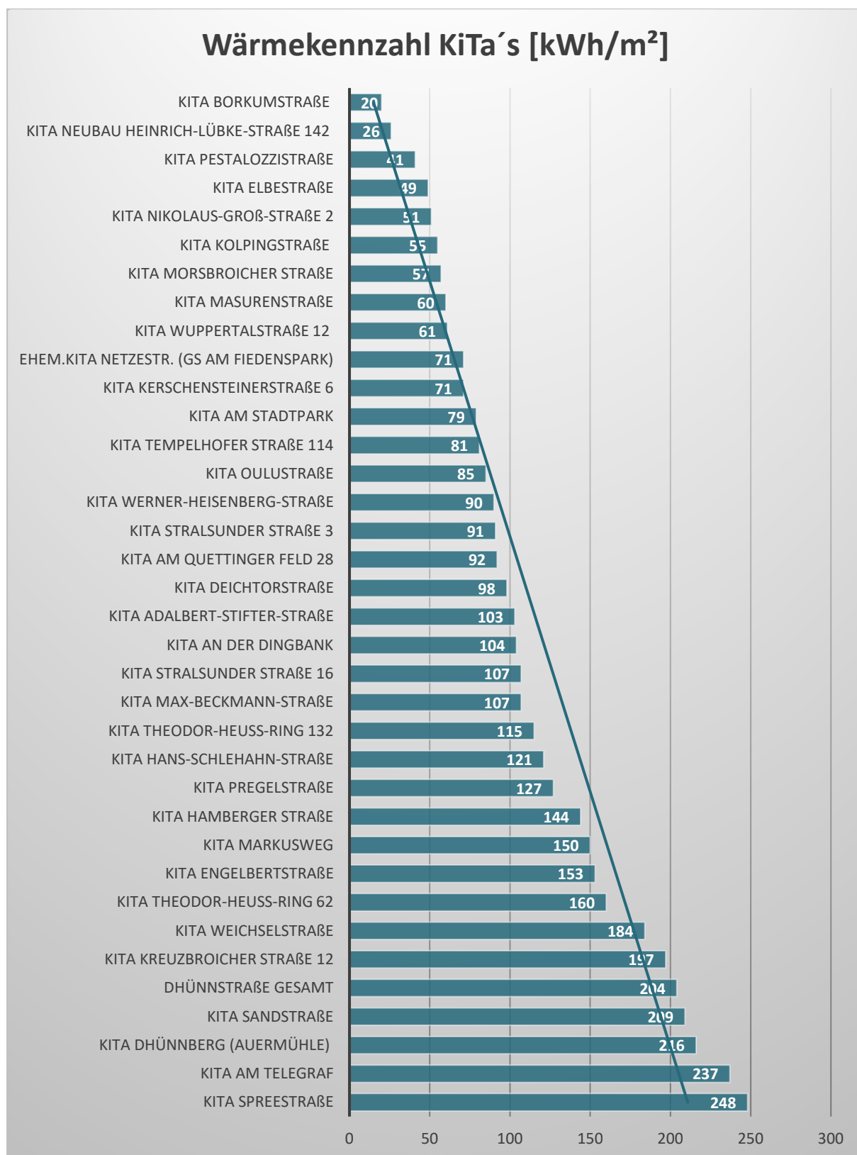
Abb. 13: Wärmekennzahl Kindertagesstätten 2020
