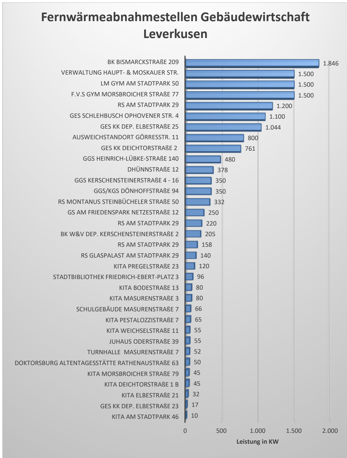
Abb. 33: Übersicht Fernwärmeabnahmestellen mit Leistungsangaben der GWL in 2020
