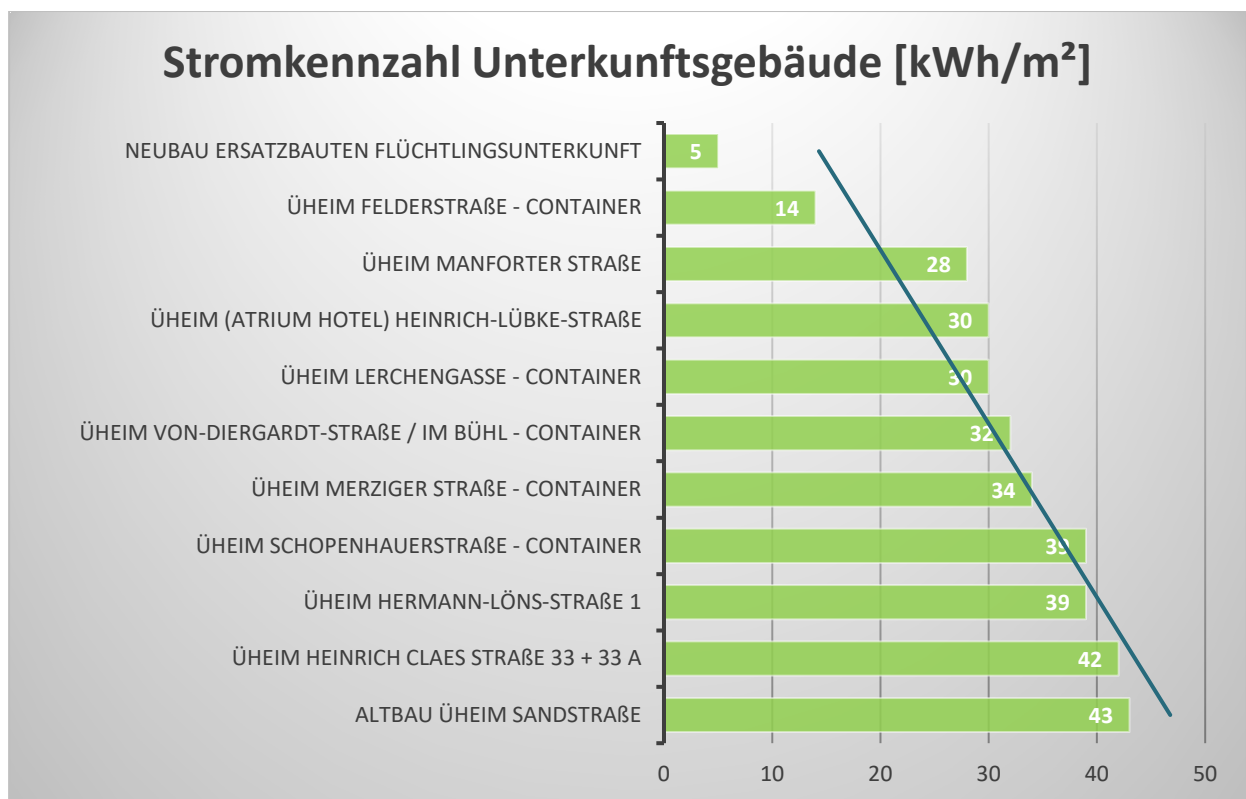
Abb. 21: Stromkennzahl Unterkünfte 2020
