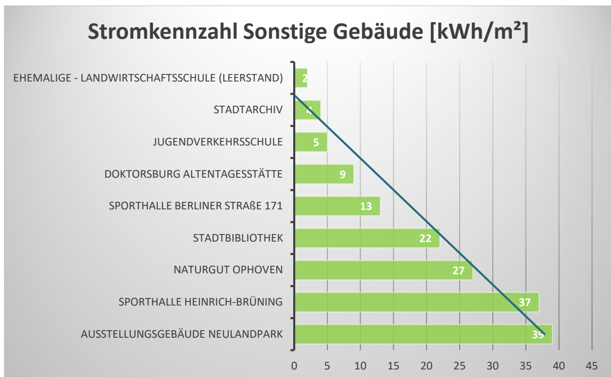
Abb. 25: Stromkennzahl Sonstige Gebäude 2020
