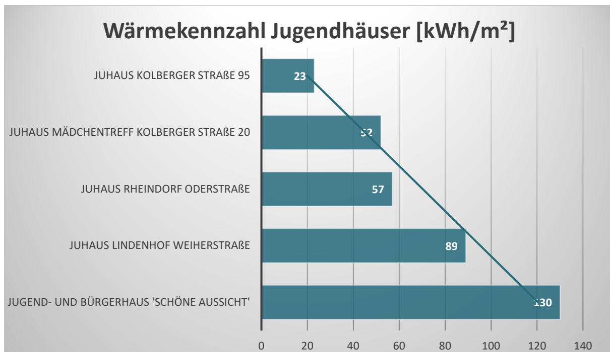
Abb. 19: Wärmekennzahl Jugendhäuser 2020
