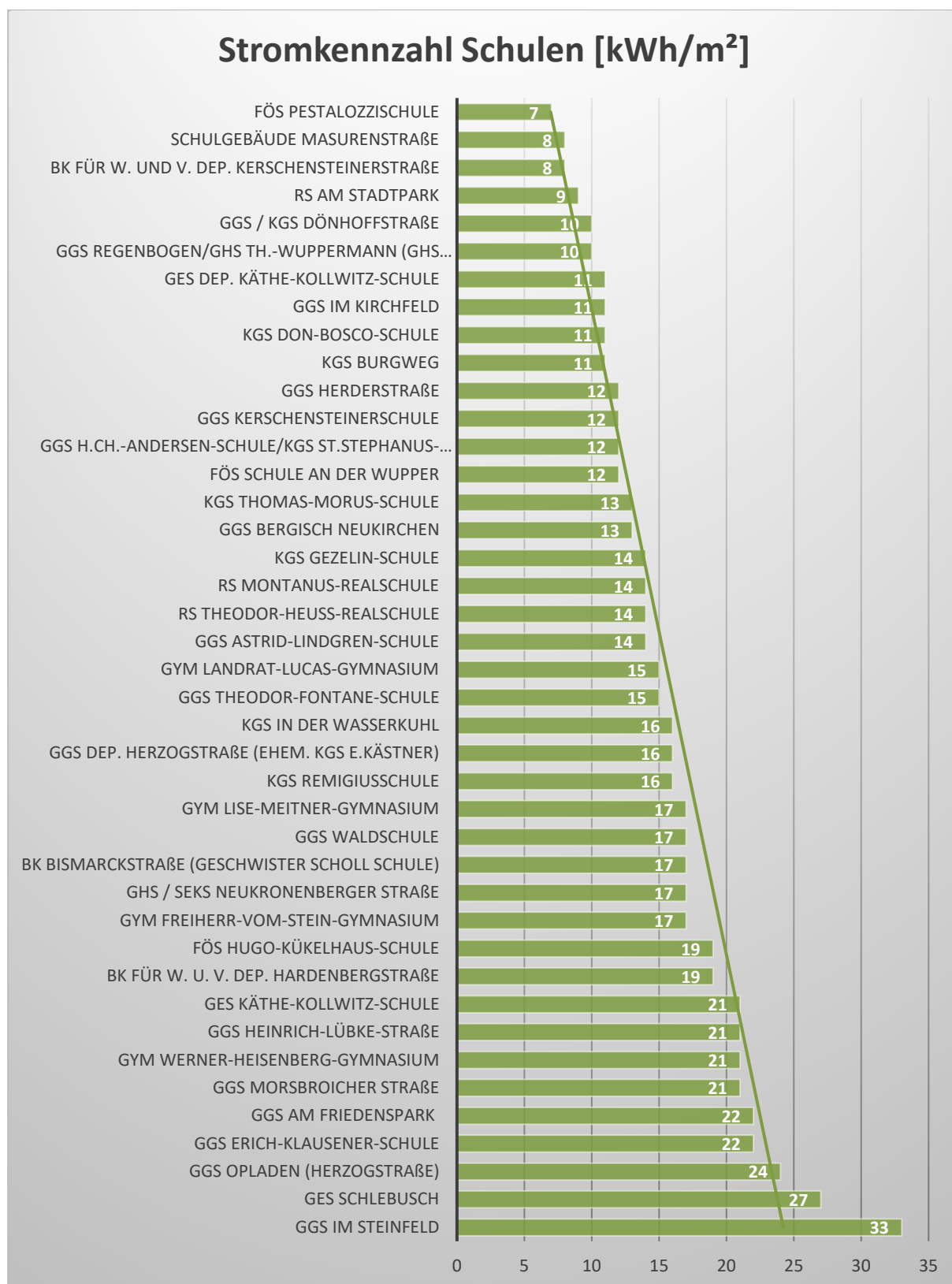
Abb. 12: Stromkennzahlen Schulen 2020
