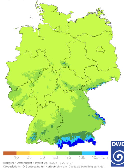
mittlere Bodenfeuchte unter Gras bei sandigem Lehm Aug. – Sep. 2021
