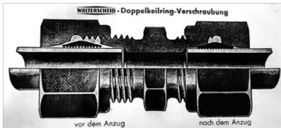
Doppelkeilring
