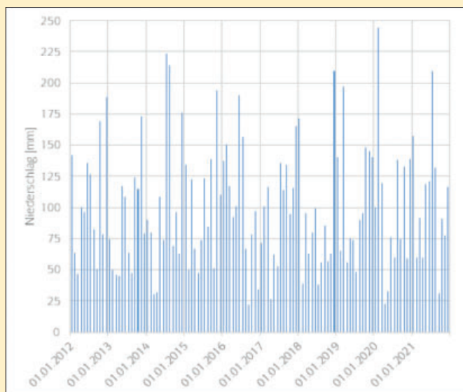
Grafik 1: Niederschlag im Wüstebach-Tal gemessen mit sechs Lysimetern: 1. Monatsmittelwert von 2012-2021. (Quelle: Forschungszentrum Jülich)
