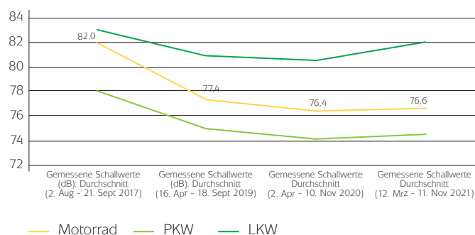
Grafik 37: Die durchschnittlichen Schallwerte an der L15 in der Nähe des barrierefreien Naturerkundungspfades „Der Wilde Weg“ haben sich nach Errichtung des Lärmschutzdisplays im April 2019 in den Motorradsaisons der Jahre 2019–2021 bei Motorrädern um 4,6 bis 5,6 Dezibel gegenüber Messungen ohne Display (2017) reduziert. 6 Dezibel entsprechen etwa einer Halbierung des Schalldrucks.
