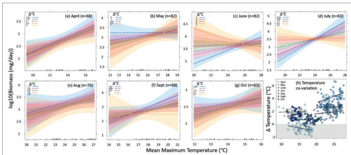
Abbildung 1: Deutschlandweites Insektenmonitoring mit Malaise-Fallen: Der Effekt von Temperatur auf die Biomasse fliegender Insekten in den Monaten April bis Oktober. Die Biomasse nimmt im Allgemeinen linear mit der Temperatur zu. Dieser Effekt kippt jedoch in den heißen Monaten Juni und Juli ins Negative, wenn lokale Temperaturen das langfristige Mittel übersteigen. Quelle: Welti et al. 2021
