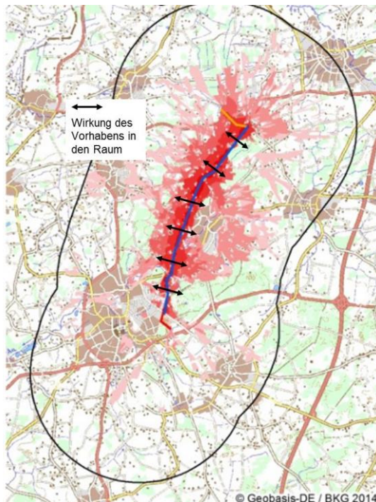
Abb. 10: Digitale Sichtbarkeitsanalyse zur Planfeststellung – Sichtbelastung durch geplante Freileitung
