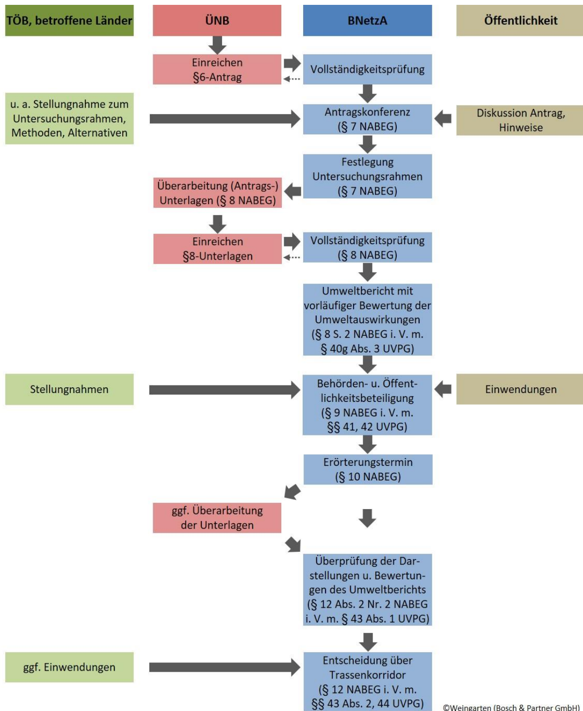
Abb. 7: Ablauf und Akteure der BFP
