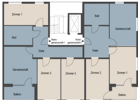
Grundriss 2./3. OG: je zwei Wohngemeinschaften mit je zwei bzw. drei Zimmern
