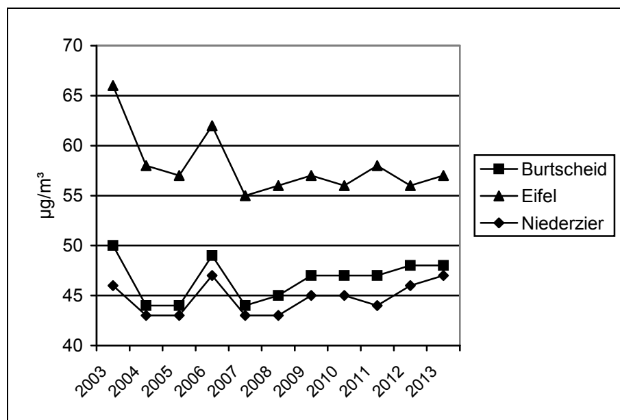
Abbildung 50: Ozon in der Außenluft in µg/m 3 , Jahresmittelwerte, Messstationen: Niederzier, Eifel (Simmerath) und Aachen-Burtscheid, 2003 - 2013
