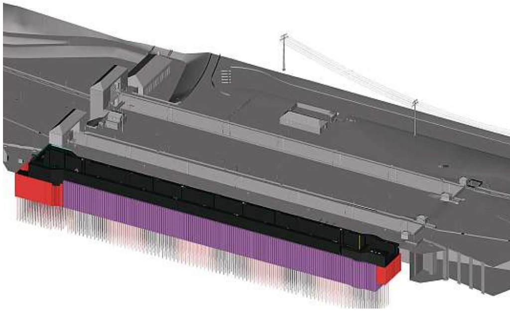
Bestandsmodell der Schleuse Wedtlenstedt ergänzt um die Planung der neuen Schleusenkammer und die Baugrubenumschließung.
