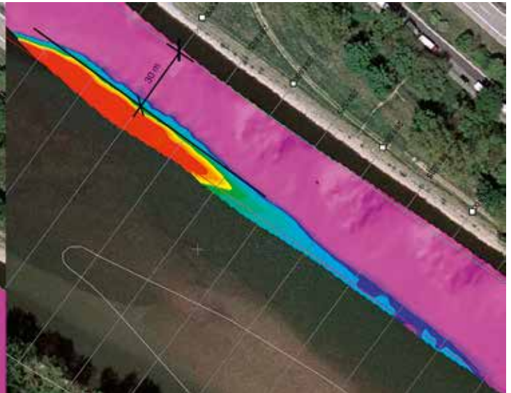
Peilung nach der Baggerung, Fahrinnenbreite 30 m
