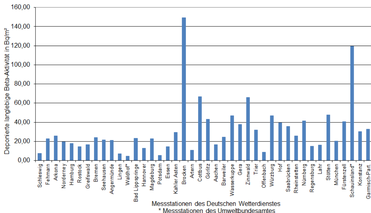
Abbildung B II 2.1-11 Dem Erdboden durch Niederschläge im Jahr 2016 zugeführte langlebige Gesamt- \beta -Aktivität – stationspezifische Jahressummen (Deposition of additional long-lived total \beta -activity due to precipitation - station specific annual total values in the year 2016)
