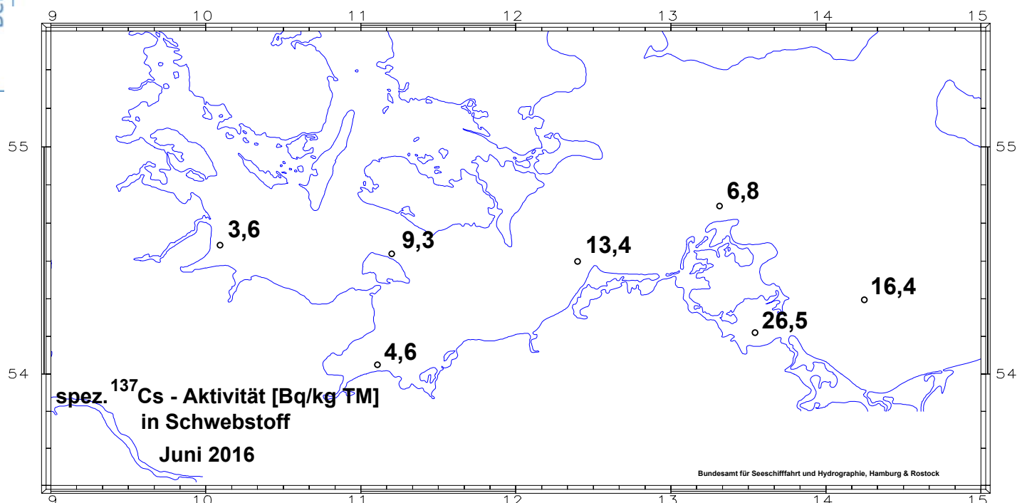
Abbildung B II 2.2-5 Spezifische Cs-137-Aktivität (Bq/kg TM) in Schwebstoff der westlichen Ostsee im Juni 2016
