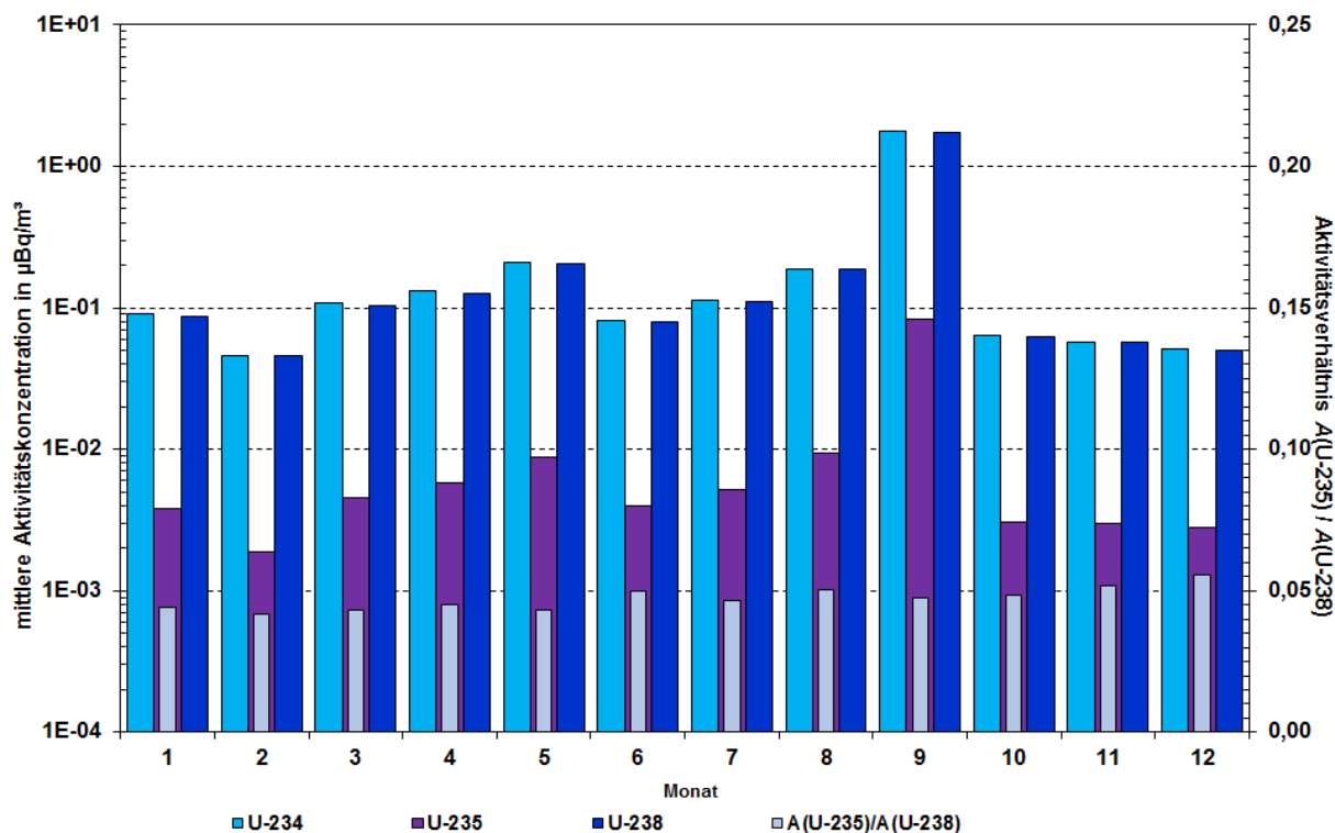
Abbildung B II 2.1-9 Aktivitätskonzentrationen und -verhältnisse der Uranisotope in der bodennahen Luft im Jahr 2016 am Probenentnahmeort Braunschweig (Activity concentrations and activity ratios of Uranium isotopes in ground-level air at the sampling site Braunschweig in 2016)
