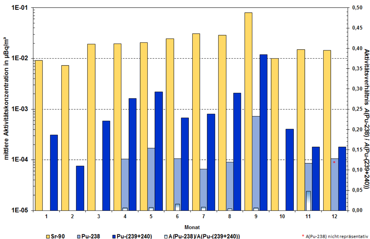
Abbildung B II 2.1-8 Aktivitätskonzentrationen der Plutoniumisotope und Sr-90 in der bodennahen Luft im Jahr 2016 am Probenentnahmeort Braunschweig (Activity concentrations Plutonium and Sr-90 in ground-level air at the sampling site Braunschweig in 2016)
