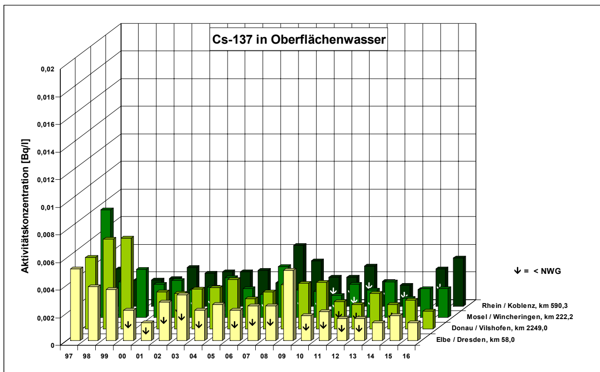
Abbildung B II 2.3-4 Aktivitätskonzentrationen (Bq/l) von Cs-137 in Oberflächenwasser ausgewählter Binnengewässer (Jahresmittelwerte) ( Cs-137 activity concentrations (Bq/l) in surface water from selected inland waters - annual mean values )
