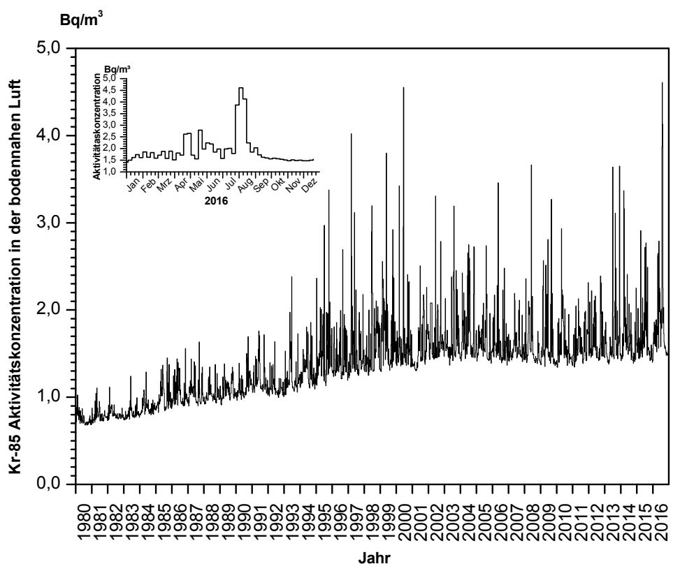
Abbildung B II 2.1-2 Kr-85-Aktivitätskonzentration in der bodennahen Luft am Probenentnahmeort Schauinsland (Kr-85-activity concentration in air close to ground level at the sampling location Freiburg/Schauinsland)
