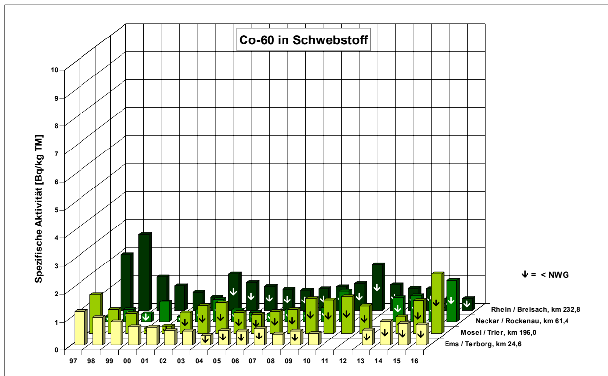
Abbildung B II 2.3-5 Spezifische Aktivitäten (Bq/kg TM) von Co-60 in Schwebstoffproben ausgewählter Binnengewässer (Jahresmittelwerte)
