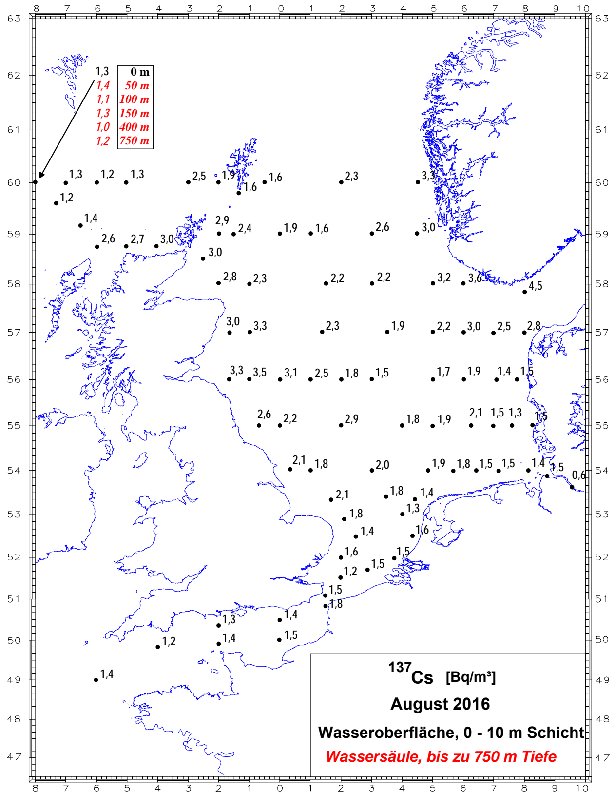
Abbildung B II 2.2-1 Die Verteilung der Aktivitätskonzentration von Cs-137 (Bq/m³) im Wasser der Nordsee im August 2016 (Distribution of the activity concentration of Cs-137 (Bq/m³) in seawater of the North Sea in August 2016)
