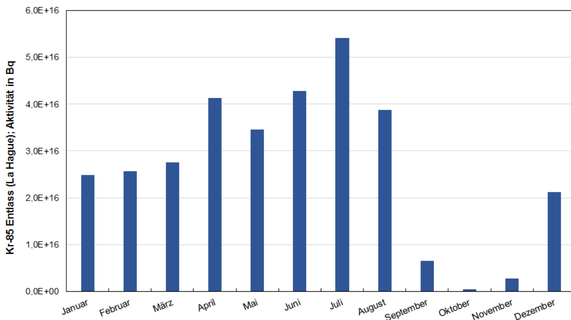
Abbildung B II 2.1-3 Monatlicher Kr-85-Entlass der Wiederaufbereitungsanlage La Hague für das Jahr 2016 ( Monthly emission of Kr-85 from La Hague reprocessing plant in 2016 )
