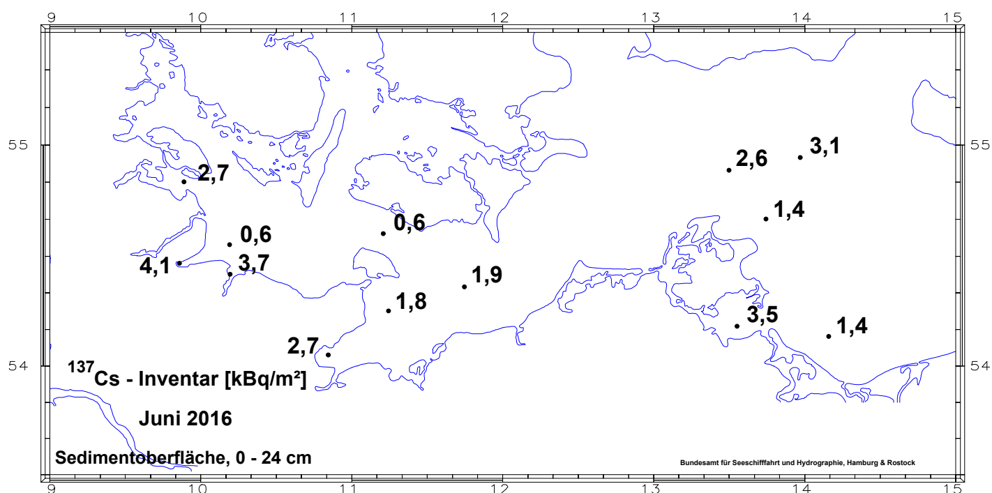
Abbildung B II 2.2-6 Cs-137 Inventar (kBq/m 2 ) in Sedimentkernen der westlichen Ostsee im Juni 2016. Das Inventar wird bis 24 cm Sedimenttiefe erfasst.
