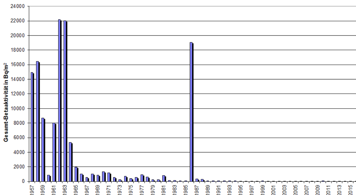
Abbildung B II 2.1-10 Dem Erdboden durch Niederschläge zugeführte langlebige Gesamt- \beta -Aktivität - Jahresmittelwerte der Jahressummen an den DWD-Messstationen von 1957 bis 2016 (Deposition of additional long-lived total \beta -activity due to precipitation - Annual mean value for the total annual levels determined at the DWD measuring stations, 1957 - 2016)
