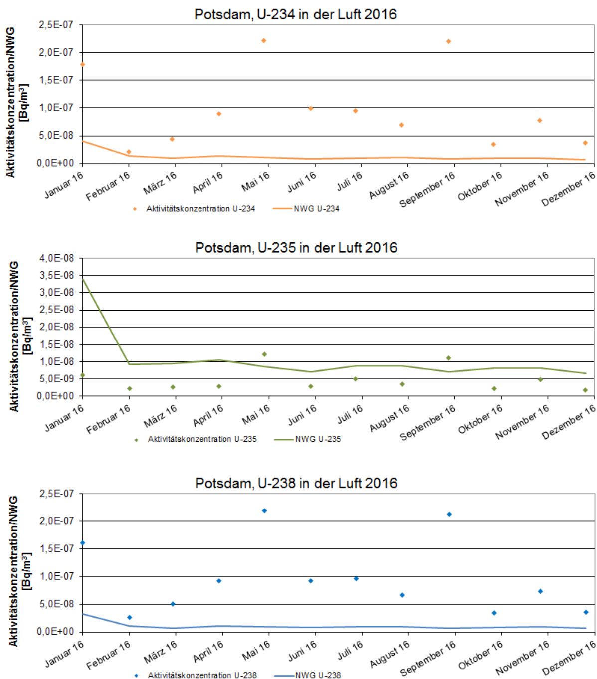
Abbildung B II 2.1-7 Aktivitätskonzentrationen in der bodennahen Luft von Uranisotopen für das Jahr 2016 am Probenentnahmeort Potsdam (Activity concentrations and activity ratio of Uranium isotopes in ground-level air at the sampling site Potsdam in 2016)
