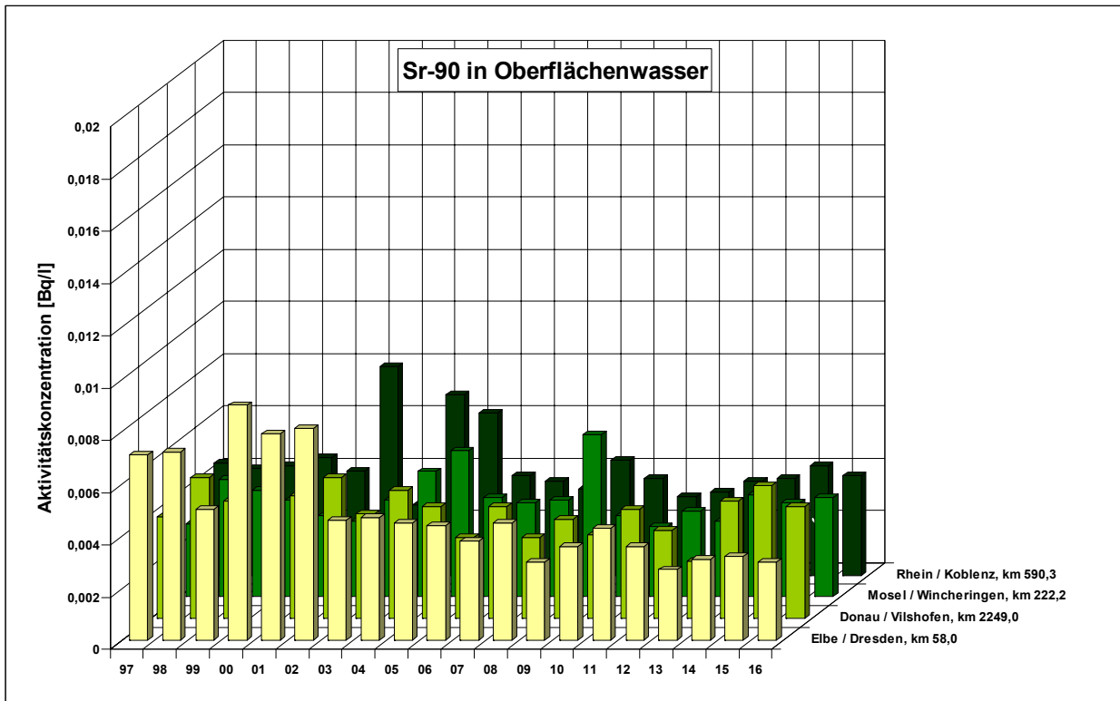
Abbildung B II 2.3-3 Aktivitätskonzentrationen (Bq/l) von Sr-90 in Oberflächenwasser ausgewählter Binnengewässer (Jahresmittelwerte) ( Sr-90 activity concentrations (Bq/l) in surface water from selected inland waters - annual mean values )
