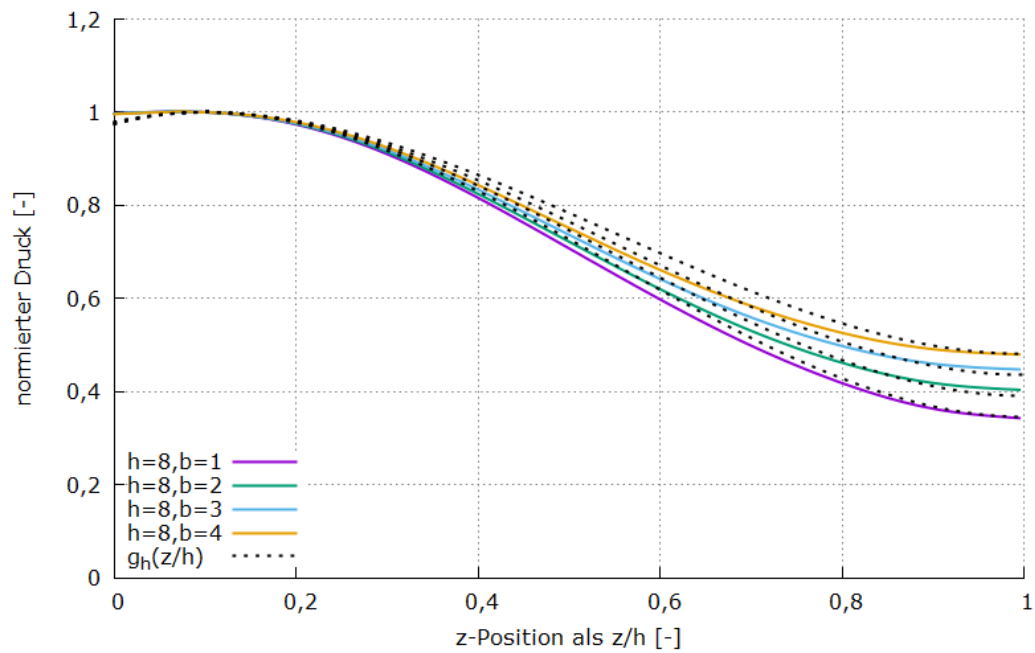
Abbildung 46: Höhenverlauf der Drucklast für h=8 m und Formfunktion g_h(z/h) für verschiedene Auskrabreiten.
