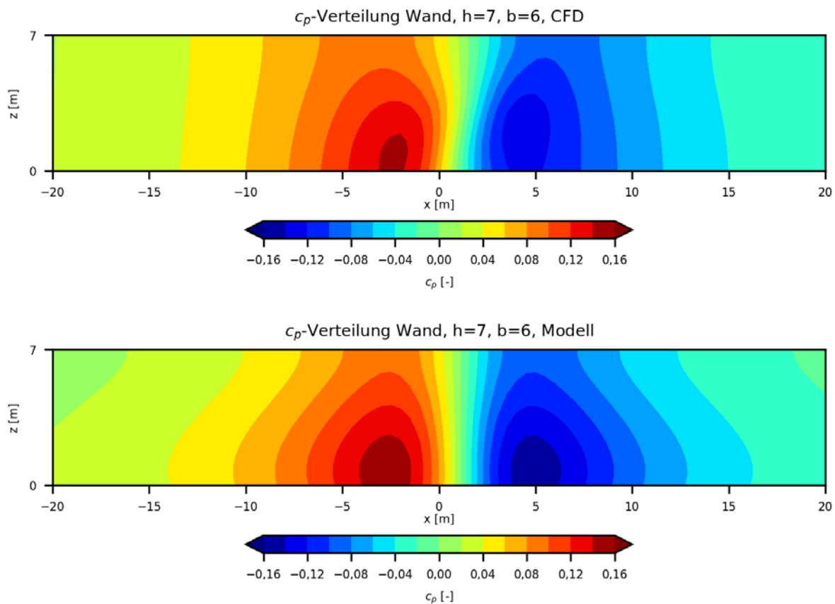
Abbildung 61: c_p -Verteilung auf der Wand aus der CFD-Simulation (oben) und dem analytischen Modell (unten)
