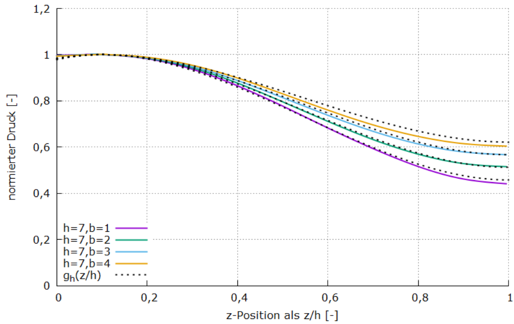
Abbildung 45: Höhenverlauf der Drucklast für h=7 m und Formfunktion g_h(z/h) für verschiedene Auskrabreiten.
