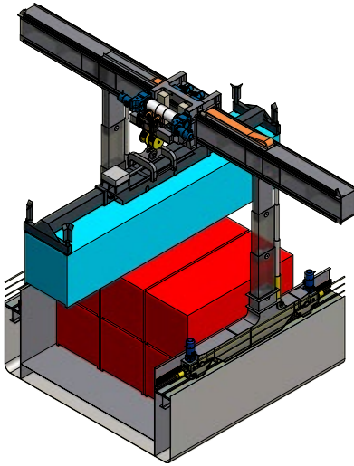
Abb. 6: Entwickelter verfahr- und teleskopierbarer Portalkran mit seitlich klappbaren Brückenträger, Winkelkatze und Containerspreader als Lastaufnahmemittel
