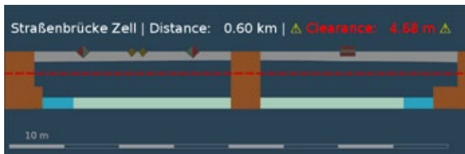
Abb. 14: Brücke mit temporärer Einschränkung der Durchfahrtshöhe
