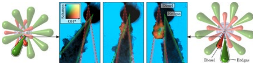
Abb. 3: Kreuzende Strahlen bei Zweinadel-Konzept (links) und tangentiale Ausbreitung bei Mehrnadel-Konzept (rechts); ausbleibende Pilotzündung bei zunehmender Kreuzung
