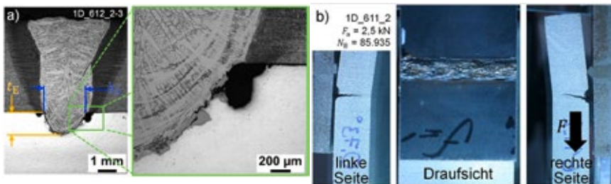
Abb. 7: Nahtquerschnitt der gependelt geschweißten Überlappnaht (VR 1D) mit Geometrieangaben (a) und Versagensverhalten im Schwingfestigkeitsversuch (b)
