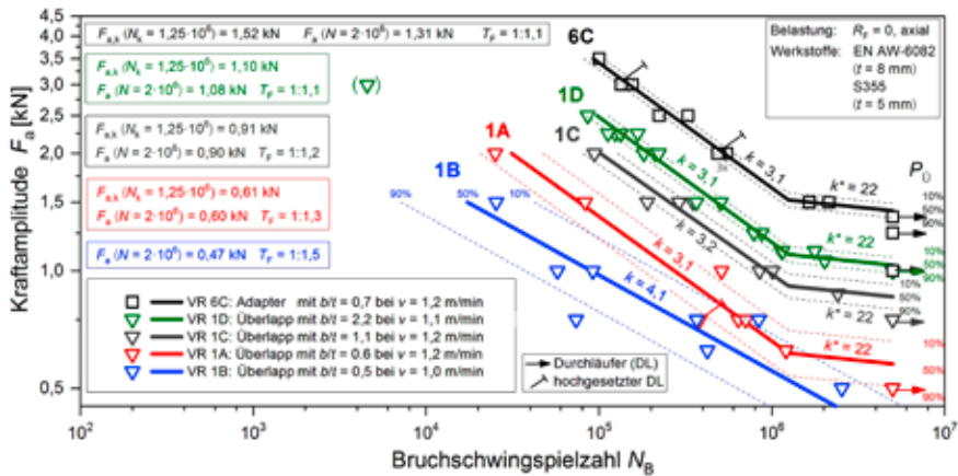
Abb. 8: Schwingfestigkeitsergebnisse für Überlappnähte und Adapter der Variante 1
