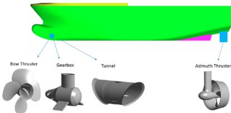
Abb. 6: Untersuchtes Offshore-Versorger-Schiff inklusive Querstrahler und Hauptantrieb.
