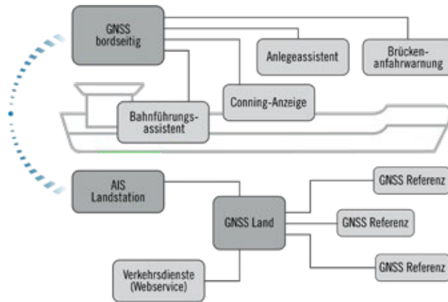
Abb. 1: LAESSI Systemaufbau
