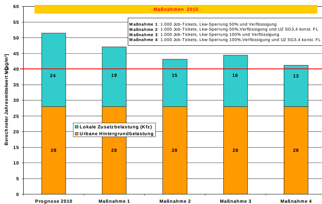
Abb. 6/1: Immissionsminderungspotenziale bezüglich \text{NO}_2 unterschiedlicher Maßnahmenpakete in Bonn (siehe LRP Bonn 2009, Seite 110)
