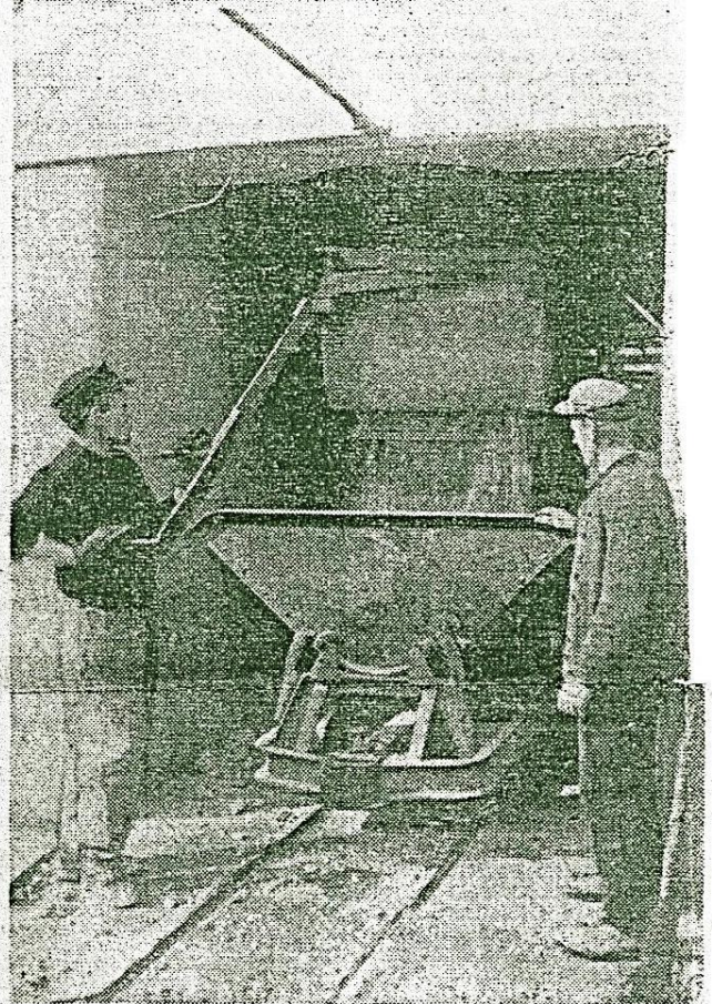
Die gebrannte Schamotte wird in die bereitstehenden Loren abgelassen
