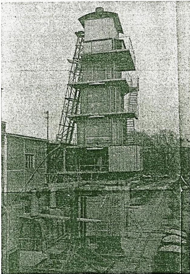
Der neue Schamotte-Ofen mit dem Gebäude des Gasgenerators
