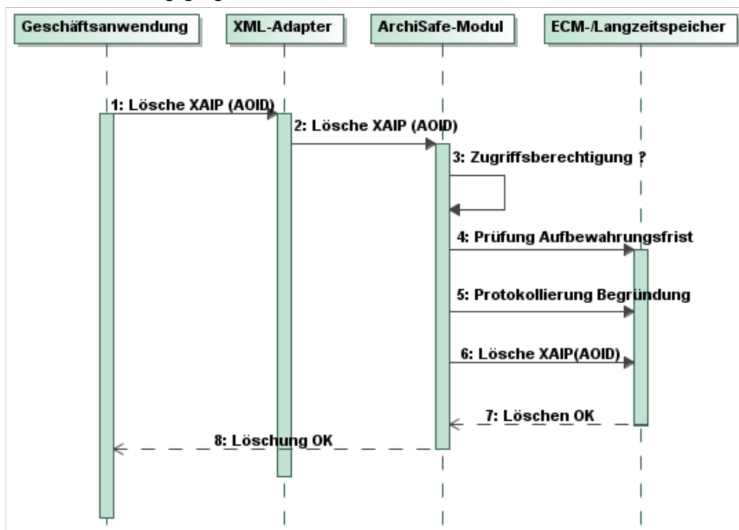
Abbildung 8: Schematischer Ablauf des Löschens von Archivdatenobjekten
