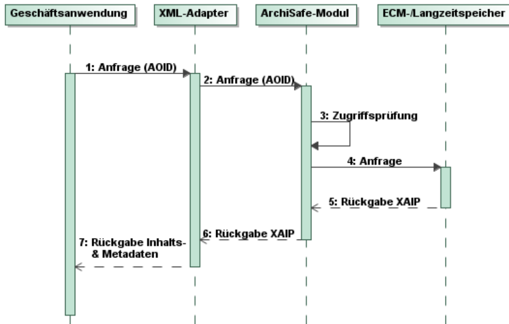
Abbildung 6: Abfrage archivierter Daten
