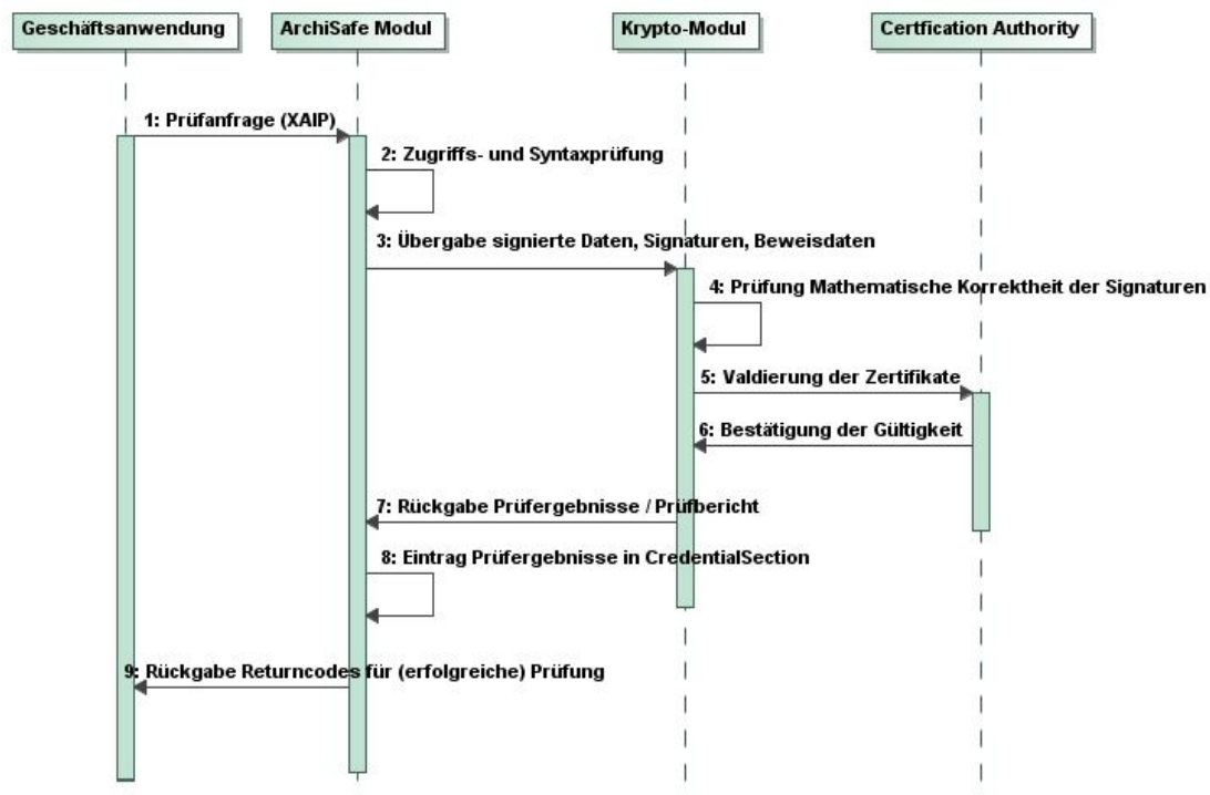
Abbildung 9: Prüfung von beweisrelevanten Daten (z.B. Signaturen) und Beweisdaten
