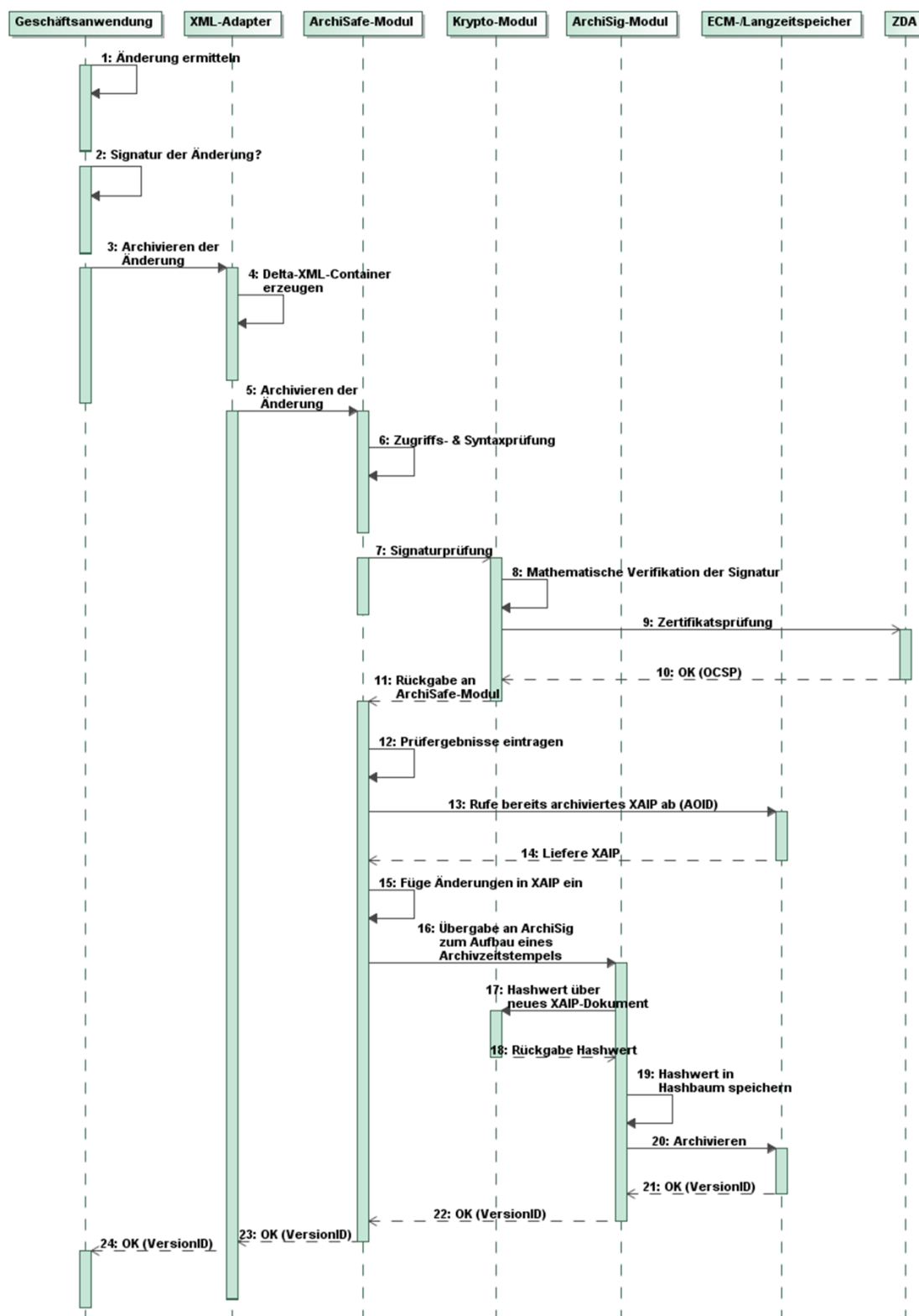
Abbildung 5: Ändern archivierter Daten
