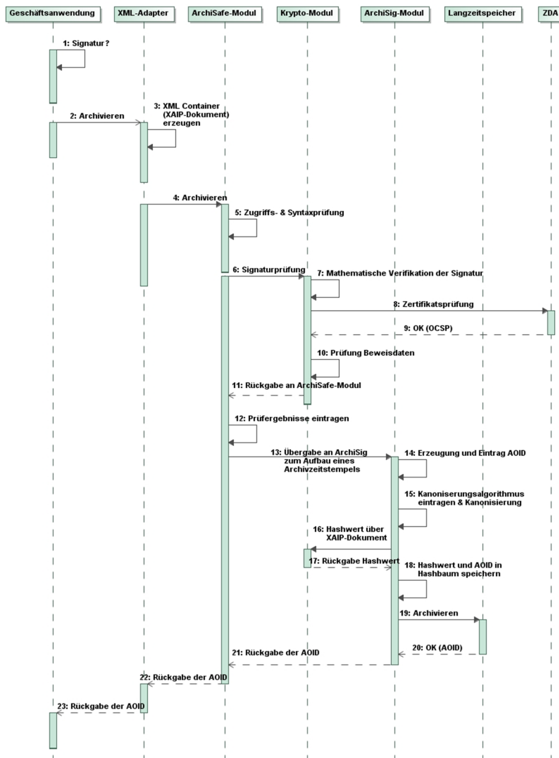
Abbildung 4: Schematischer Ablauf der Archivierung
