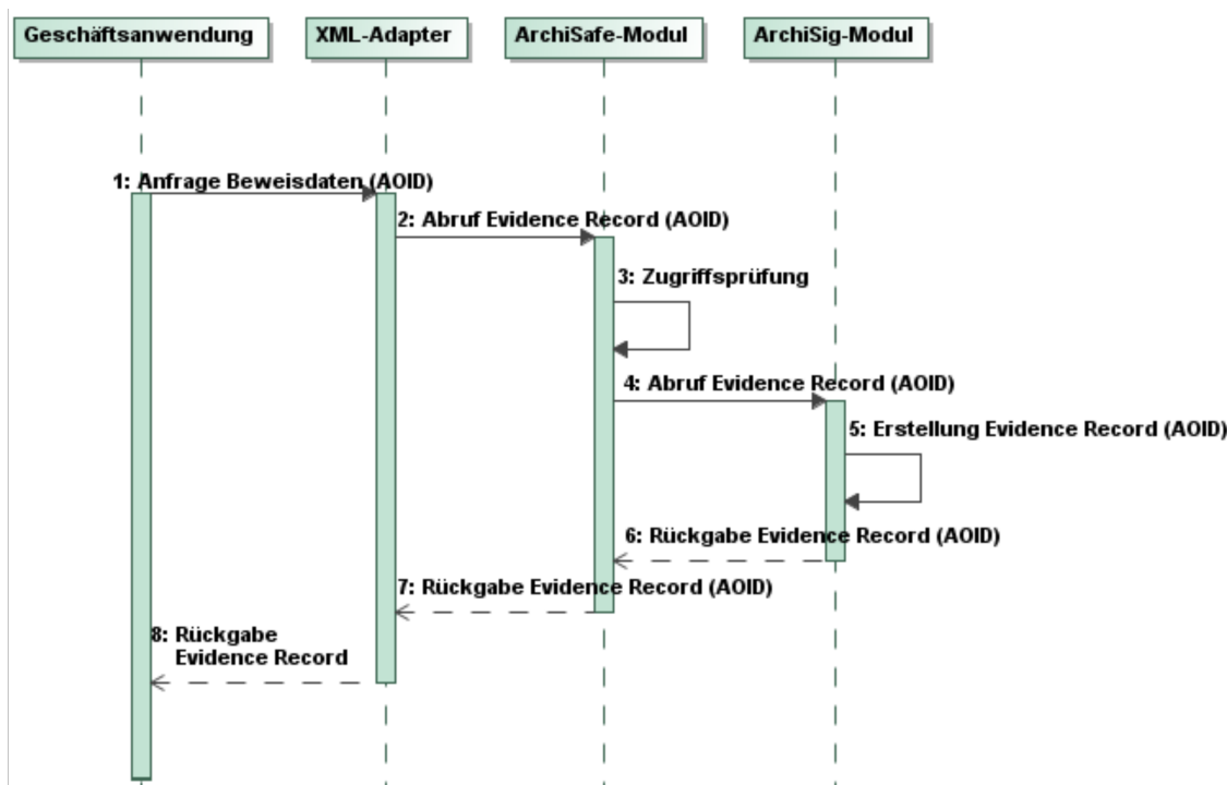
Abbildung 7: Schematischer Ablauf des Abrufs technischer Beweisdaten
