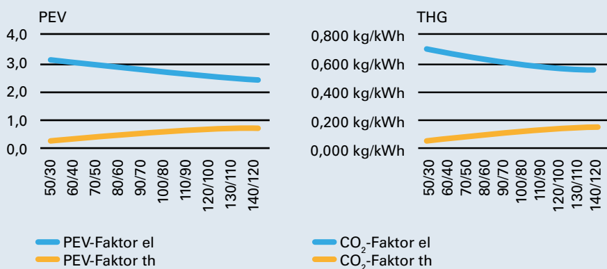
Abb. 9: Primärenergie und THG Faktoren, abhängig von der Temperatur des Wärmenetzes (Begleitforschung energetische Stadtanierung, Matthias Wangelin)
