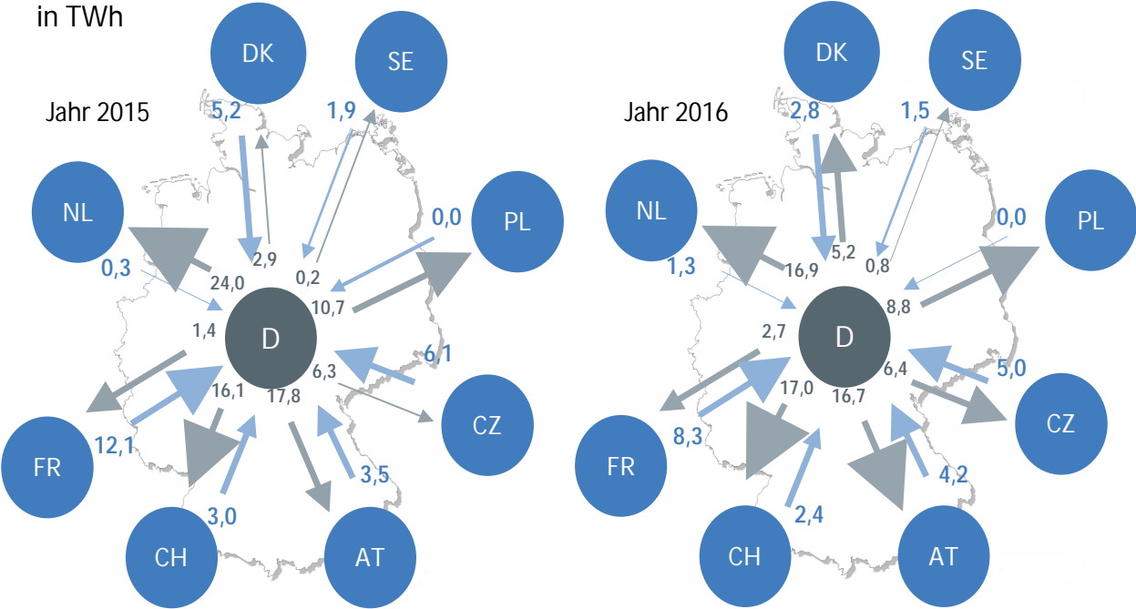
Abbildung 69: Physikalische Lastflüsse
