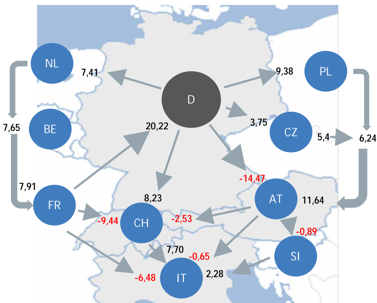
Abbildung 74: Ungeplante Flüsse 2015
