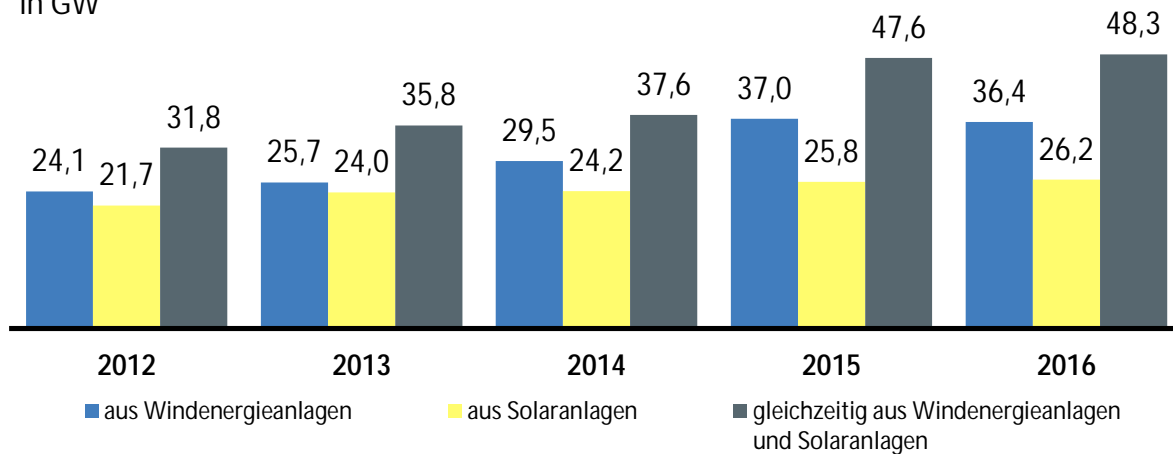
Abbildung 16: Maximale Einspeisung
