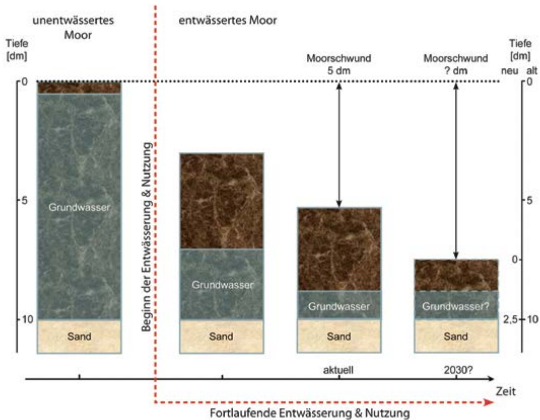
Schematische Darstellung der Bodenentwicklung eines flachgründigen Niedermoors bei fortlaufender Entwässerung und Moornutzung
