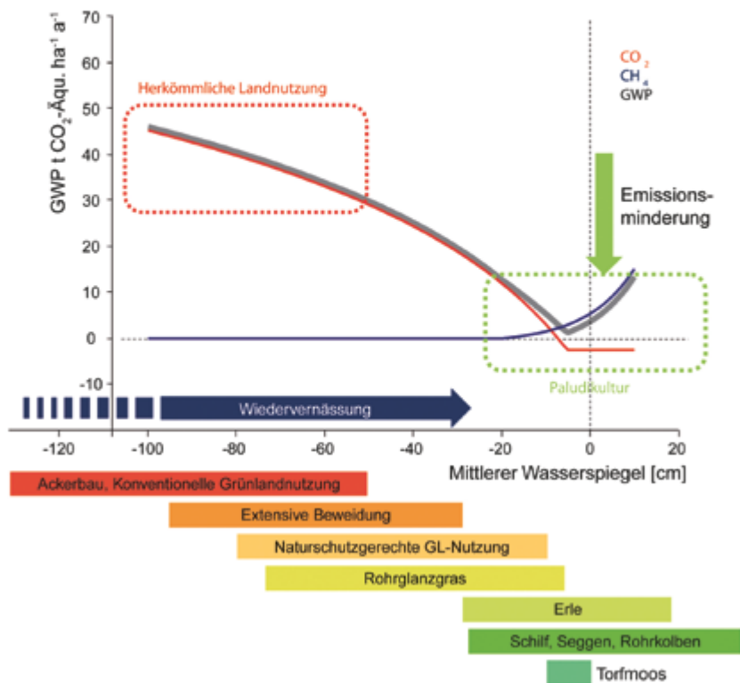
Schematische Darstellung von Treibhausgas-Emissionen (ohne N_2O ) und ausgewählten, landwirtschaftlichen Nutzungsmöglichkeiten auf Moorböden in Abhängigkeit vom mittleren Wasserstand. Eine Anhebung des Wasserstandes knapp unter Flur ermöglicht eine starke Reduktion von Treibhausgas-Emissionen, erfordert jedoch die Etablierung neuer landwirtschaftlicher Nutzpflanzen (Paludikulturen)
