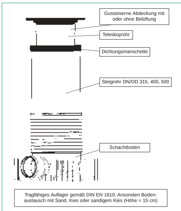
Bild 2: Inspektionsschacht / Bauteile
