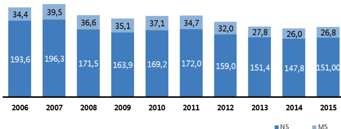
Abbildung 39: Anzahl der Versorgungsunterbrechungen in der NS und in der MS von 2006 bis 2015
