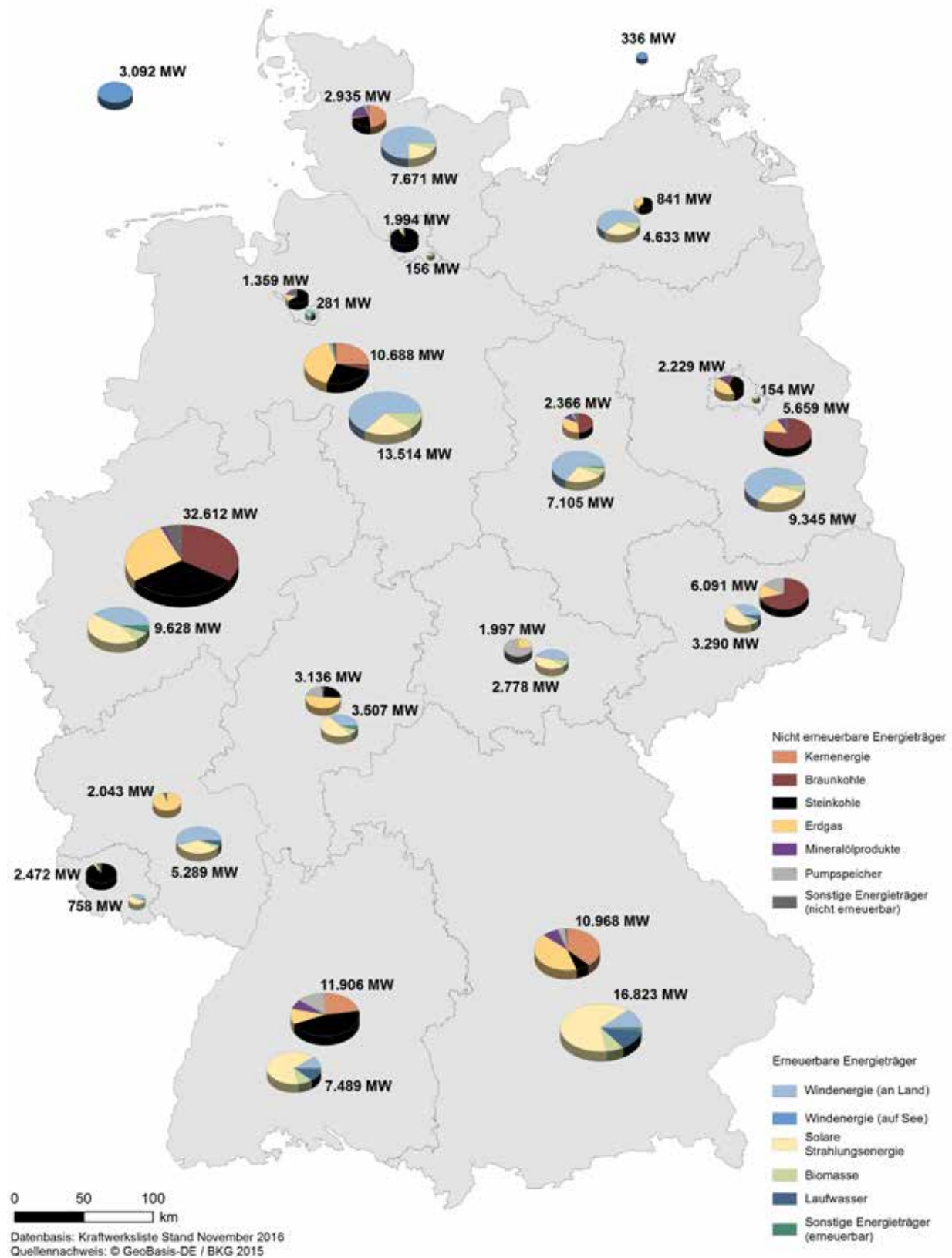
Abbildung 9: Erzeugungskapazitäten nach Energieträgern je Bundesland (Netto-Nennleistungen, Stand November 2016, EEG 31. Dezember 2015)
