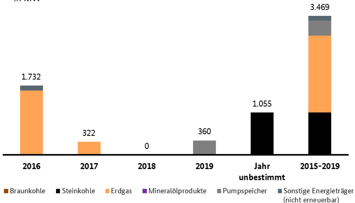
Abbildung 13: In Probetrieb oder in Bau befindliche Kraftwerke 2016 bis 2019 (Bundesweite Plandaten 2016 bis 2019 für Netto-Nennleistungen, Stand: November 2016)
