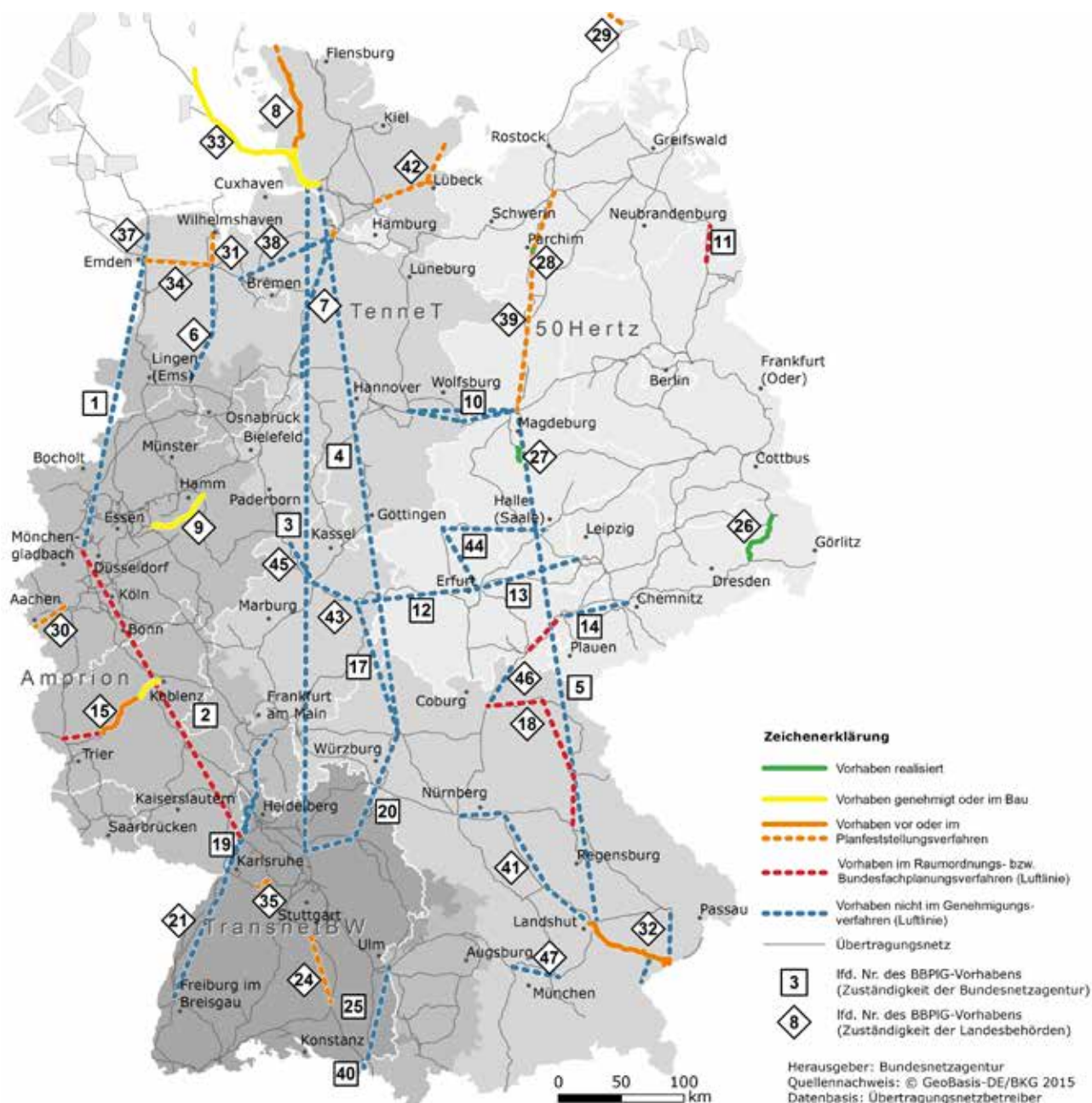
Abbildung 26: Stand der Ausbauvorhaben nach dem Bundesbedarfsplangesetz (BBPlG) zum dritten Quartal 2016
