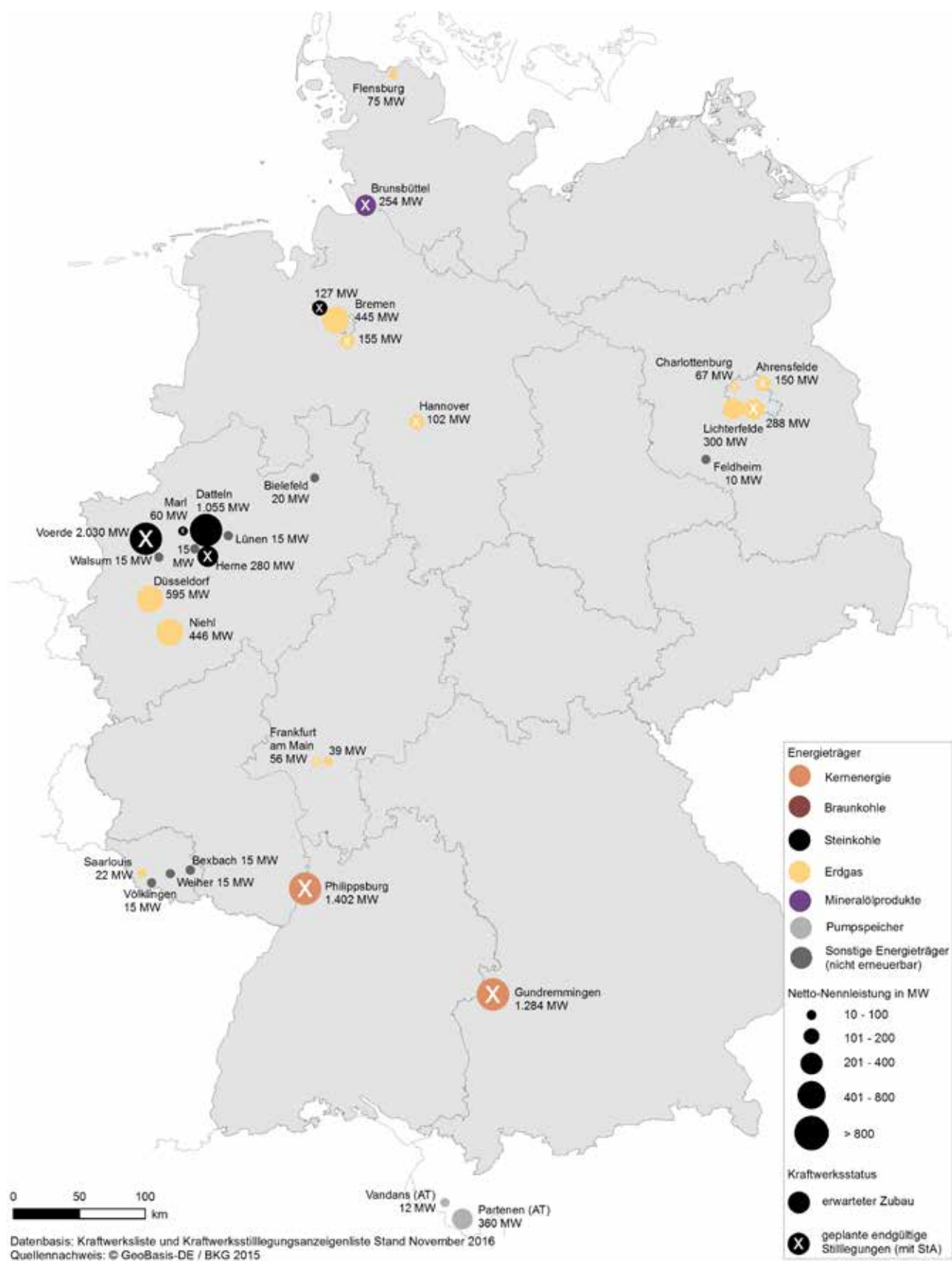
Abbildung 14: Standorte mit erwartetem Zu- und Rückbau von Kraftwerksblöcken (Stand November 2016)
