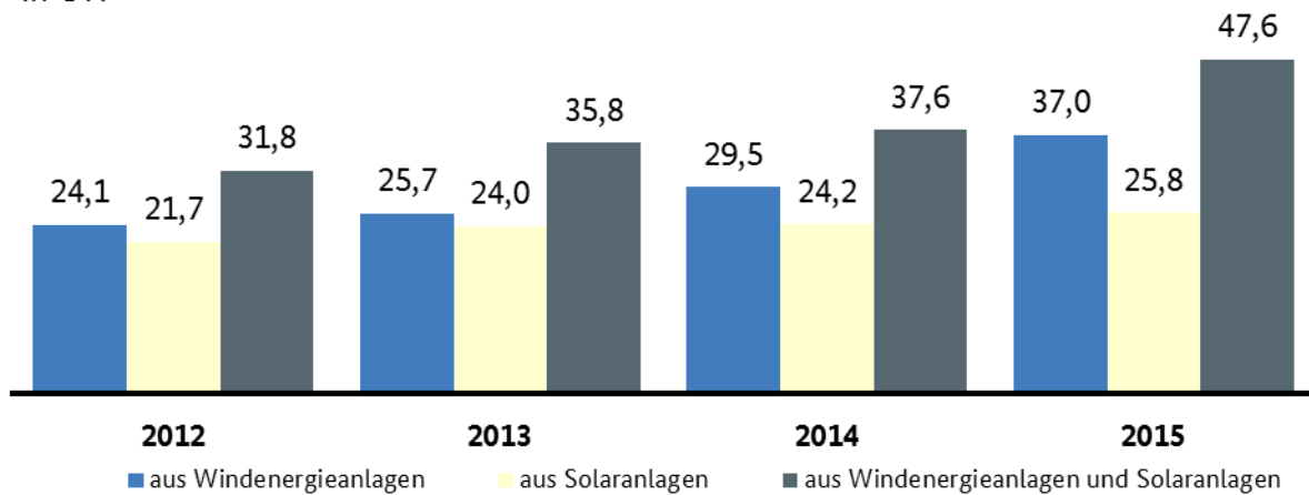
Abbildung 18: Maximale Einspeisung
