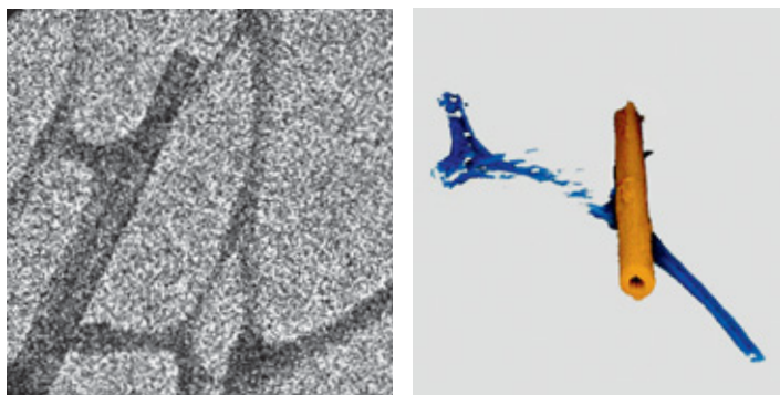
Auf Bildern wie dem linken basiert die tomografische 3-D-Rekonstruktion eines Nanoröhrchens (rechts, orange) auf einer Kohlenstoff-Trägerschicht (blau).
