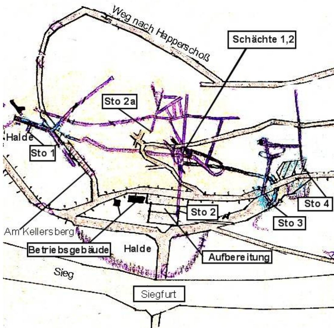
Bild 20: Abbauschwerpunkt der Grube Ziethen 1853 - 1878 (Sto = Stollen)
