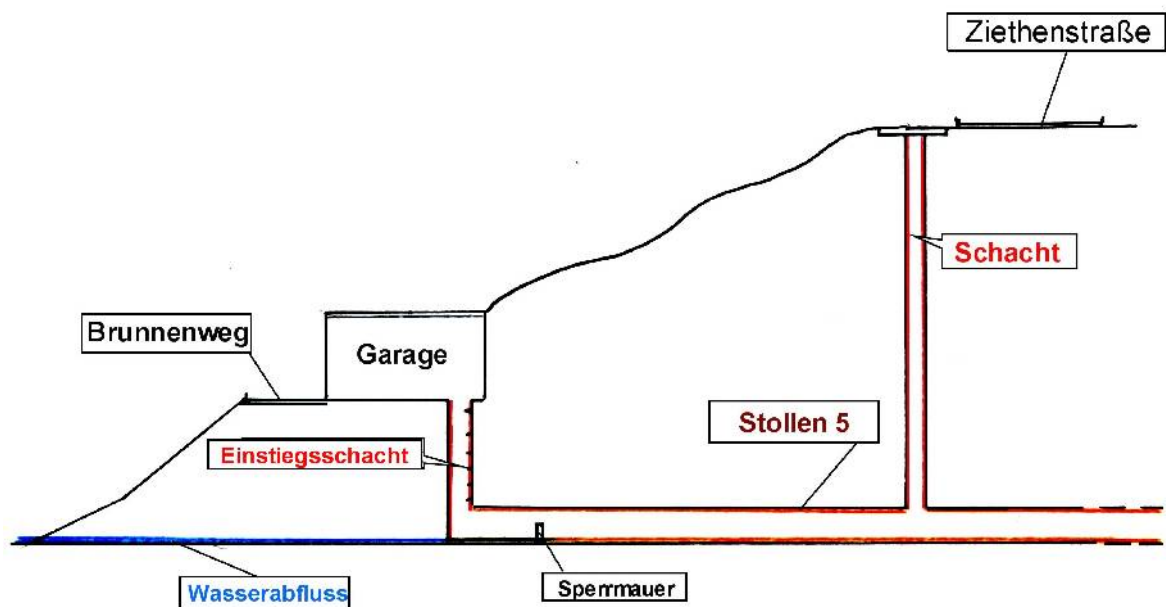
Bild 32: Stollen 5 (Weingartsgasser Stollen) oben: Stollenbereich; unten: Situationsskizze
