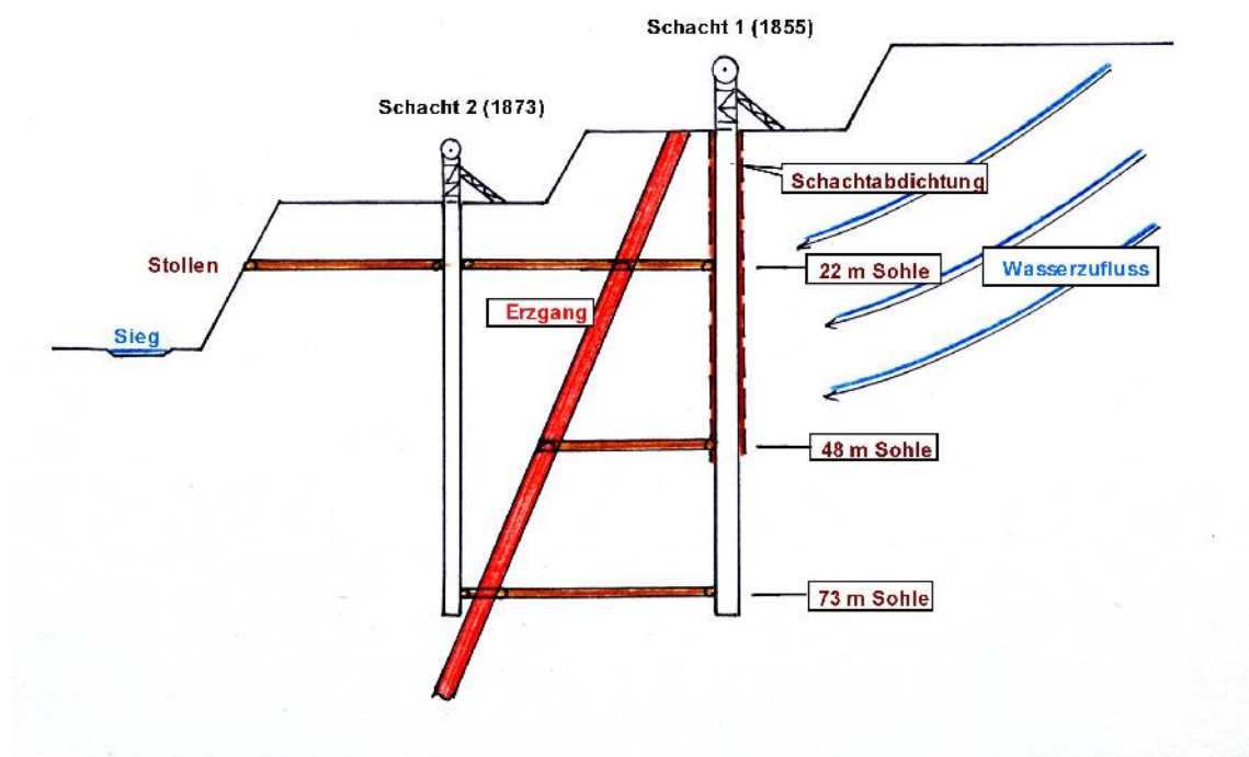
Bild 19: Grube Ziethen 1853 – 1878 (schematischer Querschnitt)
