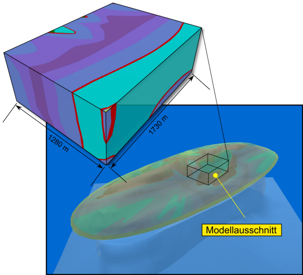
Abb. 5.6 Erstellung eines geeigneten Modellausschnitts für die thermische Simulation der Bohrlochlagerung (Experiment 2)
