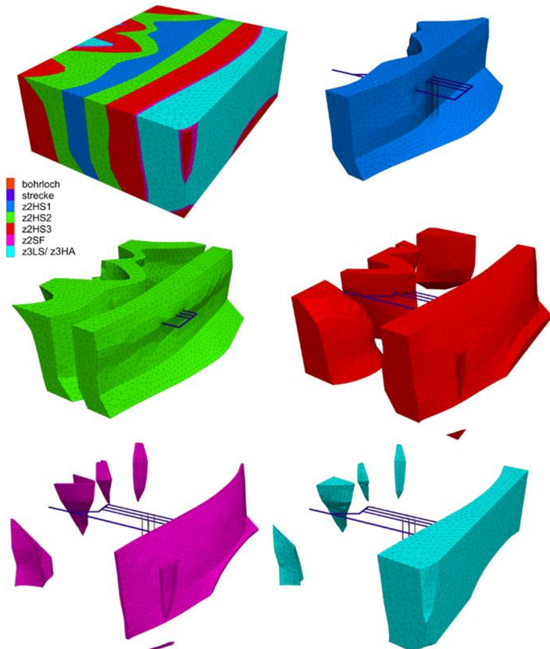
Abb. 5.13 Darstellung des vernetzen Modell in \text{FLAC}^{3\text{D}} mit Darstellung des Gesamtmodells und der einzelnen geologischen Einheiten
