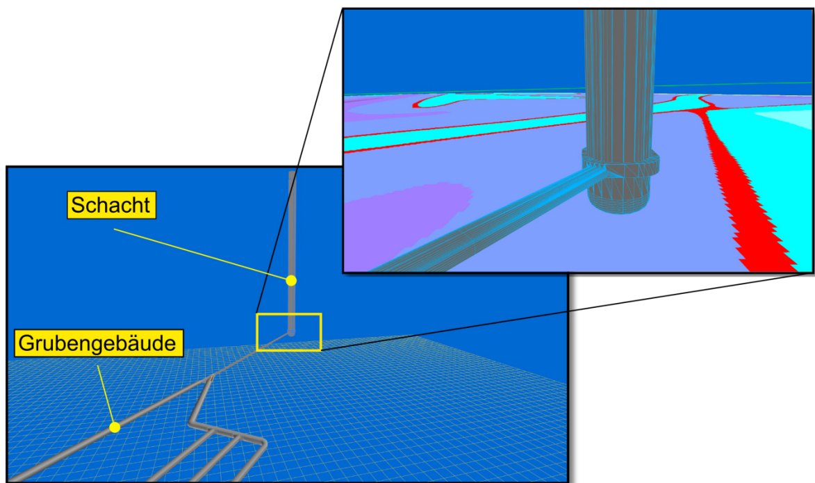
Abb. 4.9 Planung von Schächten mit den in VIRTUS implementierten Werkzeugen
