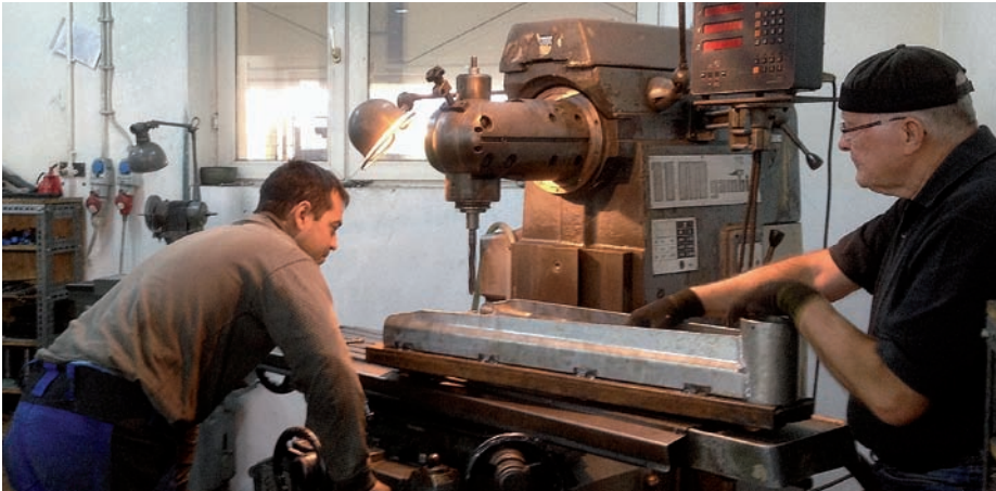
Rumänien: 'Hausdorf Step' will den Zukauf von Treppenbauteilen reduzieren. Gerd van Düllen fertigt Klemmschablone für die Herstellung von Stahlstufen.
