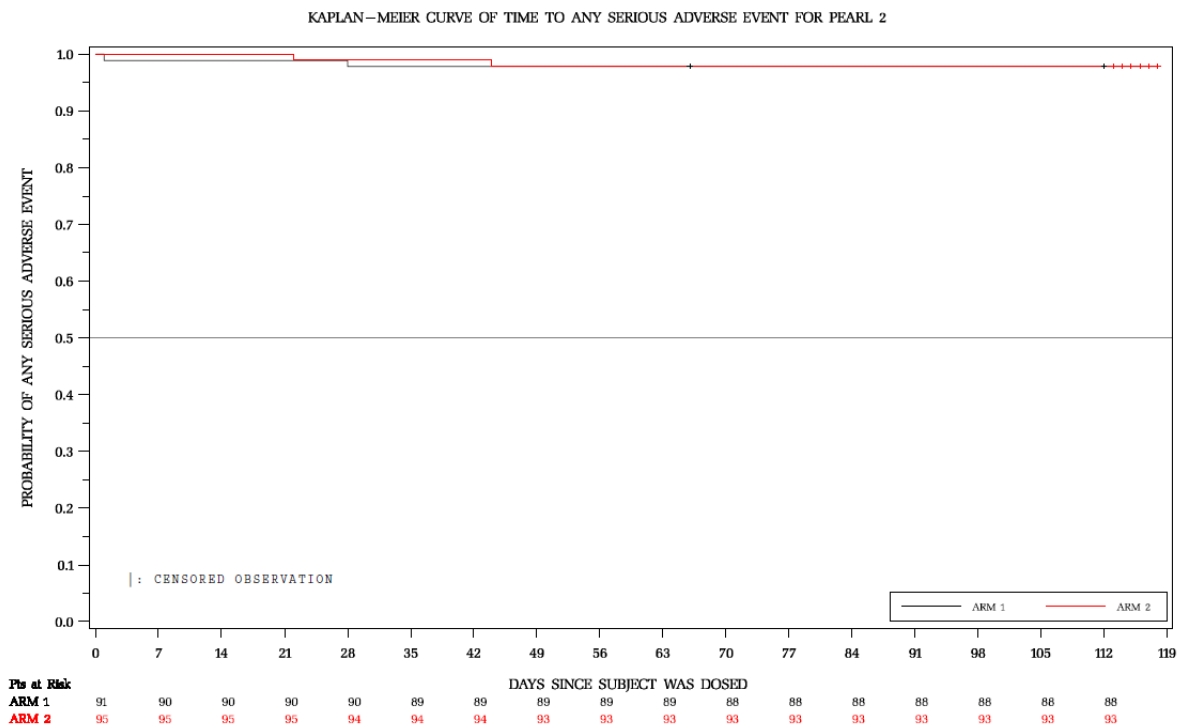
Abbildung 3: Kaplan-Meier-Kurve für die Gesamtrate an SUE bei therapieerfahrenen Patienten mit CHC-Genotyp 1b ohne Zirrhose aus der Studie PEARL-II (Arm 1: OBV/PTV/R + DSV + RBV; Arm 2: OBV/PTV/R + DSV)
