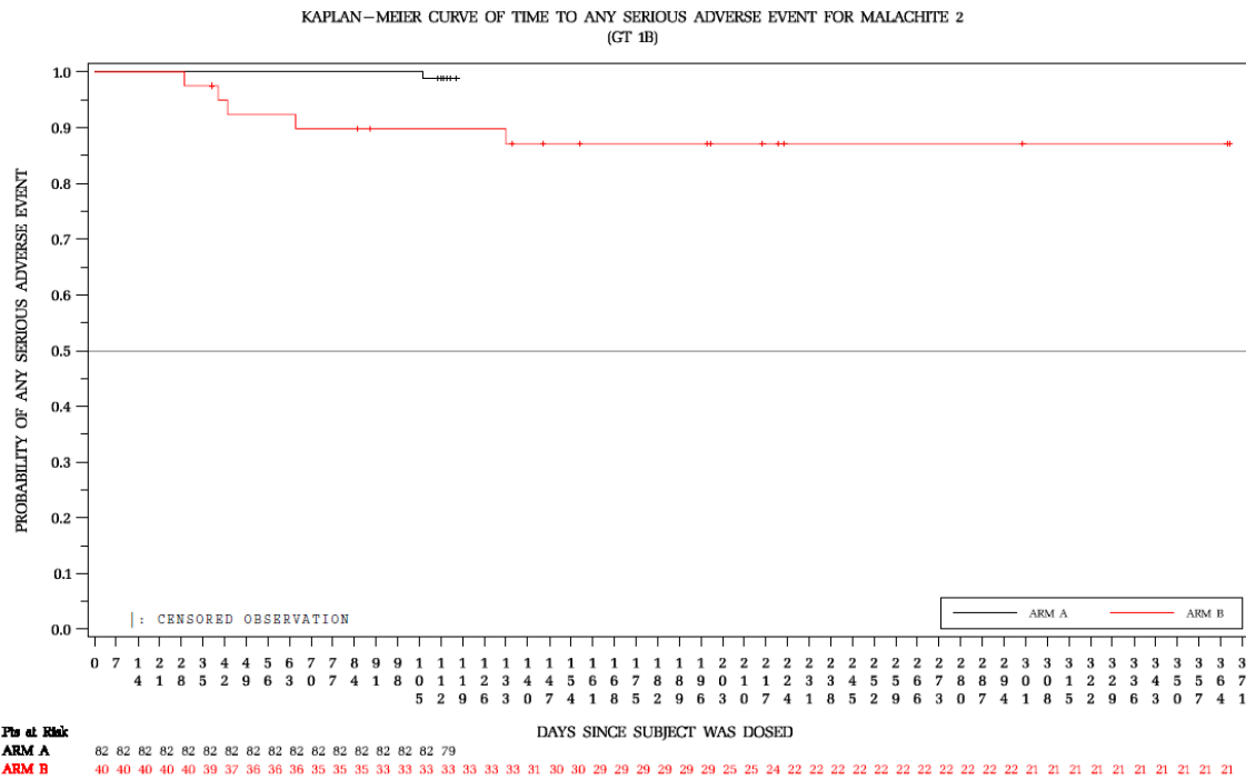
Abbildung 4: Kaplan-Meier-Kurve für die Gesamtrate an SUE bei therapieerfahrenen Patienten mit CHC-Genotyp 1b ohne Zirrhose aus der Studie MALACHITE-II (Arm A OBV/PTV/R + DSV; Arm B: TVR + PEG + RBV)
