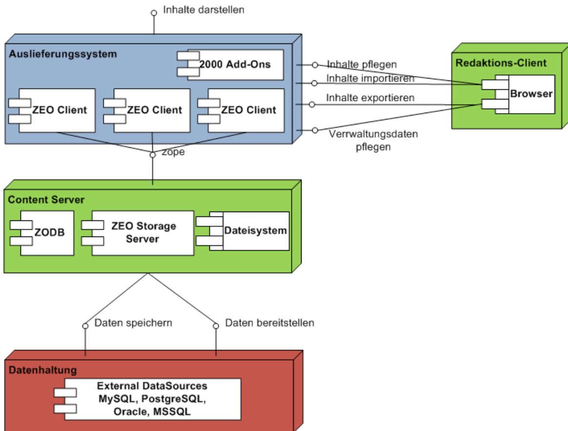
Abbildung 2.3: Plone – Systemarchitektur
