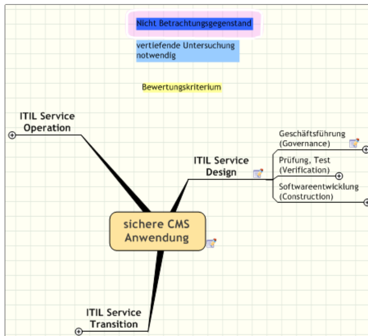
Abbildung 2.7: Kriterienüberblick
