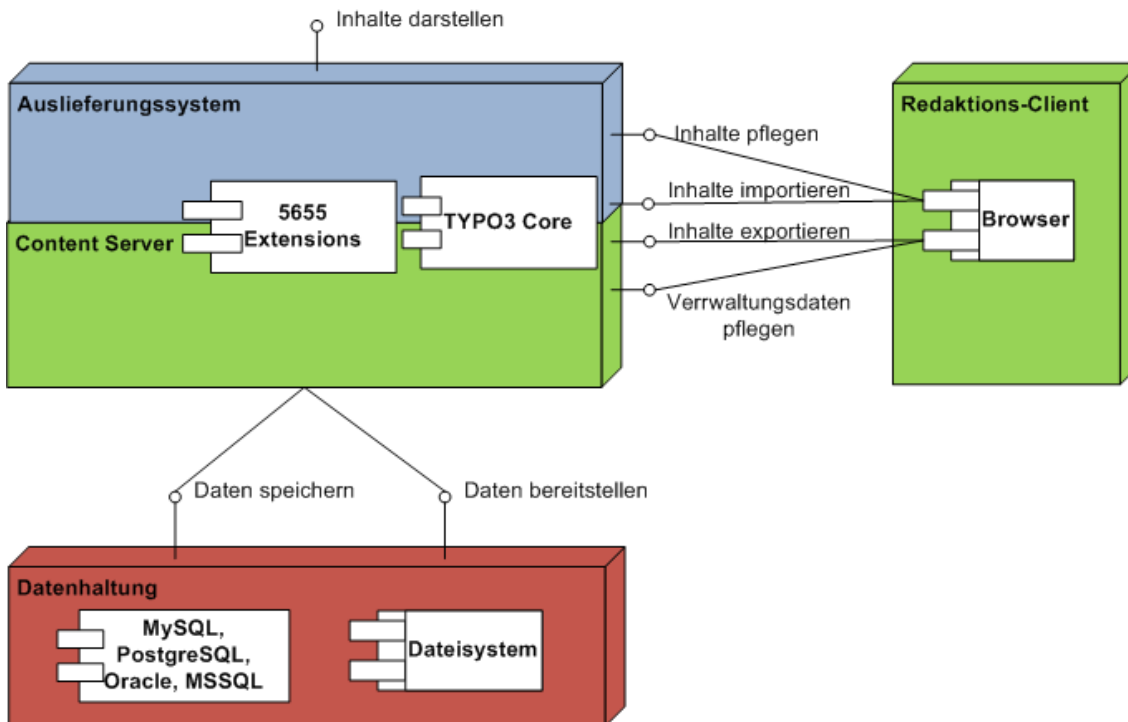
Abbildung 2.6: TYPO3 – Systemarchitektur
