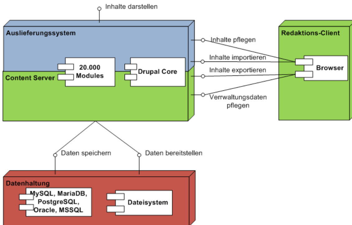
Abbildung 2.2: Drupal – Systemarchitektur
