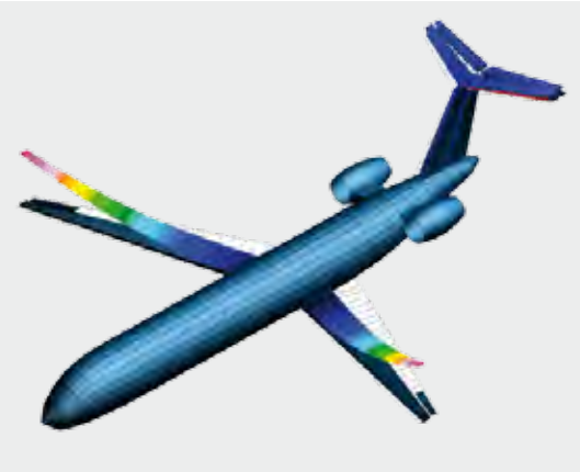
Aeroelastisches Modell zum Entwurf einer Konfiguration für 150 Passagiere mit vorwärtsgedrehten Tragflächen
