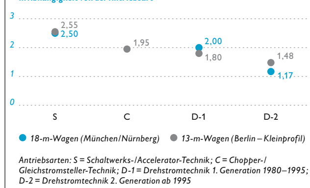
Entwicklung des Energieverbrauchs (in kWh/km und Wagen) in Abhängigkeit von der Antriebsart
