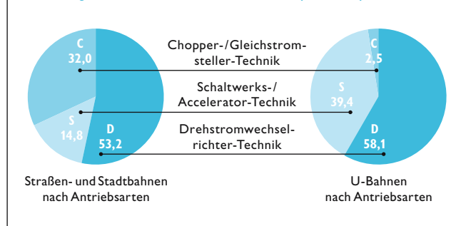
Verteilung der verschiedenen Antriebsarten 2008 (in Prozent)
