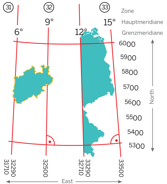
Abb. 8: Die Lage von Nordrhein-Westfalen in der UTM-Zone 32
