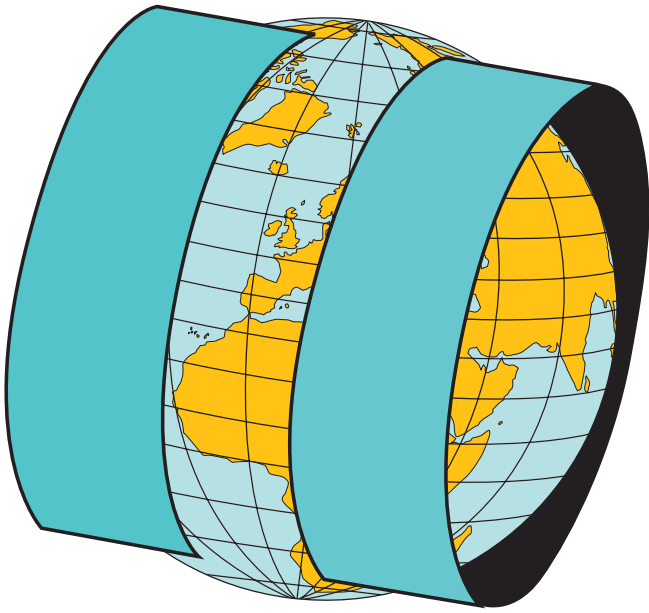
Abb. 7: Bildliche Darstellung der Lage des Schnitzzylinders bei UTM-Abbildung (Streifenbreite überhöht, sie beträgt lediglich 6°)
