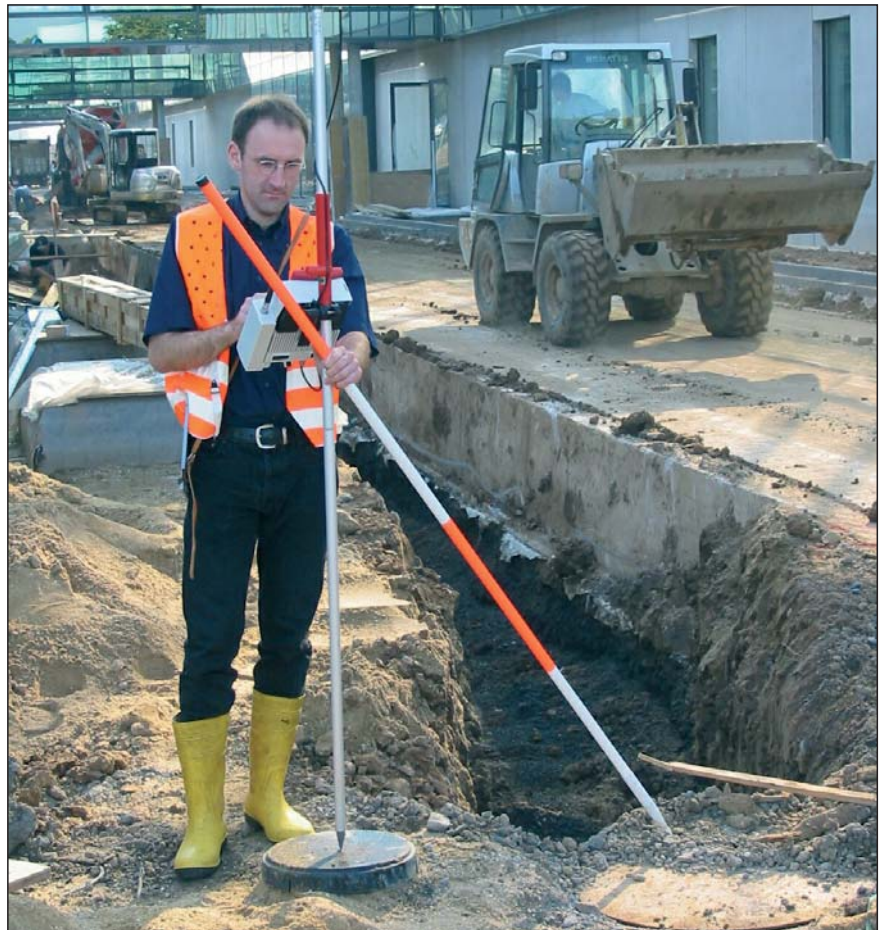
Abb. 3: GPS-Punktaufnahme im Gelände
