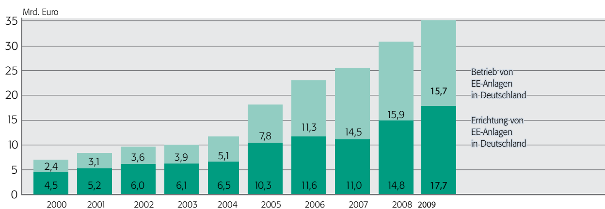
Abb. 2: Umsatz der deutschen Erneuerbaren-Energie-Branche 2000 - 2009
